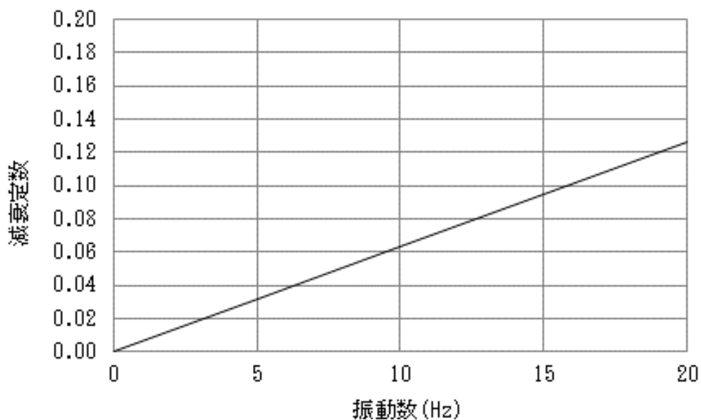
図 3-35 設定した Rayleigh 減衰
