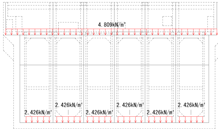
図3-36 機器・配管の荷重図（除じん機エリア）
