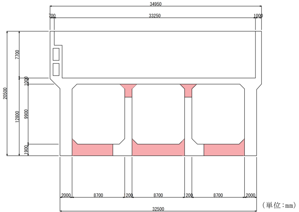
図 2-2 PHb 設置箇所 (B-B 断面)
