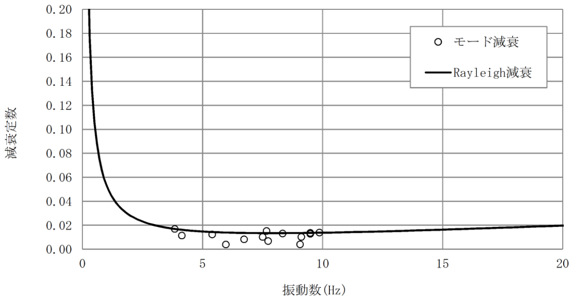
図 3-31 設定した Rayleigh 減衰 (A-A 断面)
