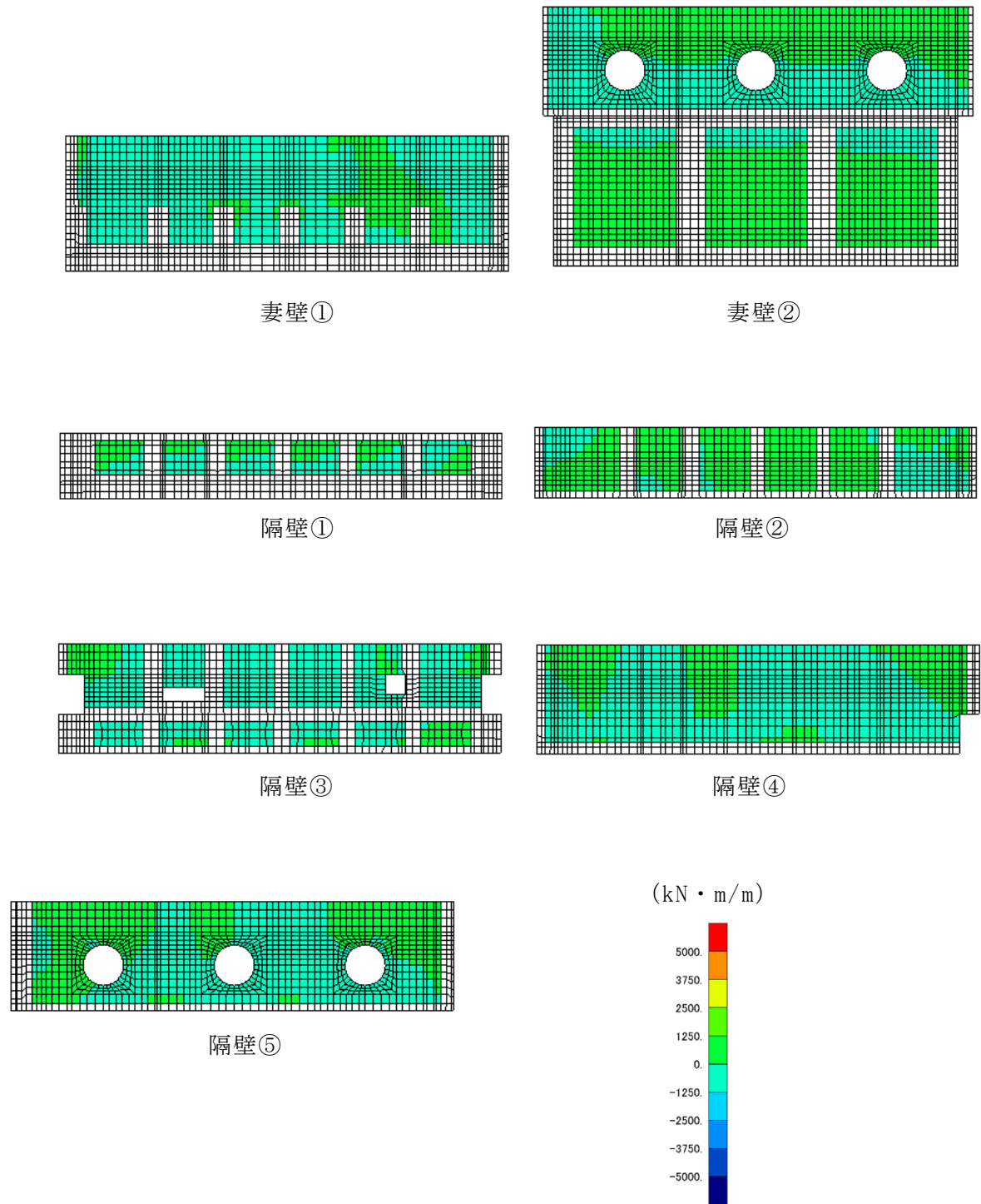
図 6-36 せん断破壊に対する照査値最大時の断面力分布図 (曲げモーメント ( \text{kN} \cdot \text{m} ) : M_y ) (側壁, 解析ケース②, S_s - D (-+) )
