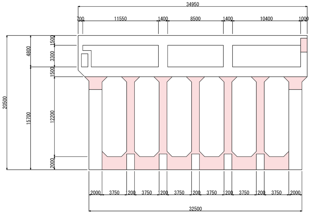
図 2-1 PHb 設置箇所 (A-A 断面) (単位:mm)
