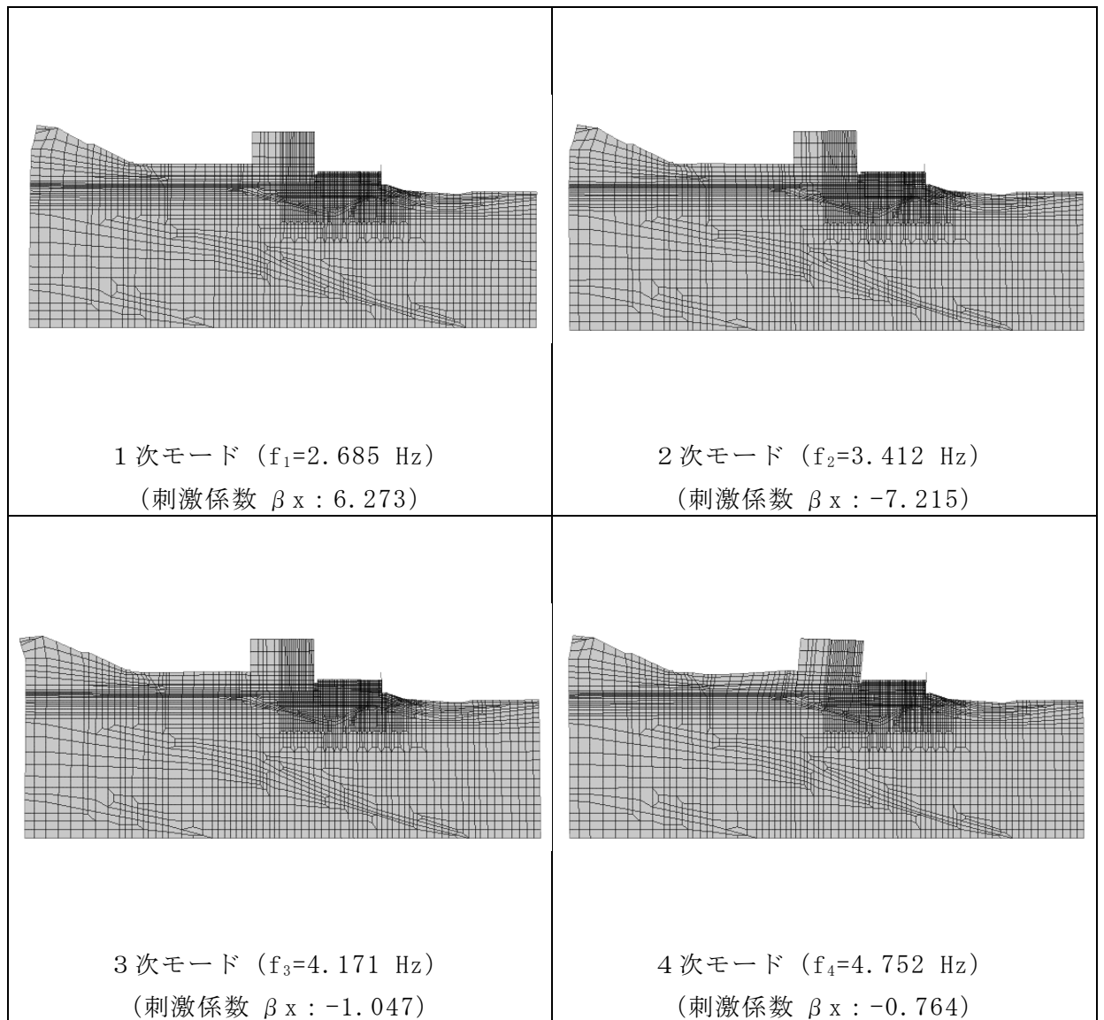
図 3-30 (1) 固有値解析結果 (モード図) (D-D断面)
