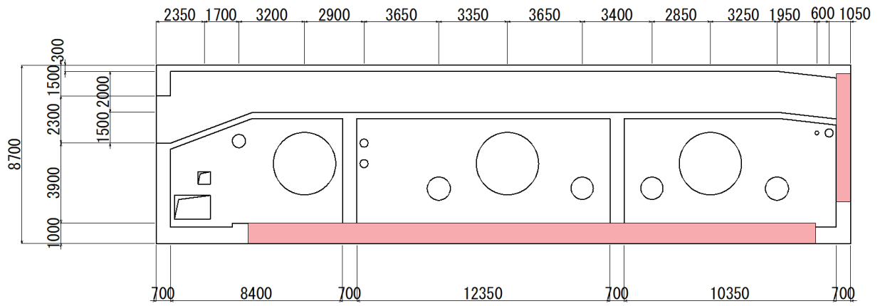
图 2-3 PHb 設置箇所 (C-C 断面) (単位:mm)
