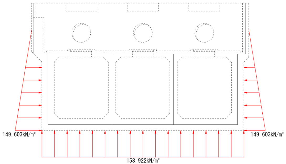
図3-50 外水圧図（海水ポンプエリア）
