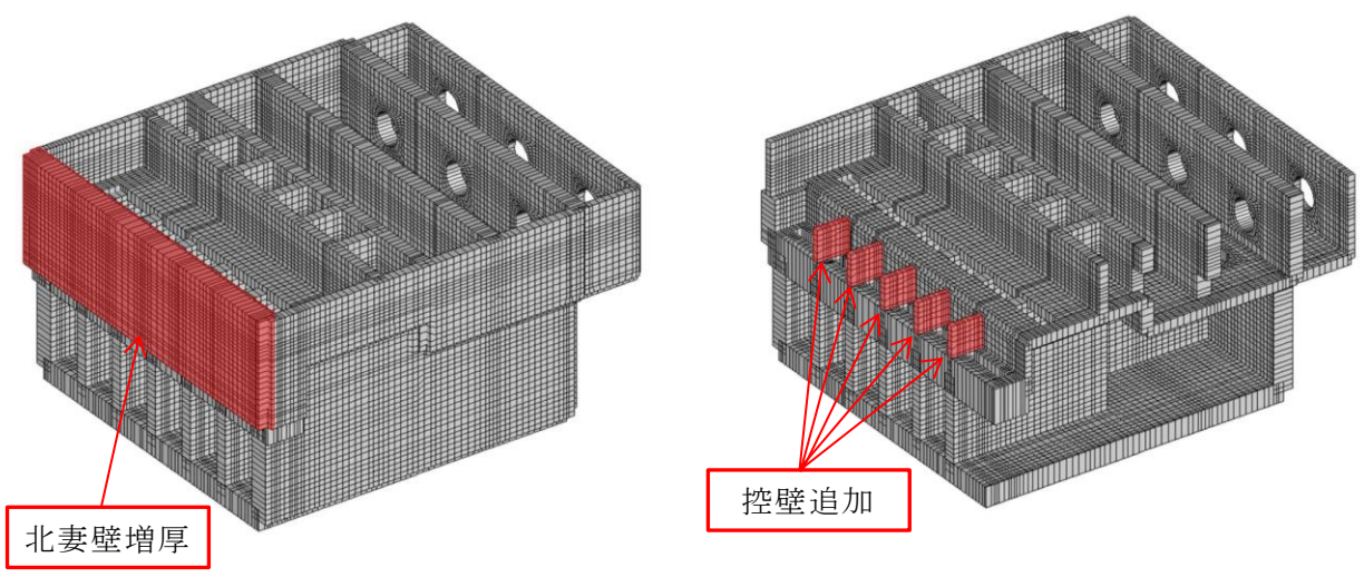
(鳥瞰図)
