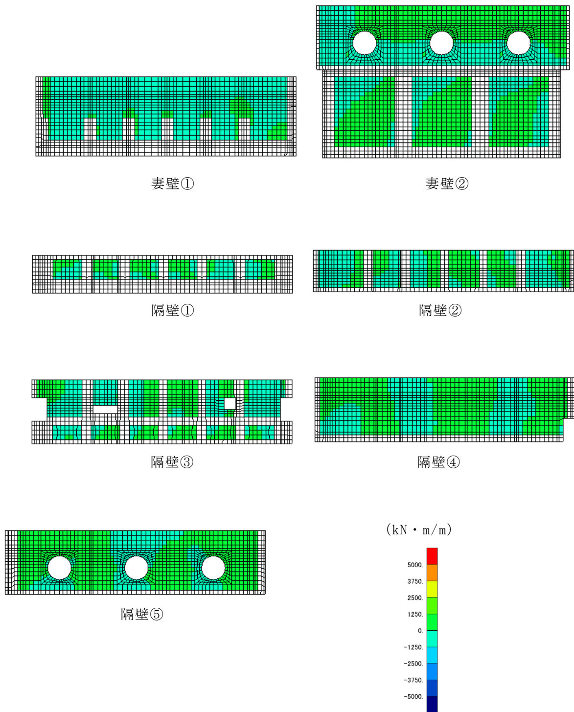
図 6-33 せん断破壊に対する照査値最大時の断面力分布図 (曲げモーメント (kN・m) : M_x ) (側壁, 解析ケース②, S_s - D (-+) )
