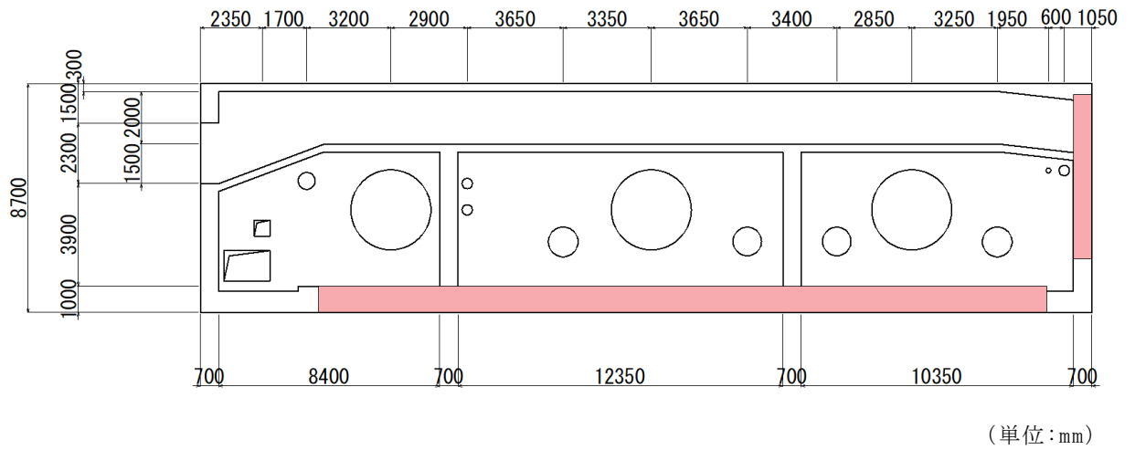
図 5-56 PHb による耐震補強箇所 (断面図 (C-C 断面)) (再掲)
