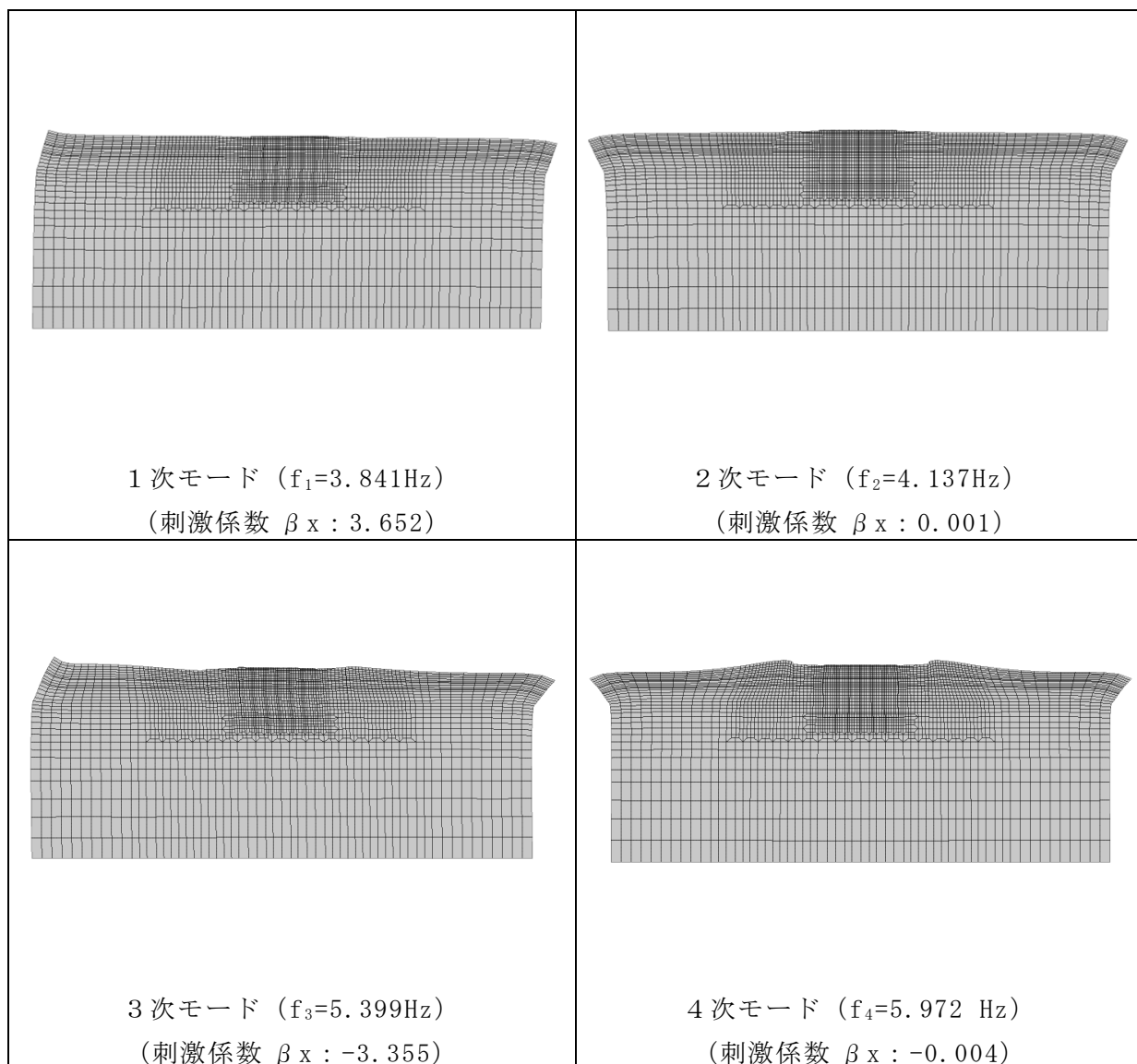
図 3-27 (1) 固有値解析結果 (モード図) (A-A断面)
