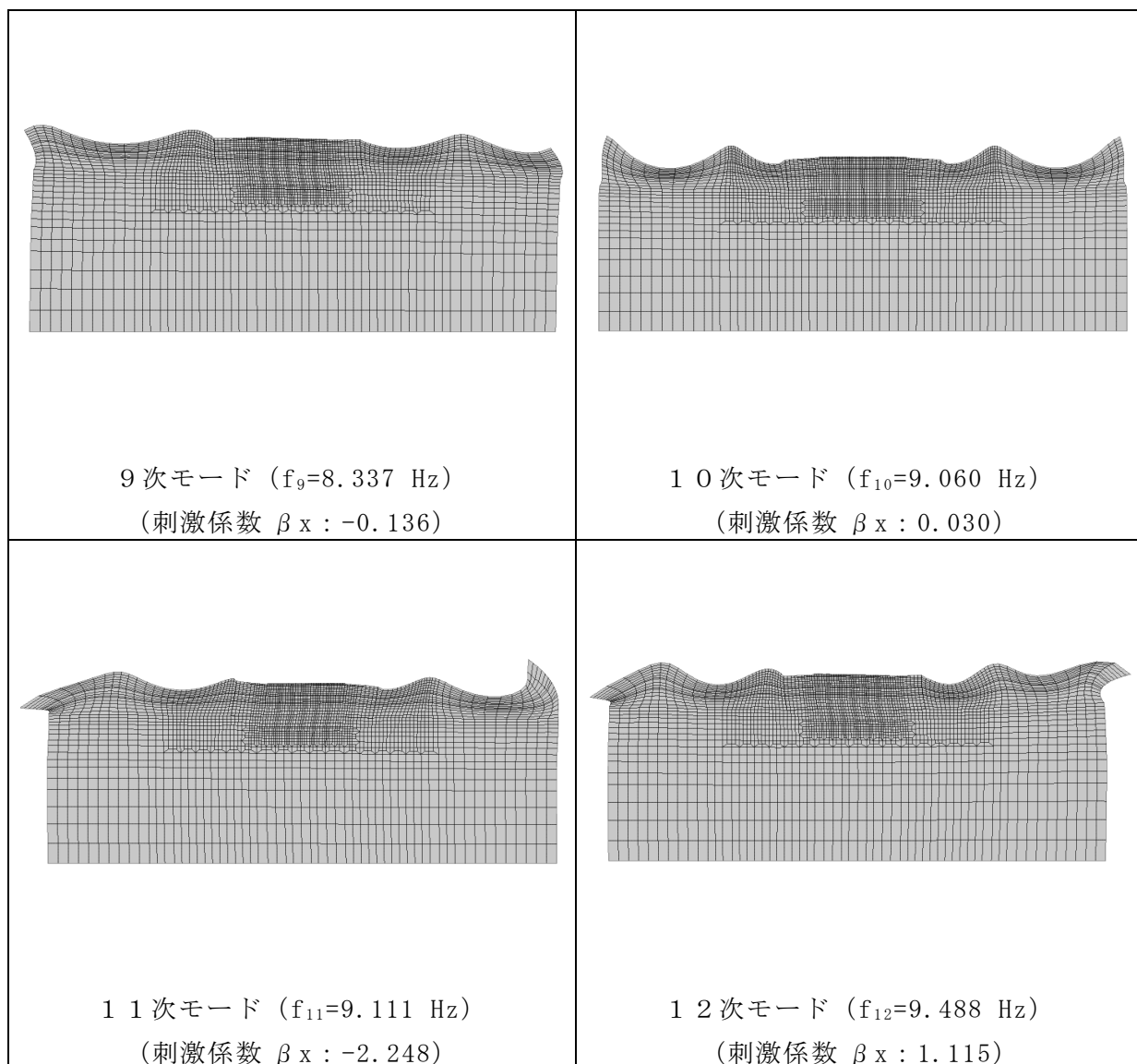
図 3-27 (3) 固有値解析結果 (モード図) (A-A断面)
