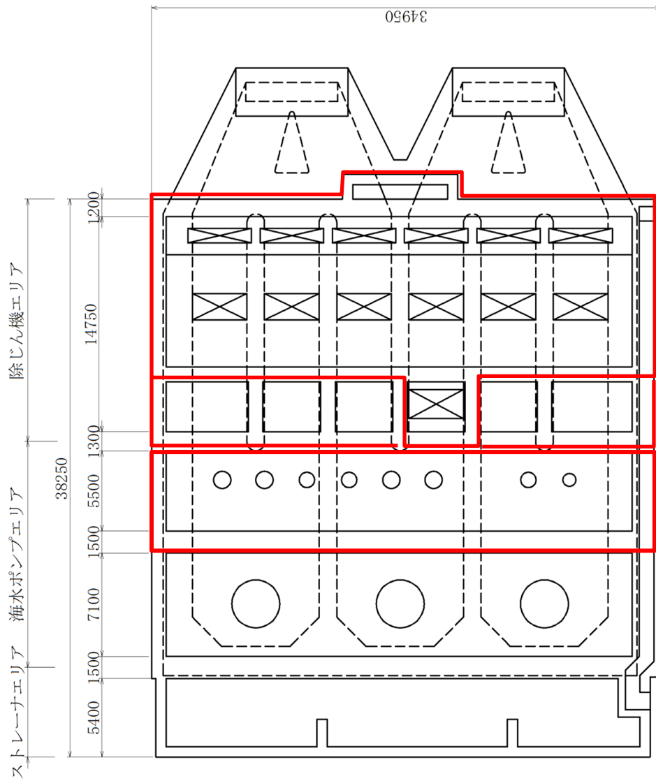
図3-40 浸水防護施設 位置図
