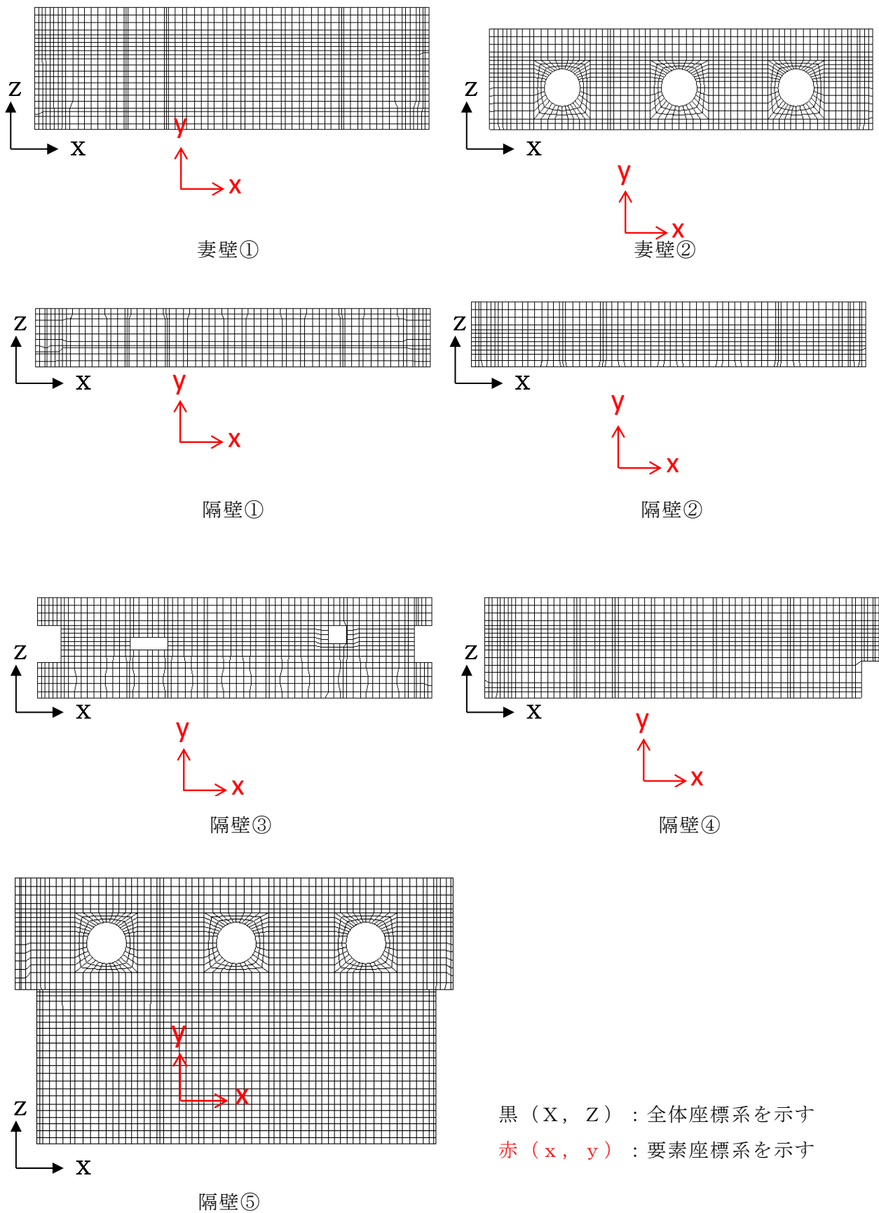
図 8-2 (3) 各部材の要素座標系
