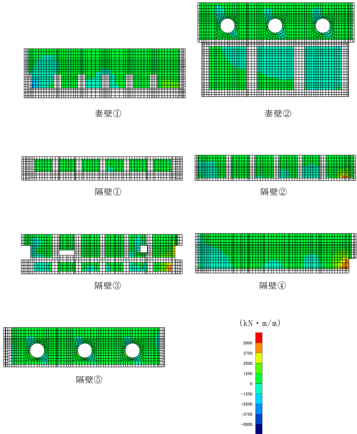
図 6-42 せん断破壊に対する照査値最大時の断面力分布図 (軸力 (kN/m) : N_y ) (側壁, 解析ケース②, S_s - D (-+) )
