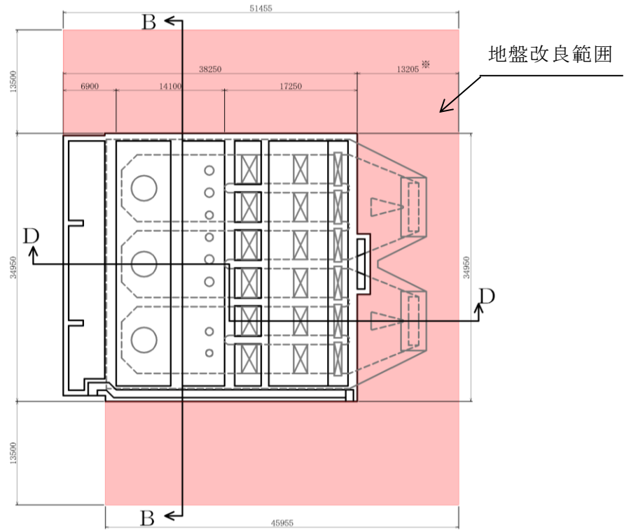
(平面図)
