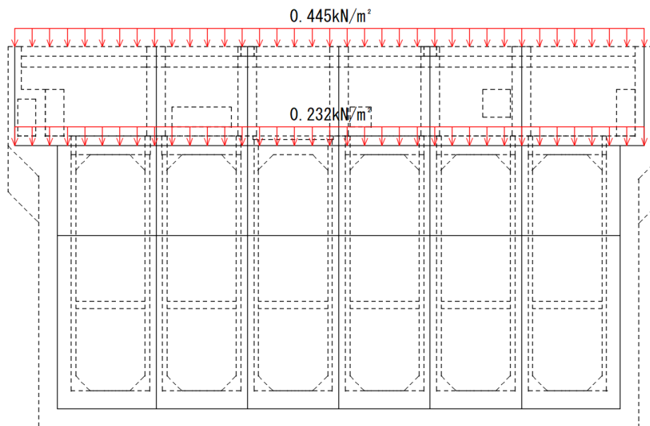
図 3-56 積雪荷重図（除じん機エリア）
