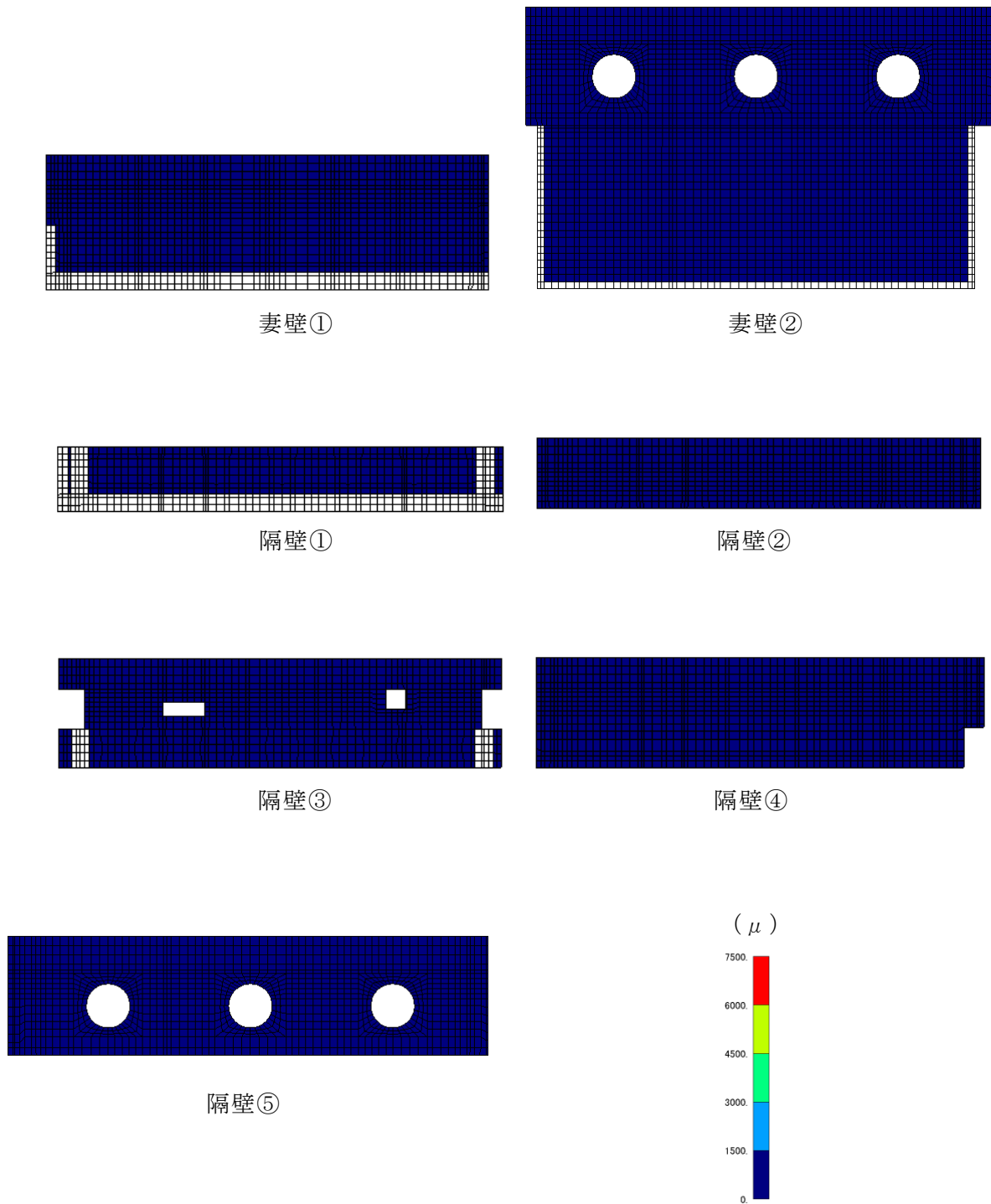
図 6-21 曲げ・軸力系の破壊に対する照査値最大時のひずみ分布図 (コンクリートの圧縮縁ひずみ) (側壁, 解析ケース④, S_s - D (-+) )
