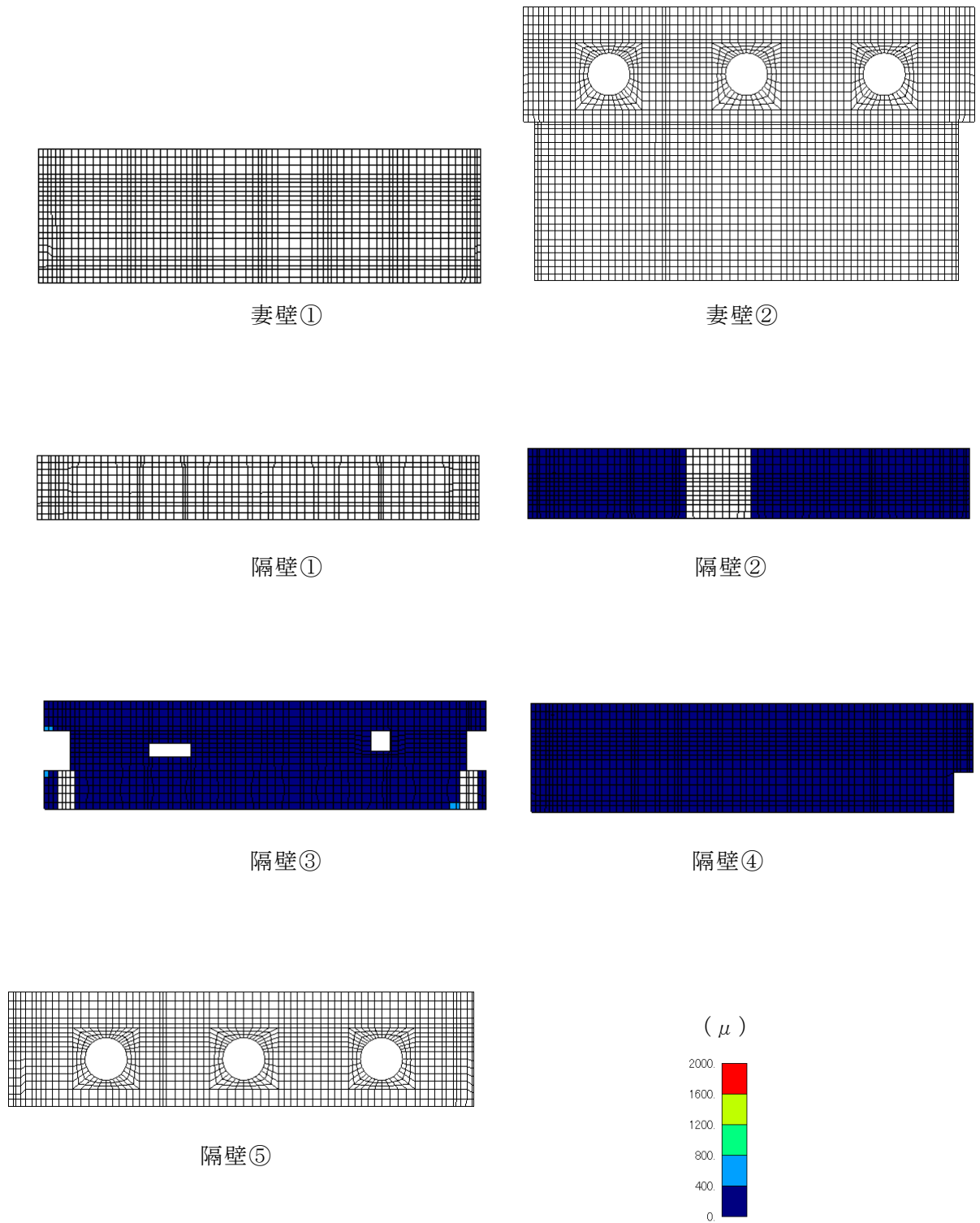
図 6-24 曲げ・軸力系の破壊に対する照査値最大時のひずみ分布図 (コンクリートの圧縮ひずみ) (側壁, 解析ケース④, S s - D (-+))
