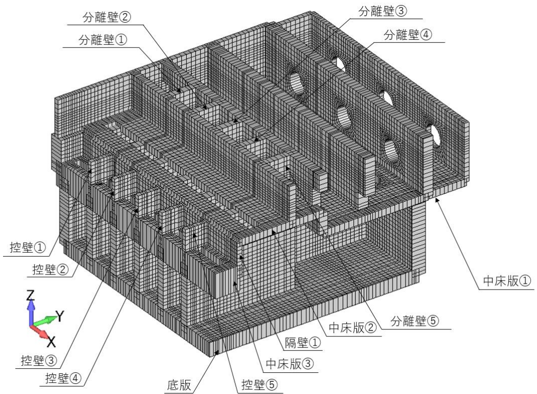
図 8-1 3次元解析モデル図*
