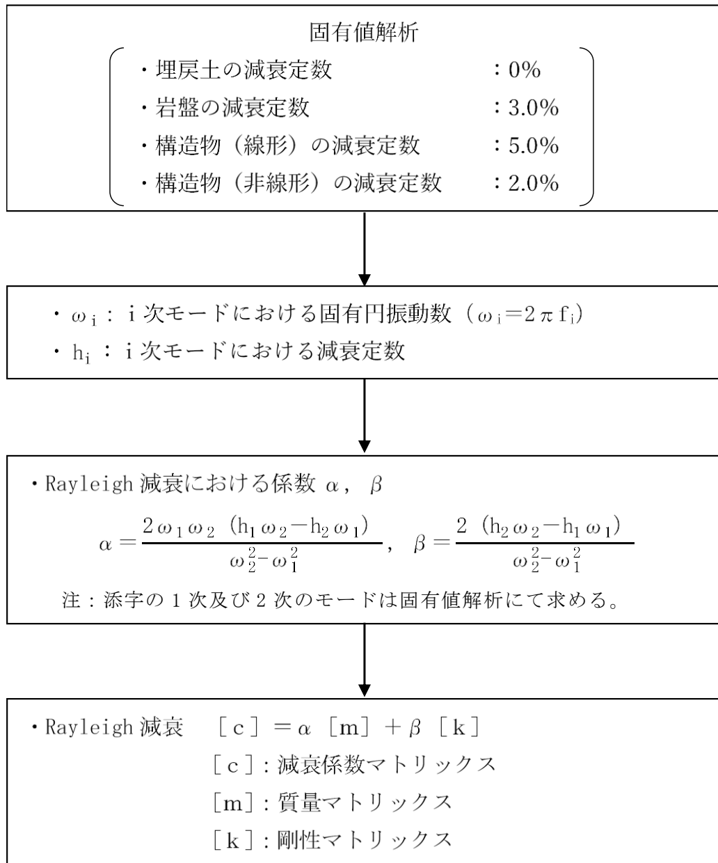
図 3-26 Rayleigh 減衰の設定フロー
