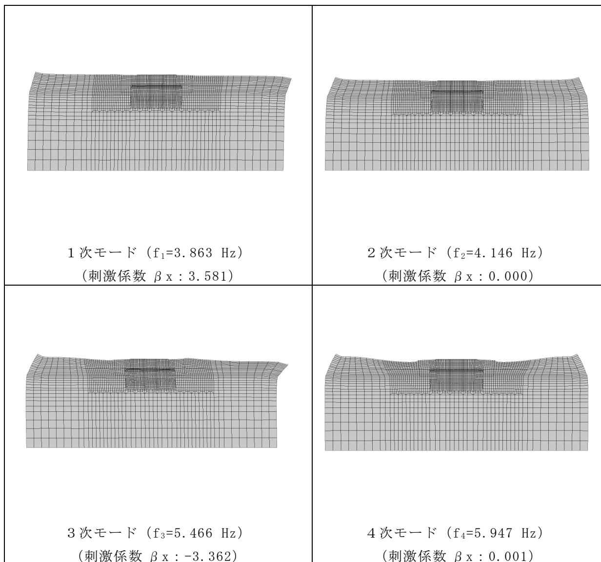
図 3-28 (1) 固有値解析結果 (モード図) (B-B 断面)
