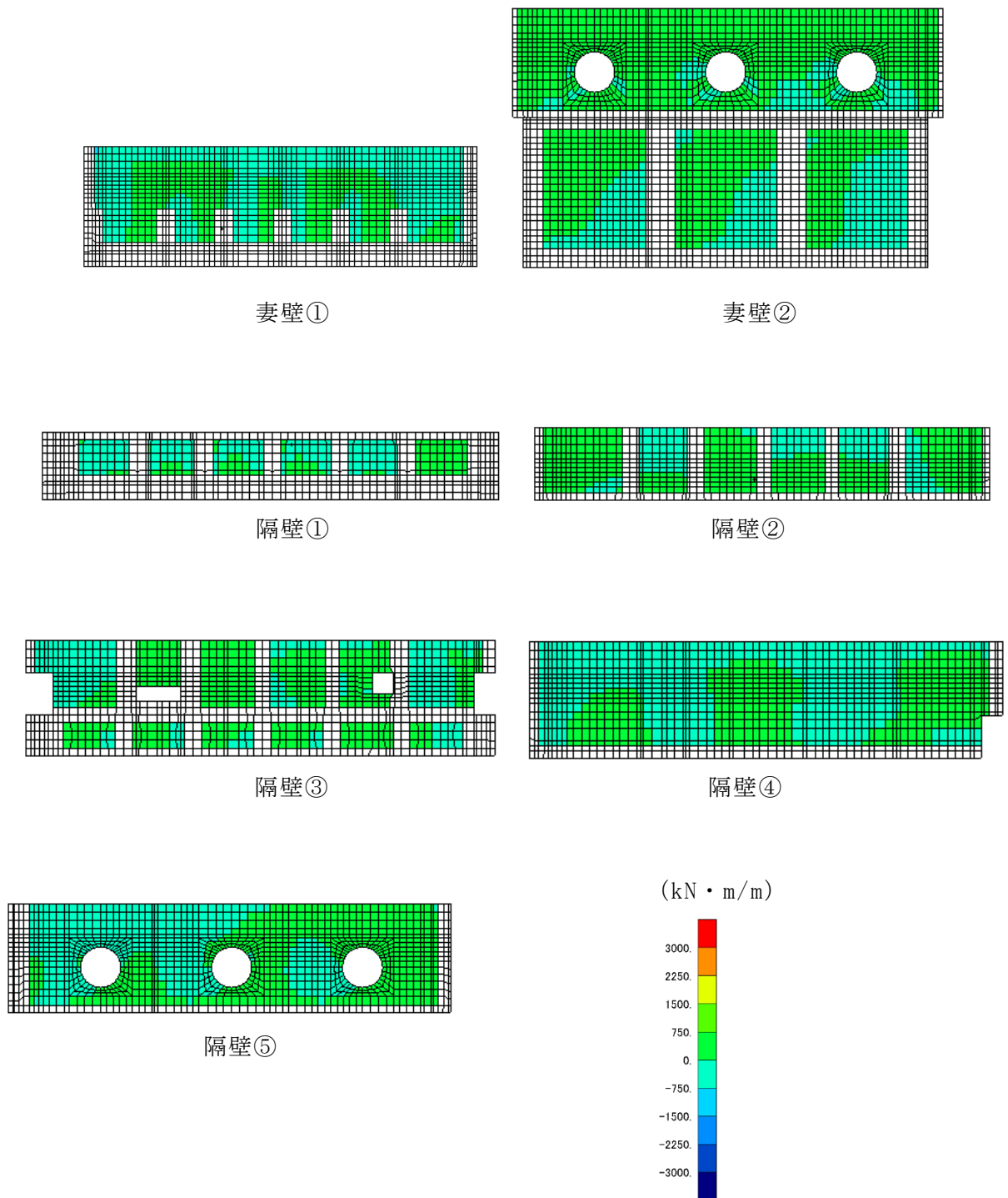
図 6-45 せん断破壊に対する照査値最大時の断面力分布図 (せん断力 (kN/m) : Q_x ) (側壁, 解析ケース②, S_s - D (-+) )
