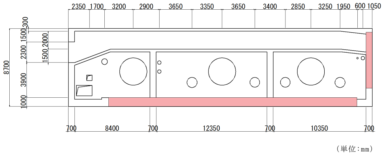
図 2-16 補強計画図 (断面図 (C-C 断面))
