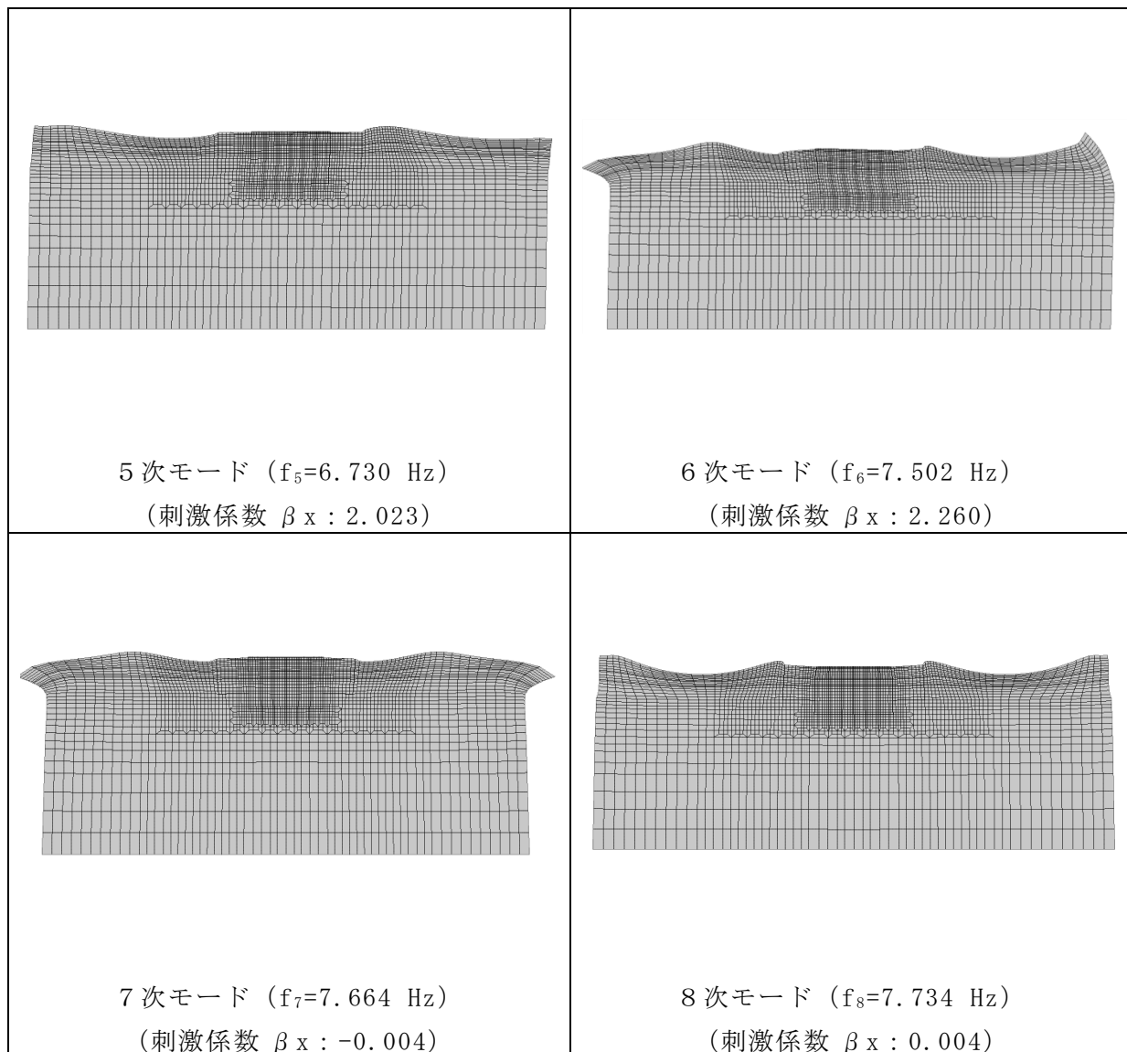
図 3-27 (2) 固有値解析結果 (モード図) (A-A断面)
