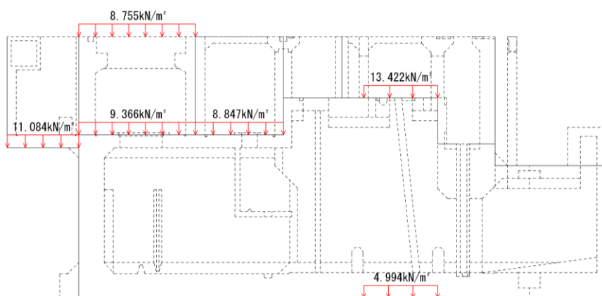
図 3-39 機器・配管の荷重図 (南北断面)
