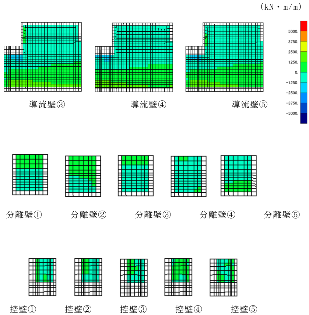
図 6-32 せん断破壊に対する照査値最大時の断面力分布図 (曲げモーメント (kN · m) : M_x ) (側壁, 解析ケース②, S_s - D (-+) )
