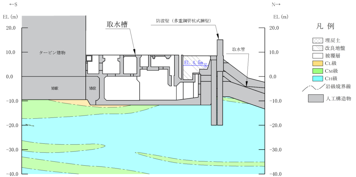
図5-65 地質断面図 (D-D断面)
