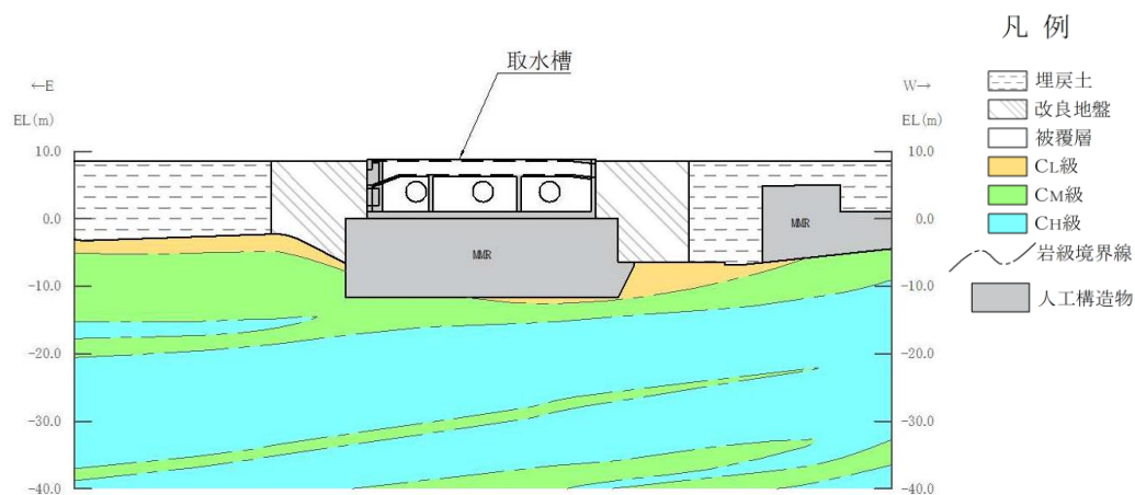
図 5-64 地質断面図 (C-C 断面)
