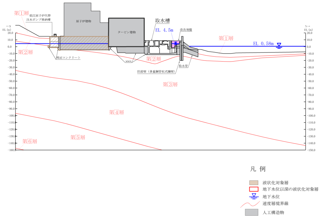
図 2-29 取水槽 地震時荷重算出断面図 (D-D 断面)
