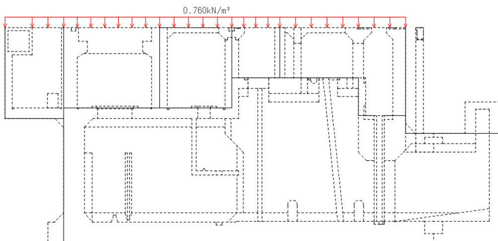
図 3-59 積雪荷重図 (南北断面)
