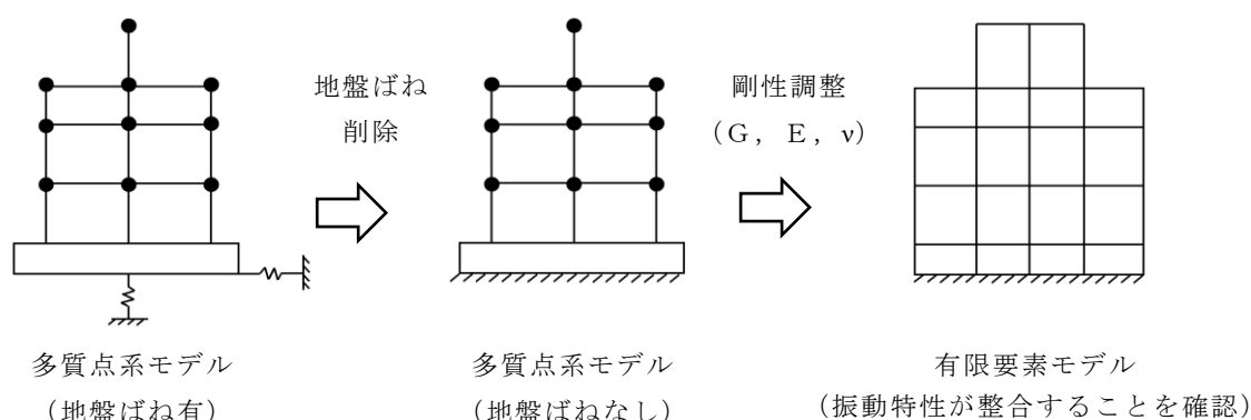
図3-18 タービン建物の有限要素モデル作成の考え方
