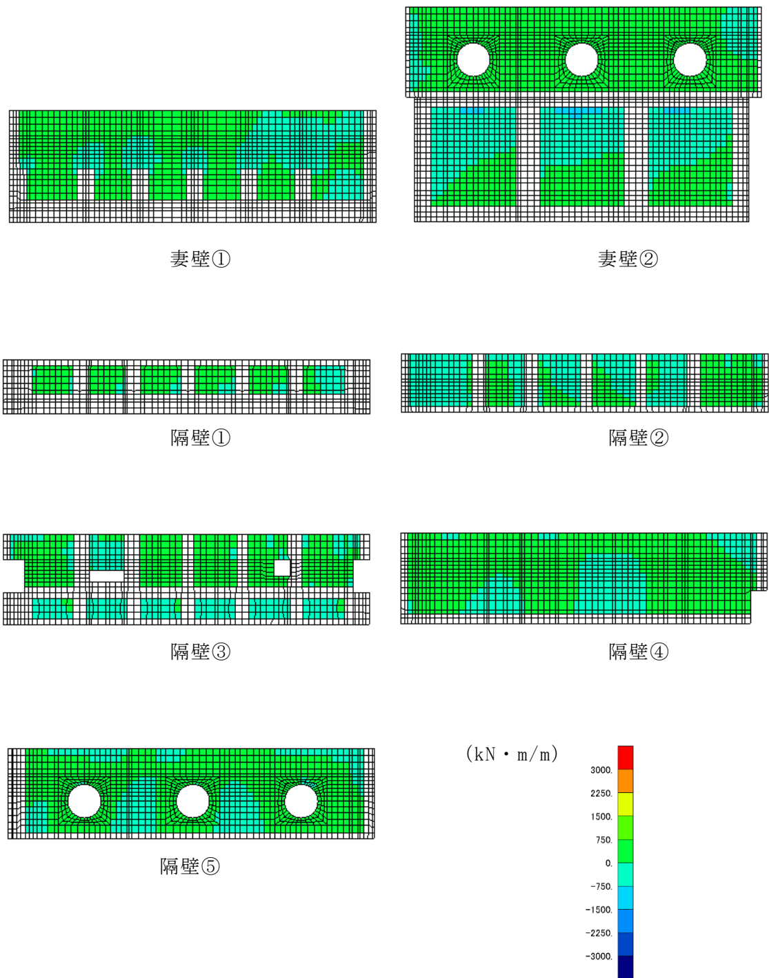
図 6-48 せん断破壊に対する照査値最大時の断面力分布図 (せん断力 (kN/m) : Q_y ) (側壁, 解析ケース②, S_s - D (-+) )
