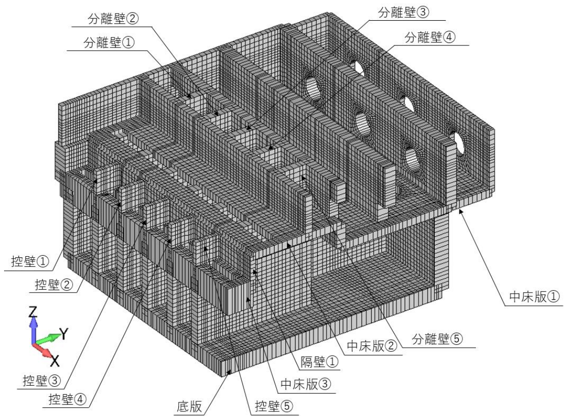
図 4-1 3次元構造解析モデルの概念図*
