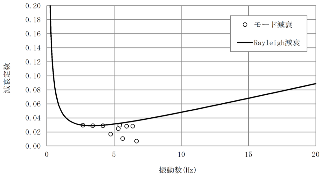
図 3-34 設定した Rayleigh 減衰 (D-D 断面)
