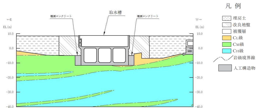
図5-63 地質断面図 (B-B断面)
