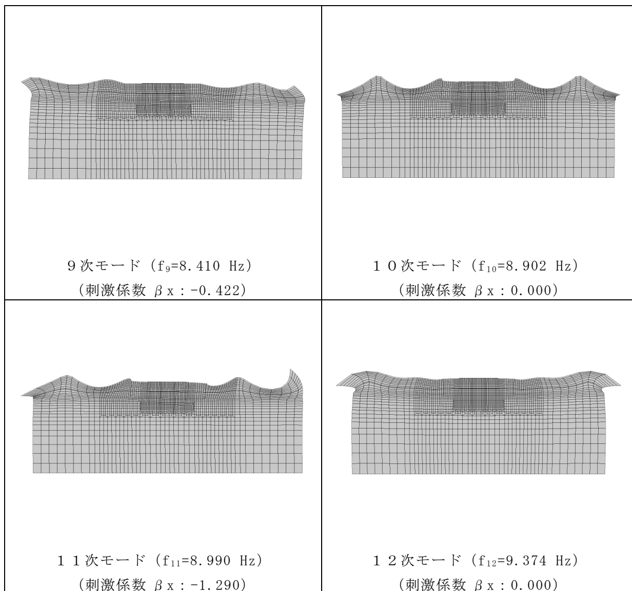
図 3-29 (3) 固有値解析結果 (モード図) (C-C断面)
