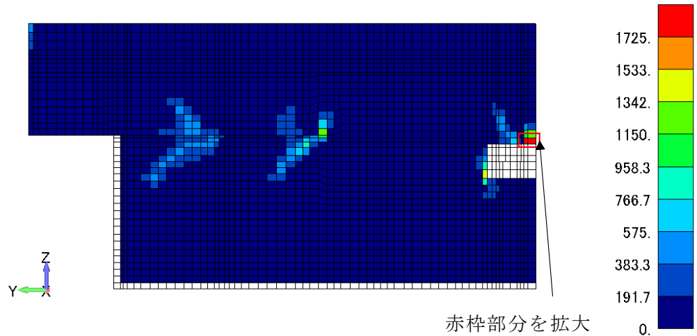
(a) 照査用主筋ひずみ分布全体図（側壁）
