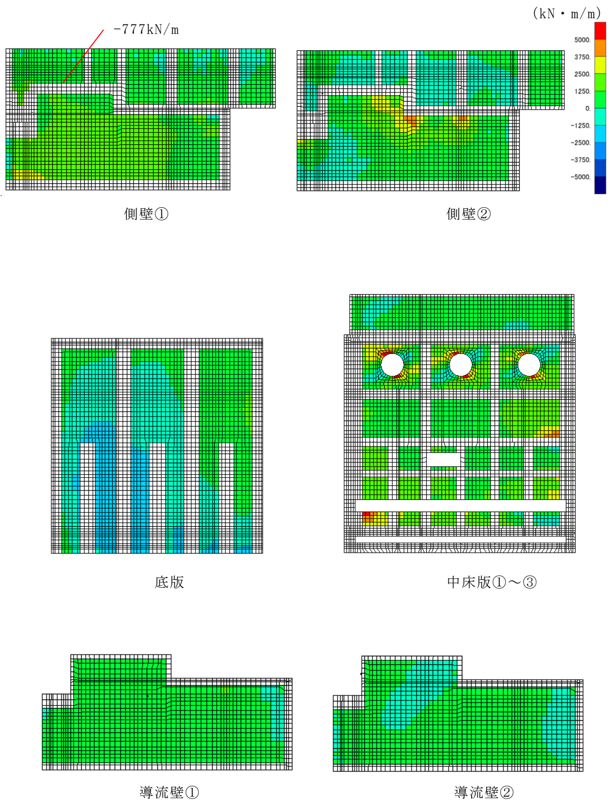
図 6-37 せん断破壊に対する照査値最大時の断面力分布図
