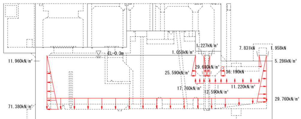
図 3-55 内水圧図（南北断面）
