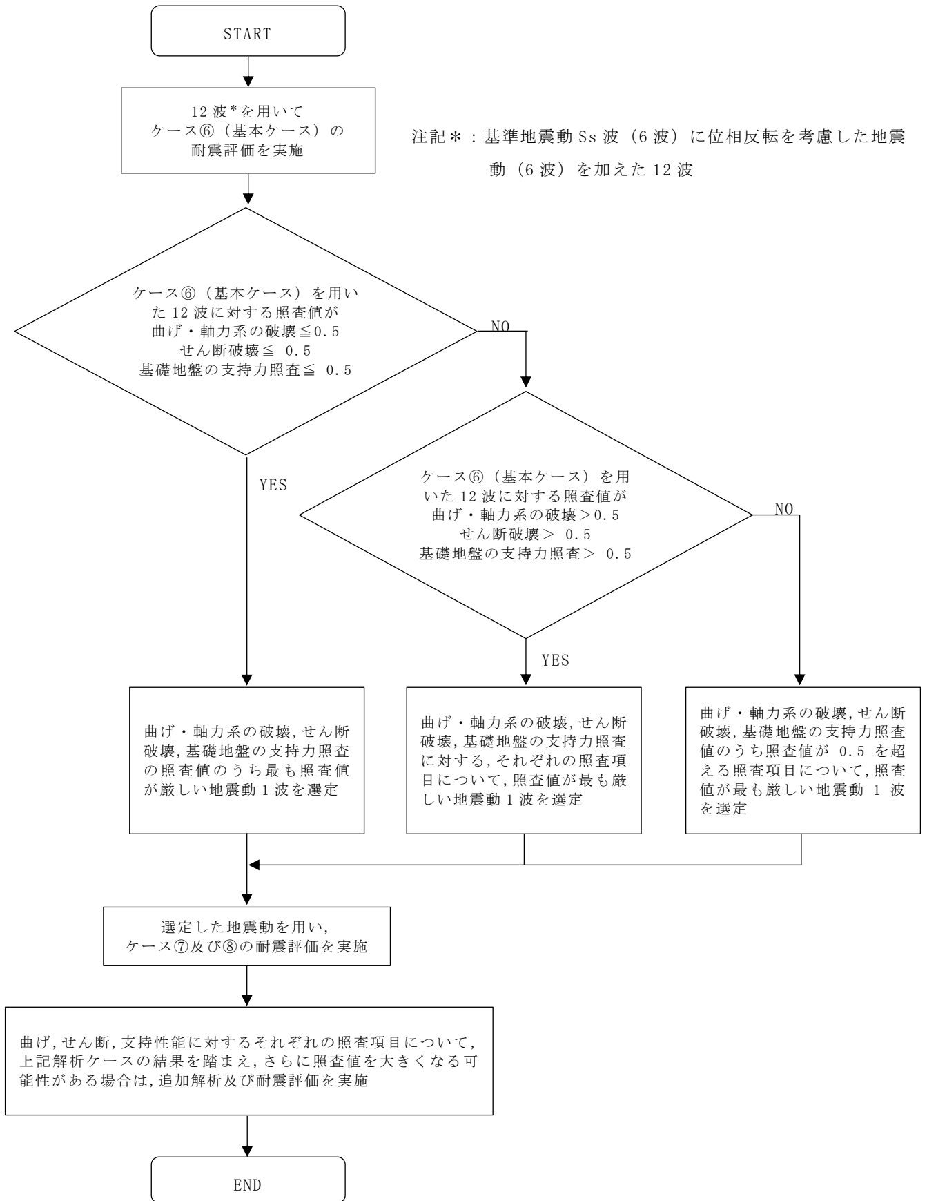
図 3-62 追加解析を実施する地震動の選定フロー (D-D 断面の例)
