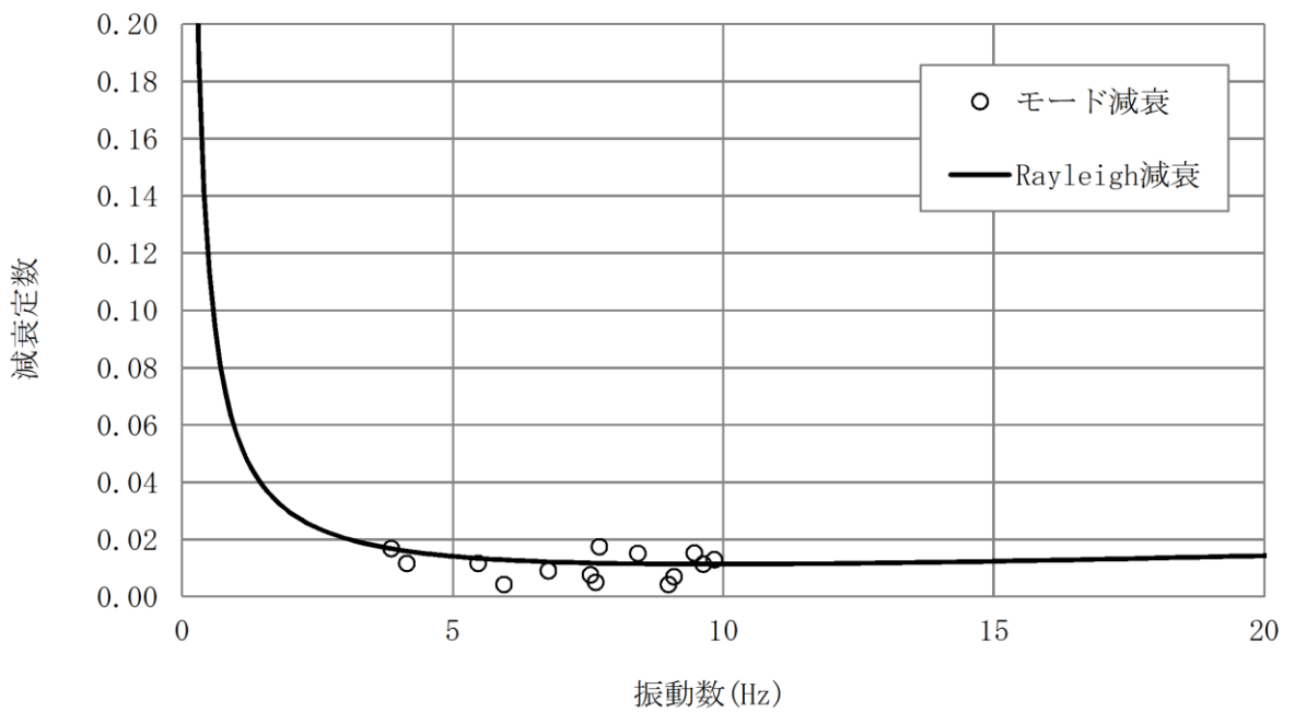
図 3-32 設定した Rayleigh 減衰 (B-B 断面)
