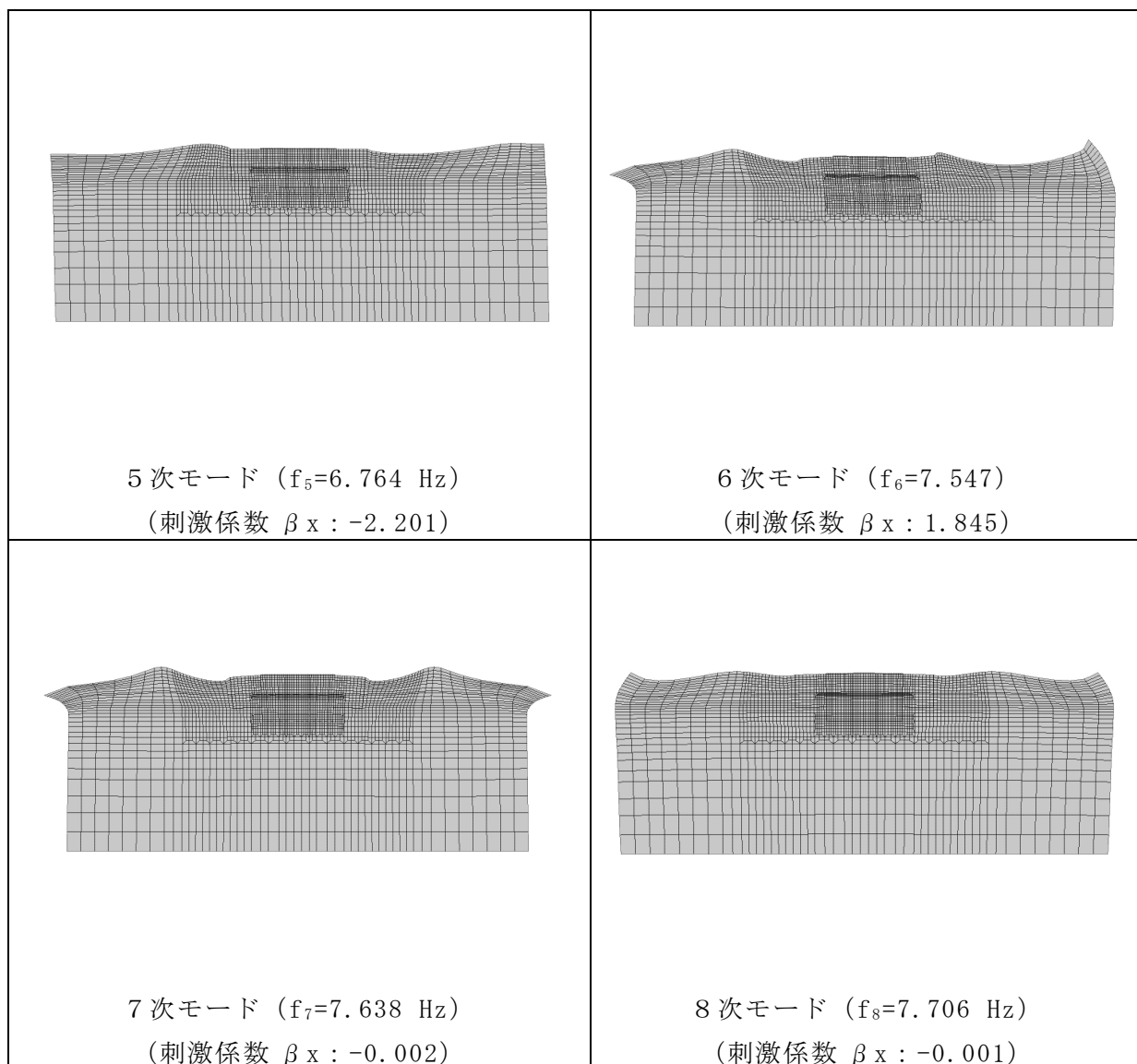
図 3-28 (2) 固有値解析結果 (モード図) (B-B断面)
