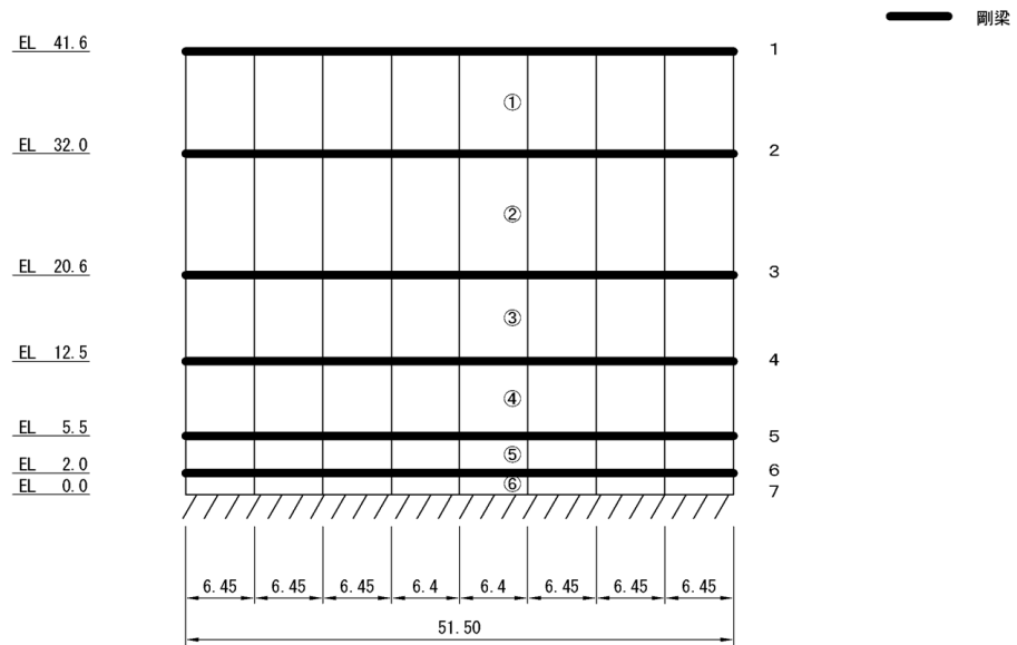
図 3-20 タービン建物 有限要素モデル図
