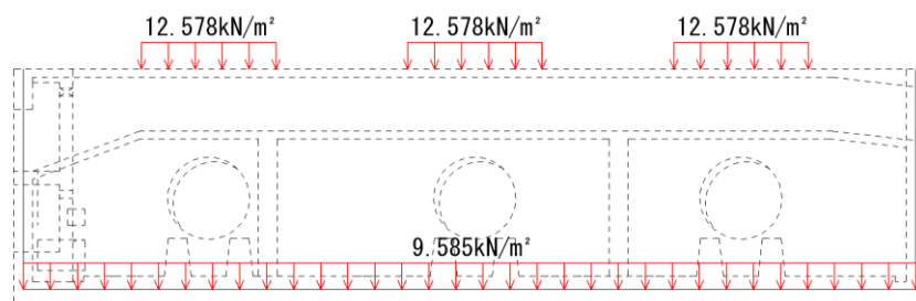
図 3-38 機器・配管の荷重図 (ストレーナエリア)
