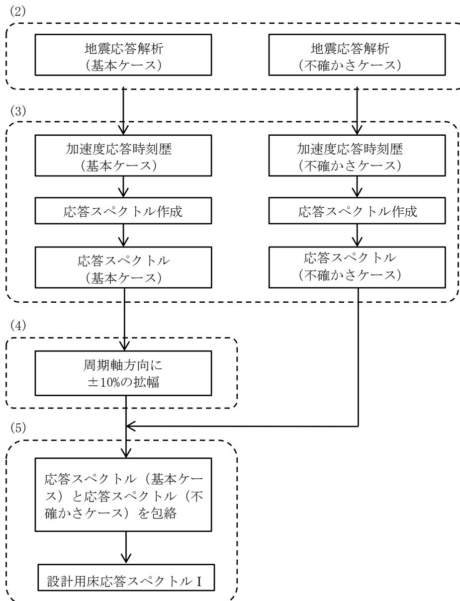
図 1 設計用床応答スペクトル I の作成方法の全体像
