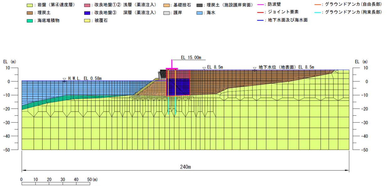
図 3-11 解析モデル (⑤-⑤断面)
