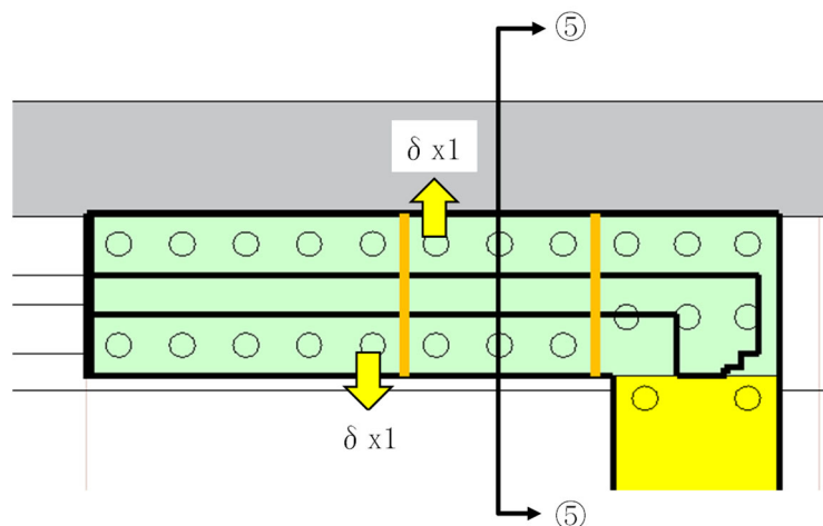
\delta_{z1} : ⑤-⑤断面の逆 T 擁壁天端における津波時の深度方向最大変位
