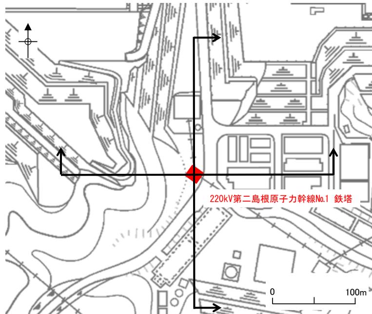
図1.1.10-8 平面図（220kV第二島根原子力幹線No.1鉄塔周辺）
