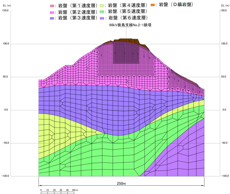
図1.2.10-12 地盤の地震応答解析モデル図(66kV 鹿島支線 No. 2-1 鉄塔)
