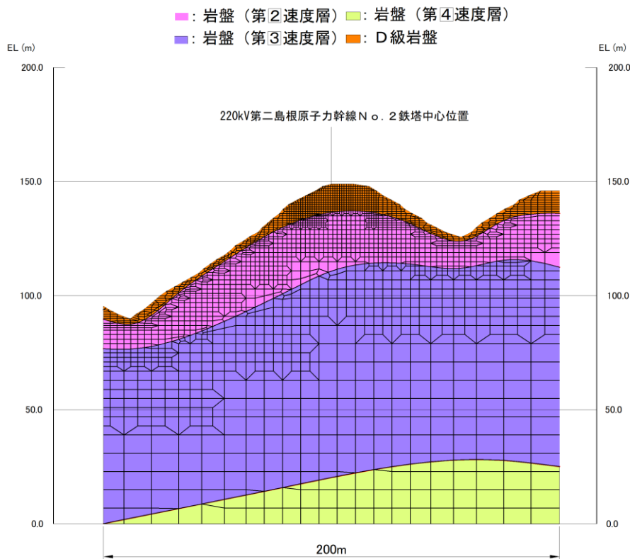
図 1. 1. 10-22 地盤の地震応答解析モデル図(220kV 第二島根原子力幹線 No. 2 鉄塔)
