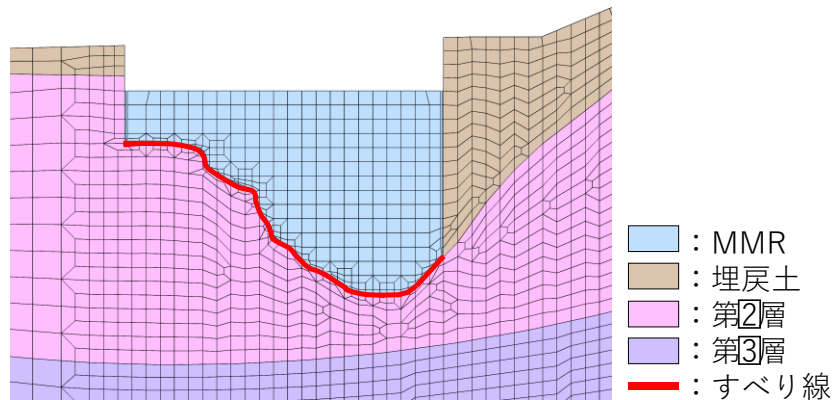
図 1.3.10-17 第2-66kV開閉所屋外鉄構におけるMMR-岩盤境界のすべり線の設定
