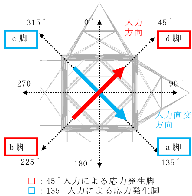
図 1.3.6-5 入力方向と支柱材発生応力の関係
