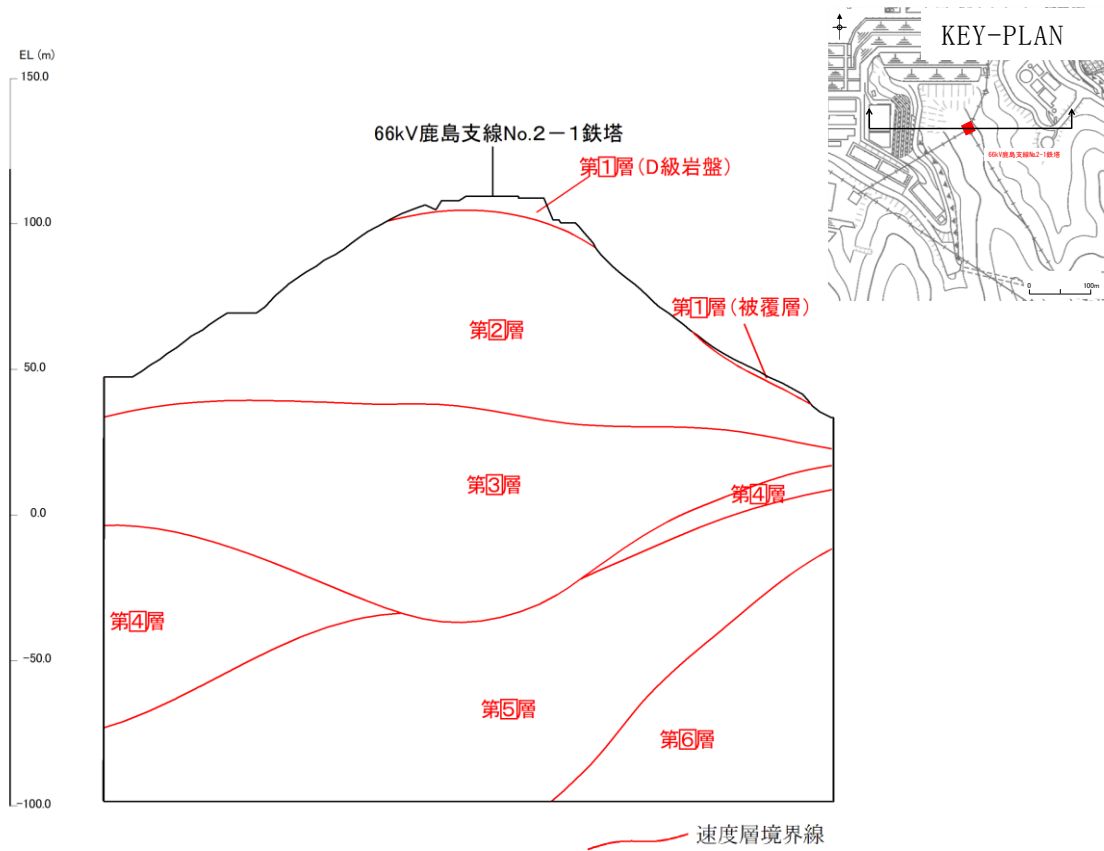
図1.2.10-11 地質断面図(66kV鹿島支線No.2-1鉄塔)
