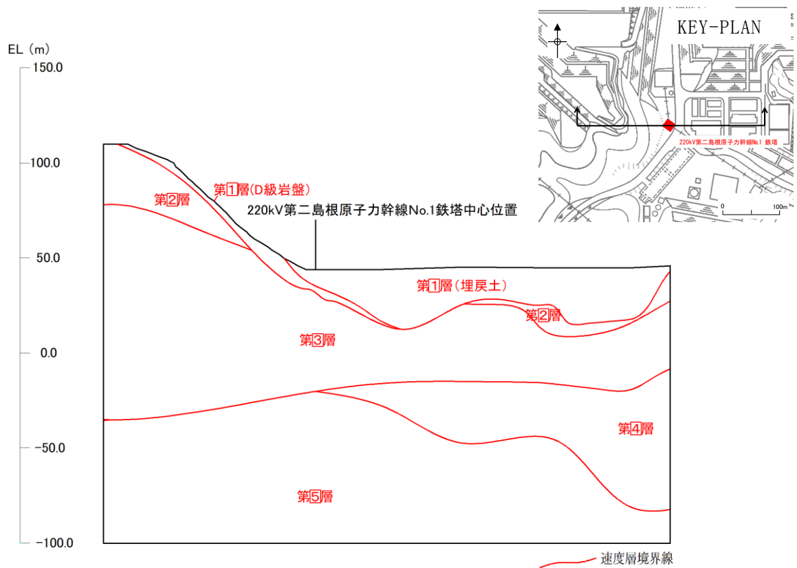
图 1.1.10-9 220kV 第二島根原子力幹線 No.1 鉄塔 地質断面図(速度層区分)
