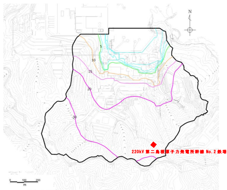
図1. 1. 10-18 敷地の地下水位分布（1, 2号機エリア）と220kV第二島根原子力発電所幹線No. 1鉄塔の位置関係
