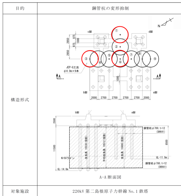
図 1.1.10-15 220kV 第二島根原子力発電所幹線 No. 1 鉄塔における地盤改良
