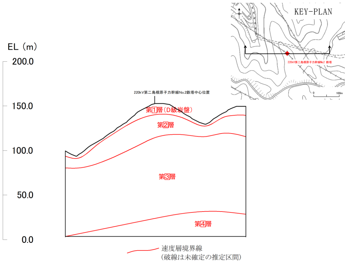
図 1. 1. 10-21 地質断面図(220kV 第二島根原子力幹線 No. 2 鉄塔)
