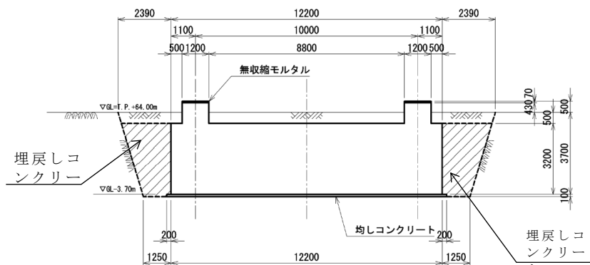
(b) 正面図
