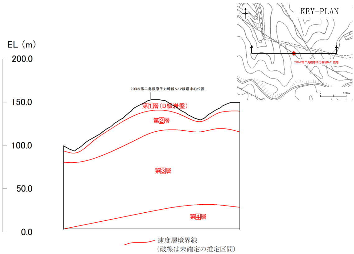
図1.1.10-20 220kV第二島根原子力発電所幹線No.2鉄塔 地質断面図(速度層区分)
