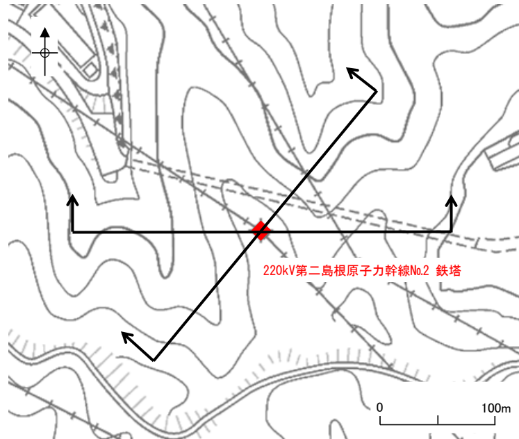
図1.1.10-19 220kV第二島根原子力発電所幹線No.2鉄塔の南北方向及び東西方向の平面位置図
