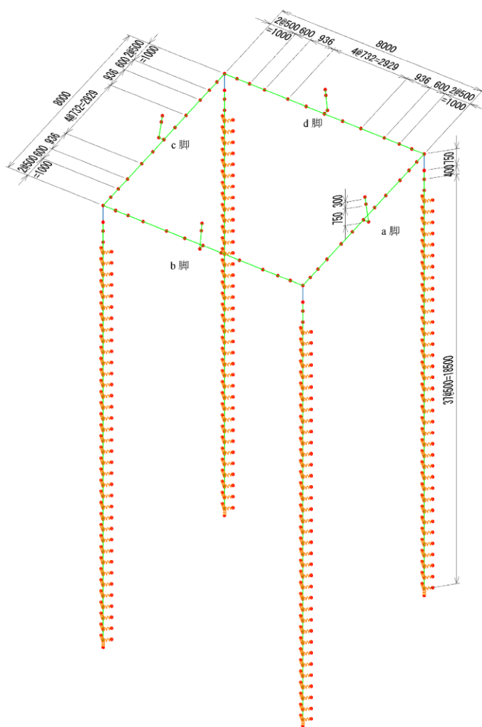
図 1.2.10-14 66kV 鹿島支線 No.2-1 鉄塔基礎解析モデル
