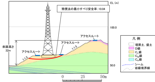
C-C' 断面
