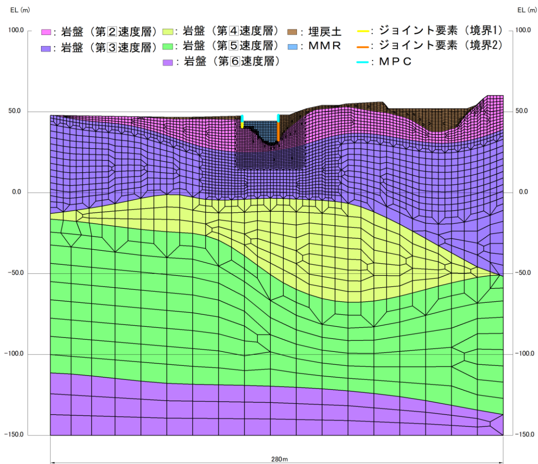
図1.3.10-13 地盤の地震応答解析モデル図(第2-66kV開閉所屋外鉄構)
