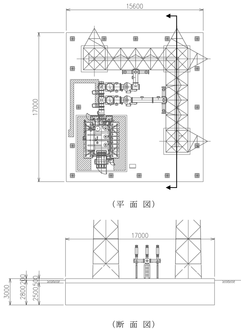
図 1.3.10-18 第2-66kV開閉所屋外鉄構基礎構造図
