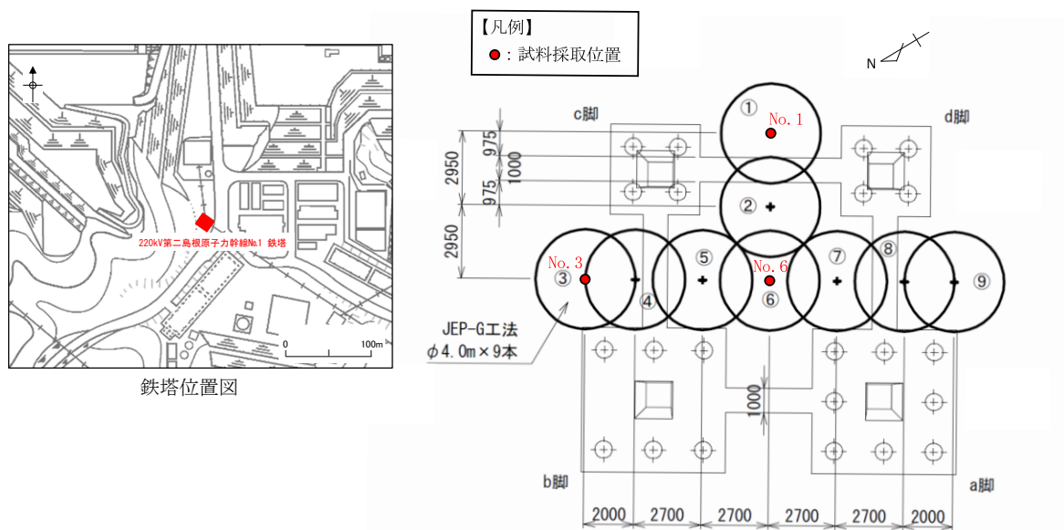
図1.1.10-14 当該改良地盤のコア資料採取位置図
