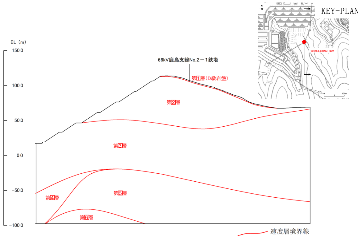
図1.2.10-9 地質断面図(66kV鹿島支線No.2-1鉄塔)
