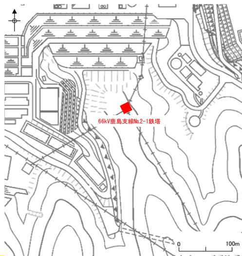
図1. 2. 10-5 66kV鹿島支線No. 2-1鉄塔周辺の地形
