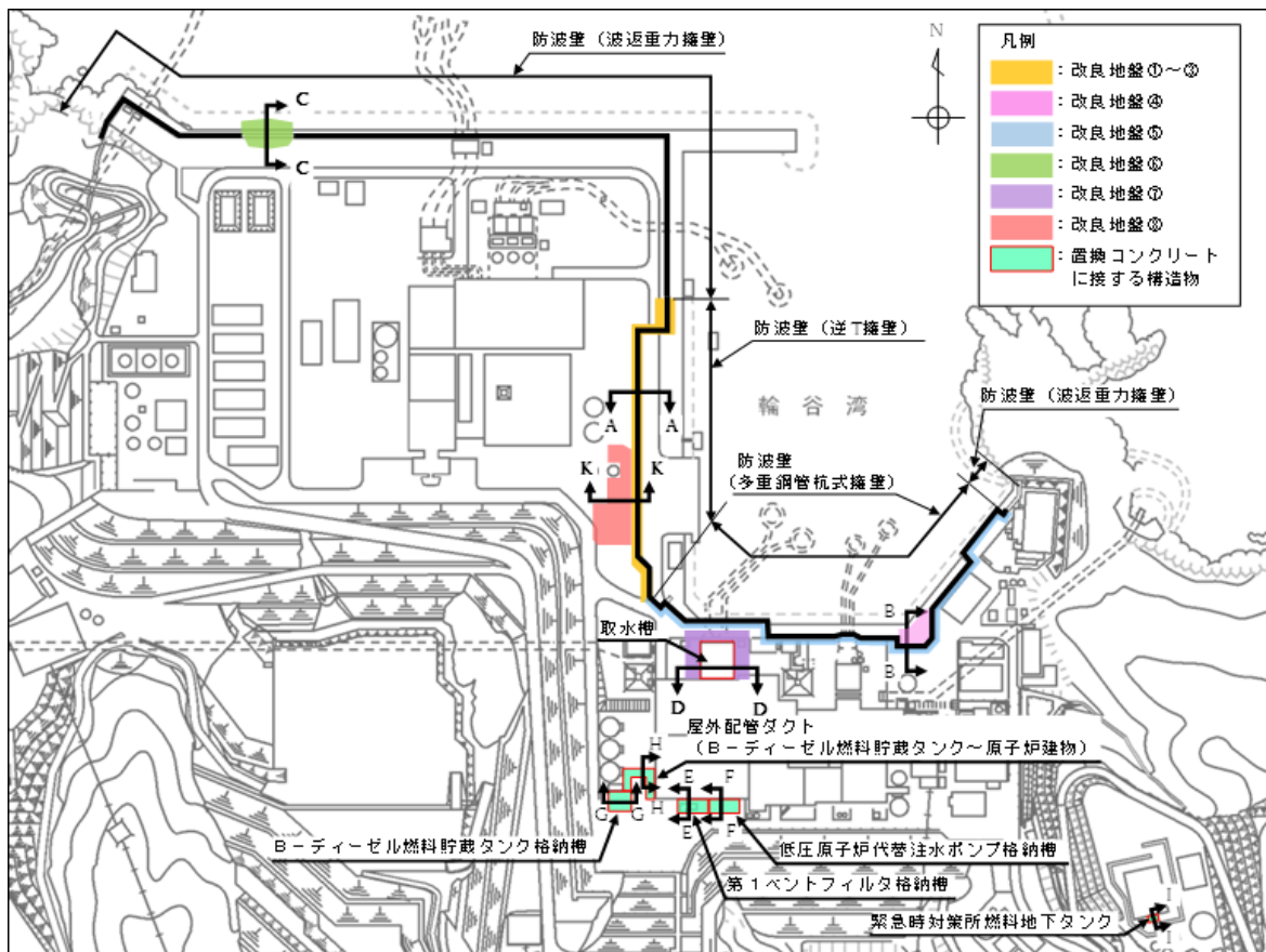
図1.1.10-13 改良地盤を設置する施設の平面配置図
