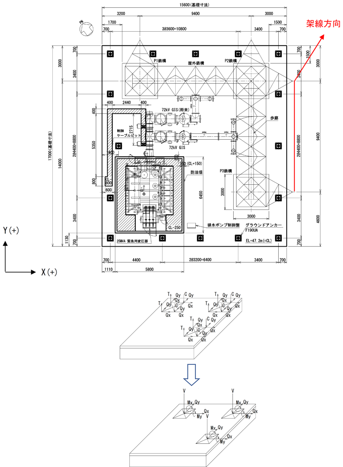
図 1.3.10-31 鉄構からの基礎荷重図
