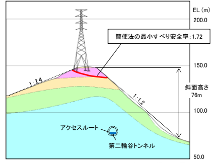
B-B' 断面
