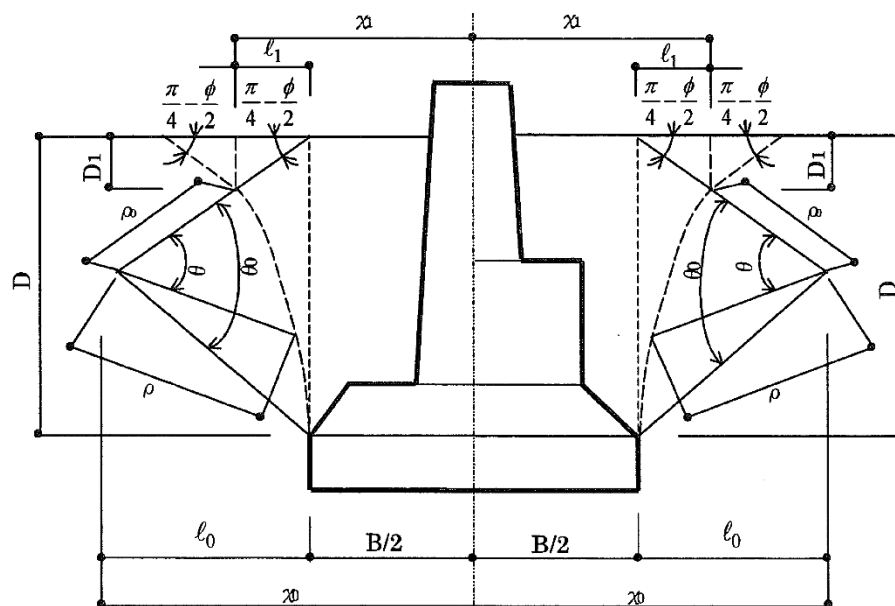
図1 基礎に引揚荷重が作用した場合の地盤のせん断破壊の模式図
