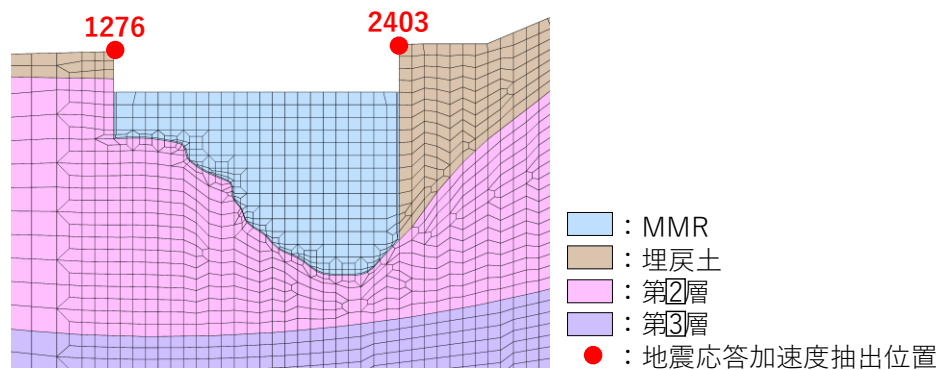
図 1.3.10-16 応答加速度抽出位置
