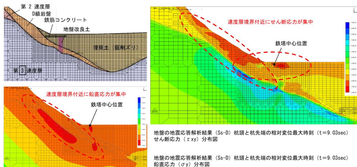
図1 220kV第二島根原子力幹線No. 1鉄塔の地盤の地震応答解析結果
