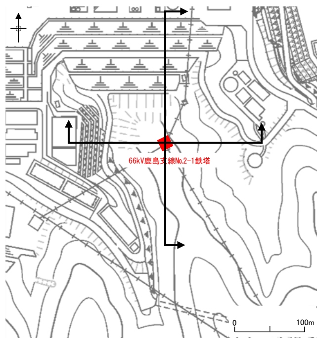
図 1.2.10-7 66kV 鹿島支線 No.2-1 鉄塔の南北方向及び東西方向の平面位置図
