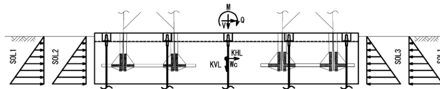
図 1.3.10-19 に荷重モデル図(安定性評価)を示す。
