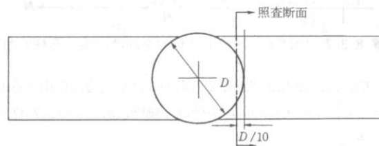
図 1.2.10-15 床板部の照査断面
