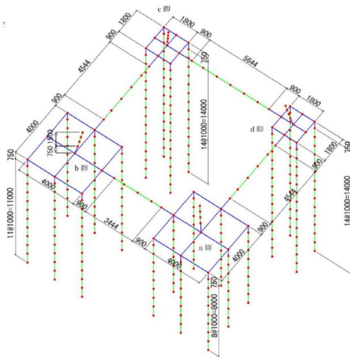
図 1.1.10-23 220kV 第二島根原子力幹線 No.1 鉄塔基礎解析モデル
