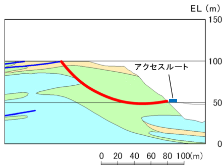
⑩－⑩' 断面
