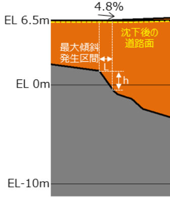
③-③断面
