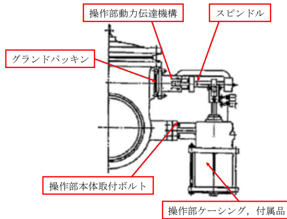
別紙 2-5-12 図 一般弁（逆止弁）の構造強度評価部位（操作装置付きの場合）
