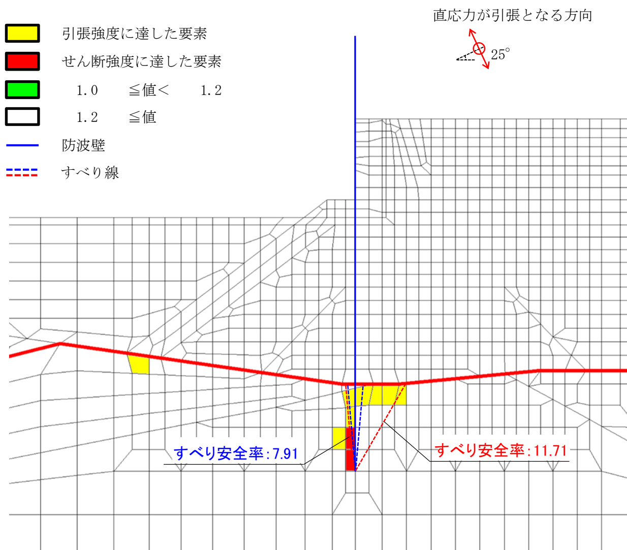
図 4.1.9-5 鋼管杭周辺岩盤の局所安全係数分布図 (④-④断面)
