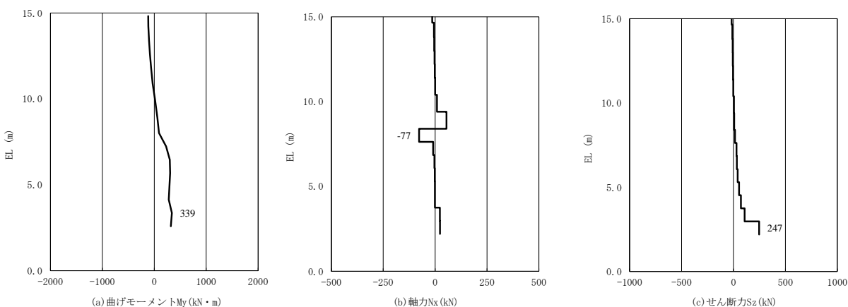
図 4.2.5-1 (2) コンクリートのせん断破壊に対する照査に用いる断面力 (③-③断面, S_s - D(-+) , 評価対象位置②)
