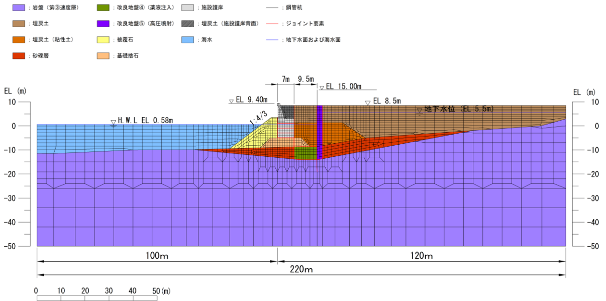
図 3.2.8-2 地震応答解析モデル (②-②断面)
