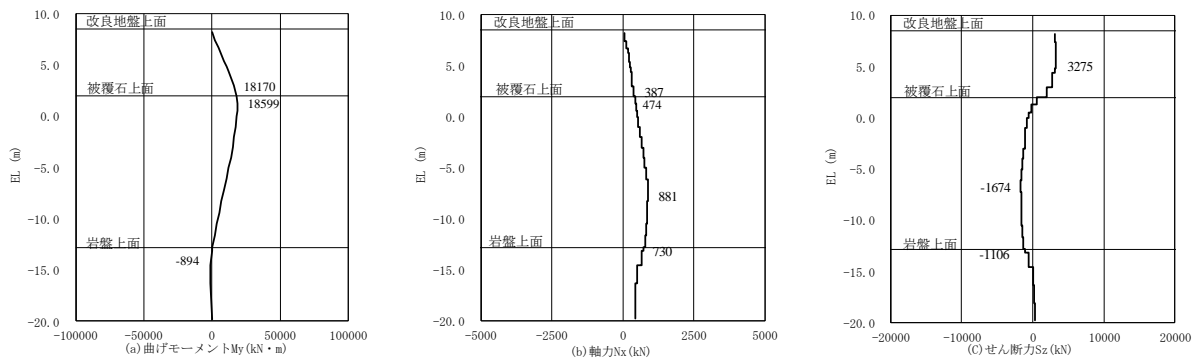
図 4.1.2-1(4) 鋼管杭の曲げ・軸力系破壊に対する照査
