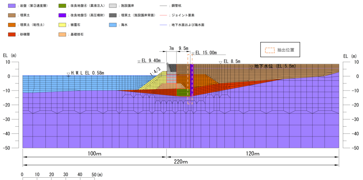
図 3.3.5-4(1) 応答加速度の抽出位置 (②-②断面)
