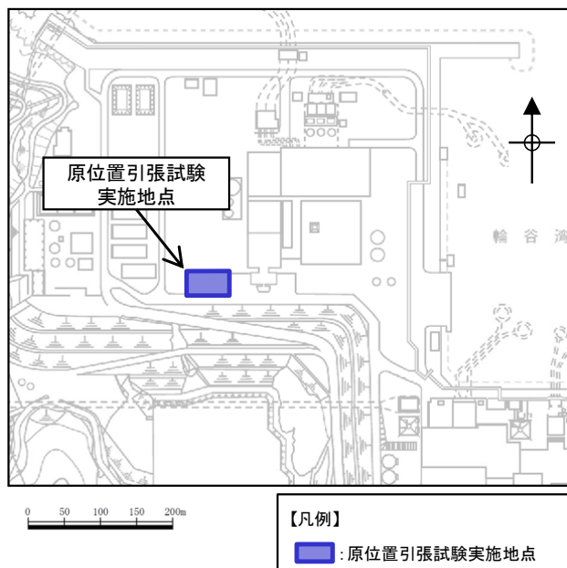
図 3.2.11-2 平面位置図
