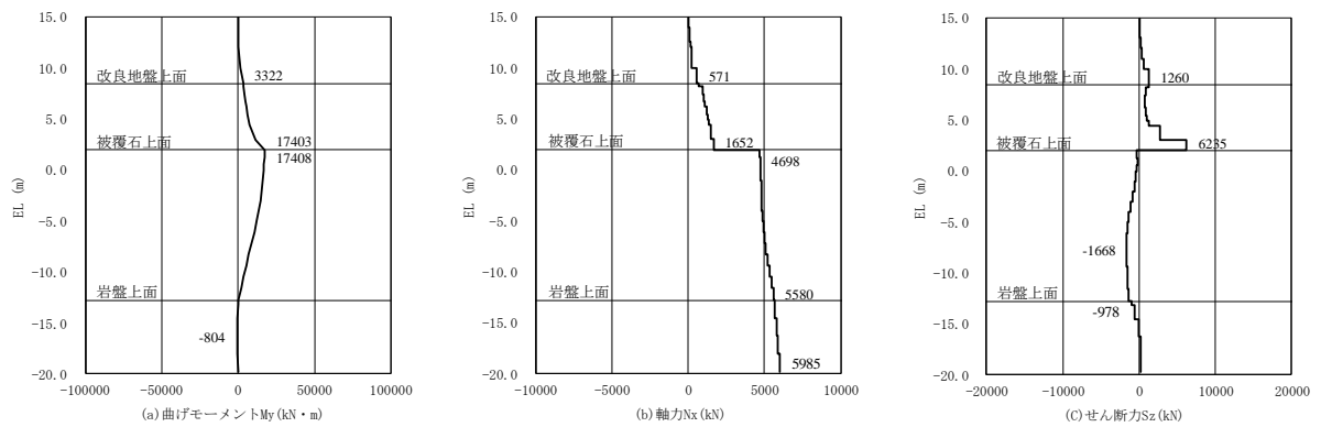
図 4.1.3-1(3) 鋼管杭のせん断破壊に対する照査における 最大照査値の評価時刻での断面力
