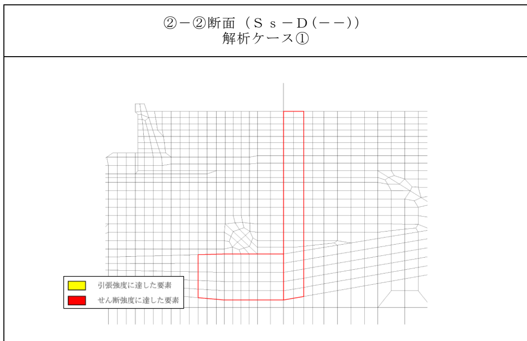
図 4.1.8-1(1) 全時刻における破壊履歴図 (②-②断面)
