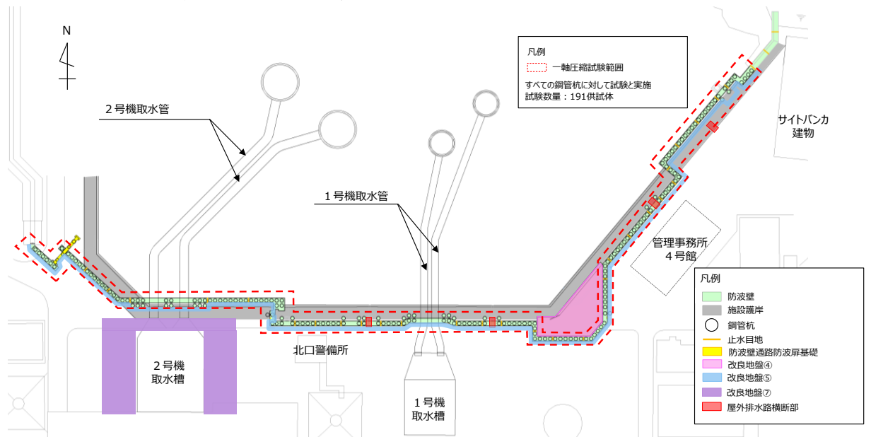
図 2-1 セメントミルクの一軸圧縮試験範囲
