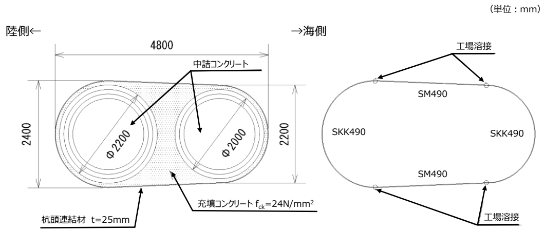
(平面図)
