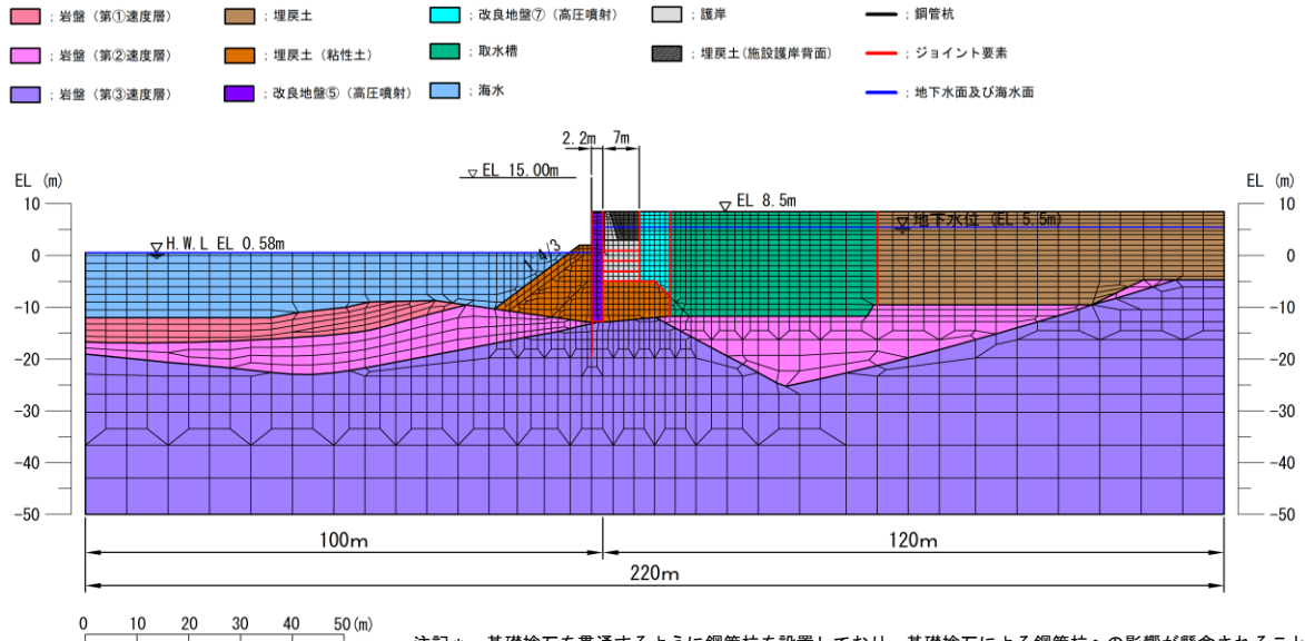
図 3.2.8-6 地震応答解析モデル (④-④断面)
