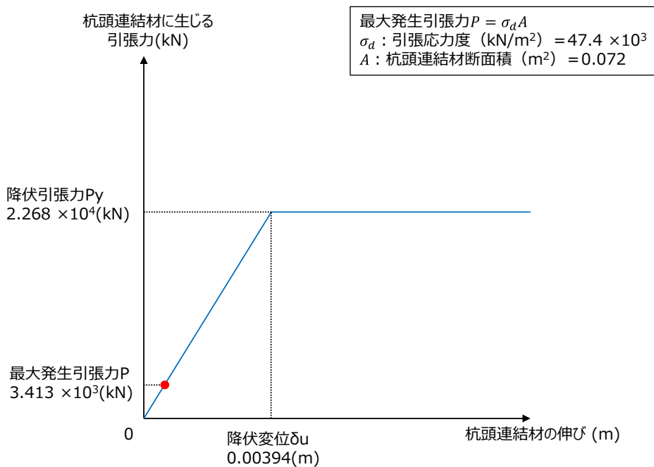
図 4.1.4-1 杭頭連結材の最大引張力発生時における引張力とひずみの関係
