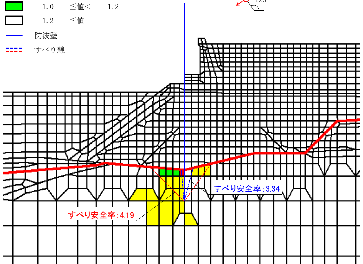
図 4.1.9-4 鋼管杭周辺岩盤の局所安全係数分布図 (③-③断面)
