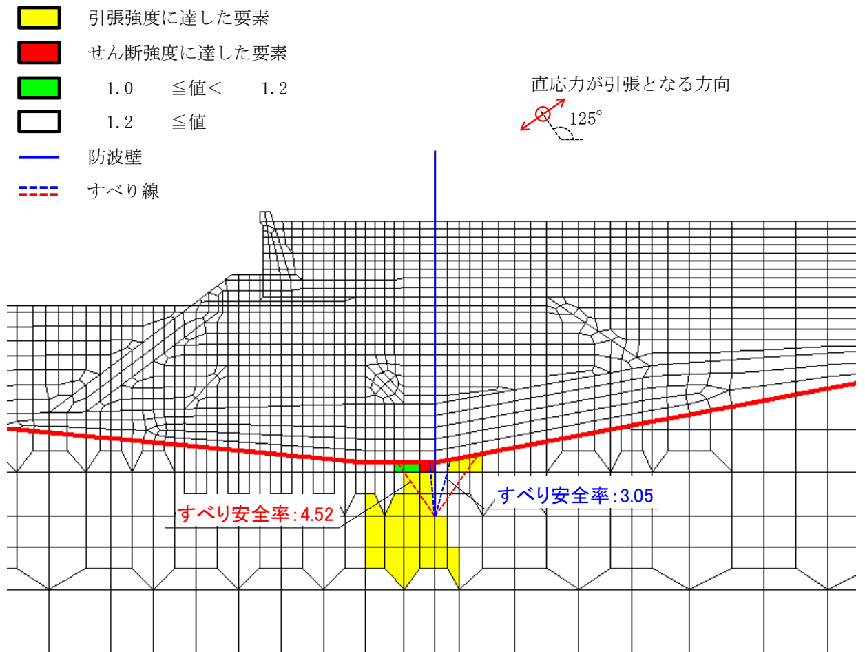
図 4.1.9-3 鋼管杭周辺岩盤の局所安全係数分布図 (②-②断面)
