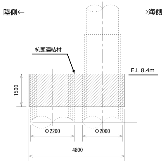
(断面図)
