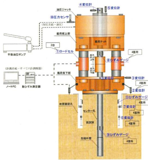
図 3. 2. 11-5 試験装置の概要
