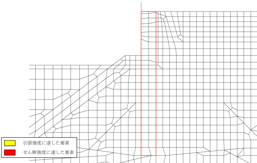
図 4.1.8-1(2) 全時刻における破壊履歴図 (③-③断面, ④-④断面)
