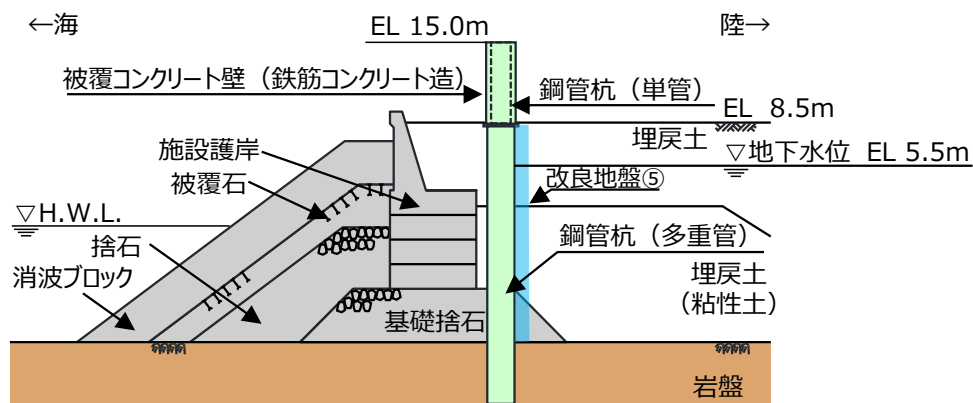
図 2.2-2 防波壁（多重鋼管杭式擁壁）の構造概要図（断面図）
