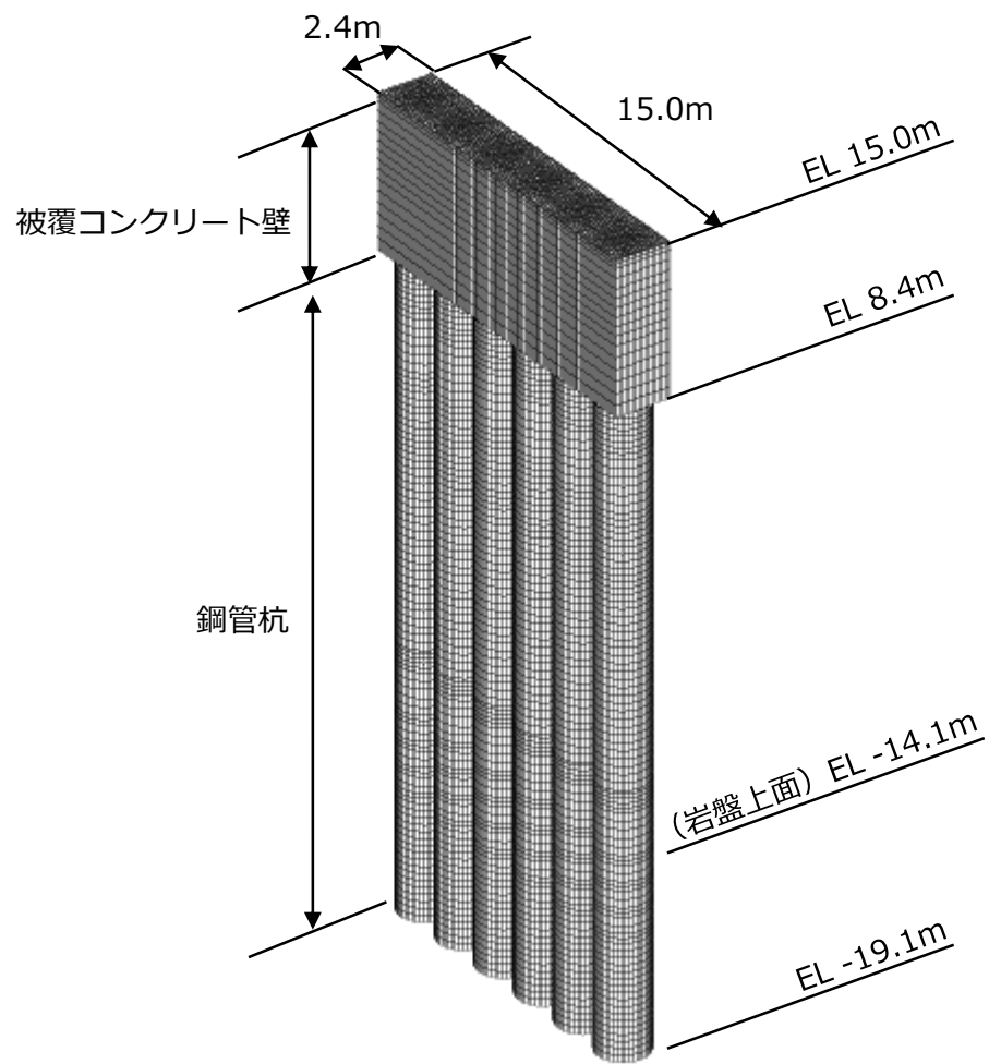
図 3.3.3-1 ②—②断面を含む区間における 3次元構造解析モデル
