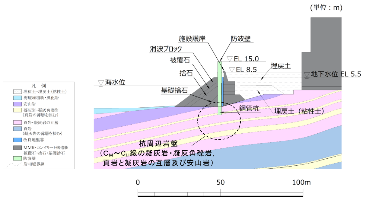
図 3.2.11-10 岩相区分図 (③-③断面)
