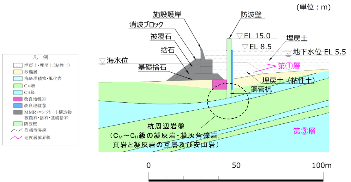
図 3.2.11-7 岩級区分図 (②-②断面)
