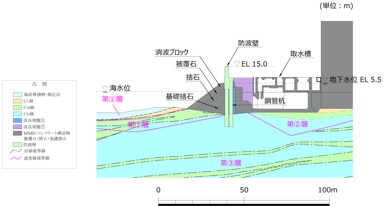
図 3.2.8-7 地質断面図 (④-④断面)
