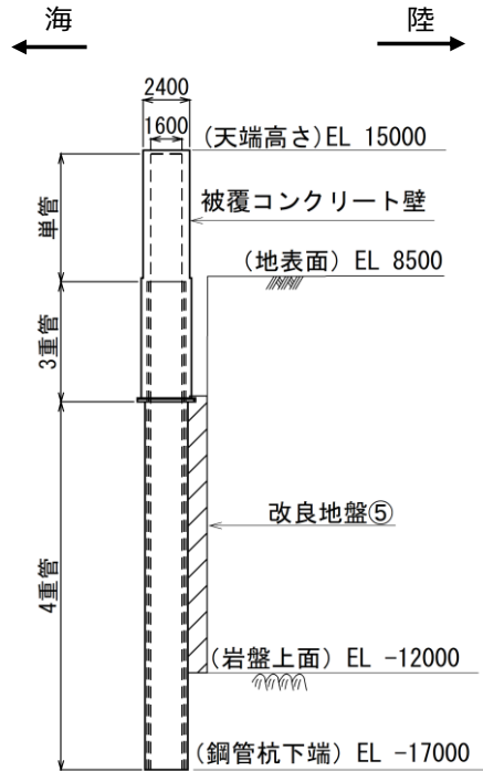
(断面図)
