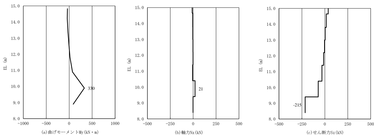
図 4.2.5-1 (1) コンクリートのせん断破壊に対する照査に用いる断面力 (②-②断面, S_s - D(-+) , 評価対象位置⑤)
