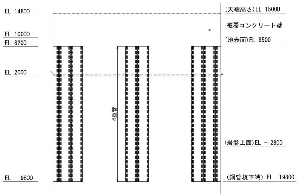
(正面図)
