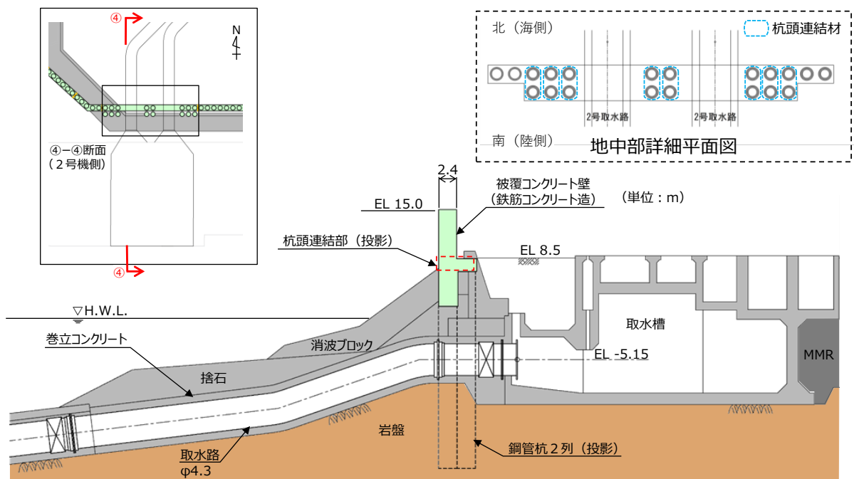
図3.2.8-15 防波壁（多重鋼管杭式擁壁）の④-④断面（断面図）
