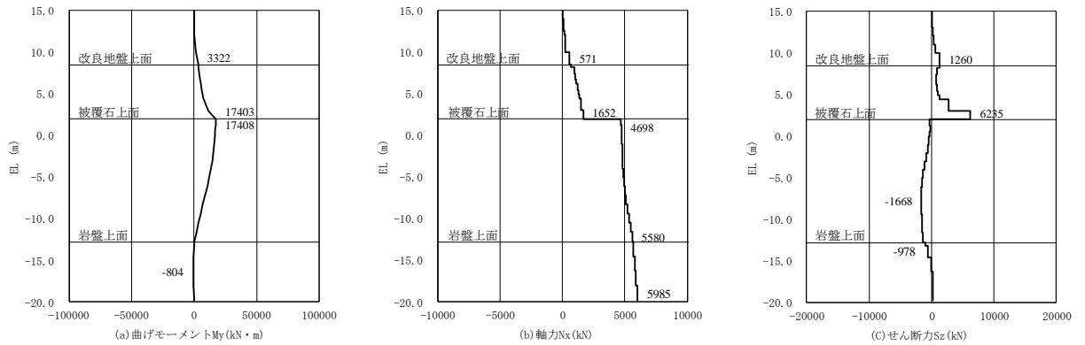
図 4.1.2-1(3) 鋼管杭の曲げ・軸力系破壊に対する照査
