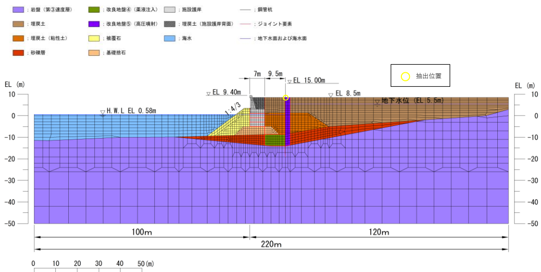
図 3.3.5-5(1) 鋼管杭変位の抽出位置 (②-②断面)
