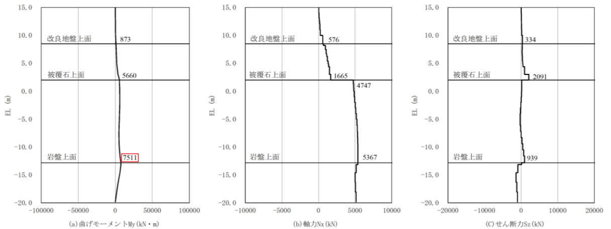
図 4.1.9-2 岩盤上面において鋼管杭に作用する曲げモーメントが
