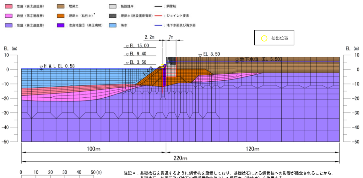
図 3.3.5-5(2) 鋼管杭変位の抽出位置 (③-③断面)
