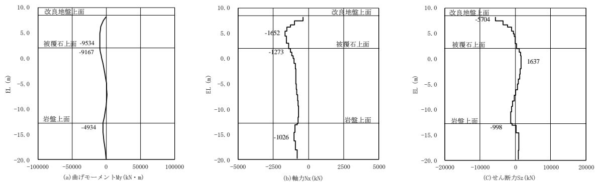
図 4.1.3-1(4) 鋼管杭のせん断破壊に対する照査における 最大照査値の評価時刻での断面力
