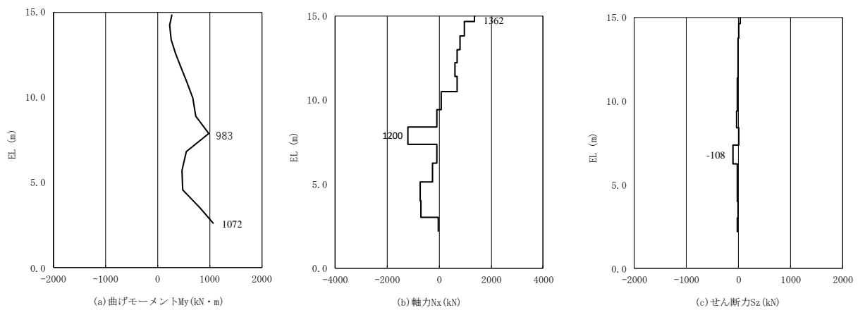
図 4.2.4-2(3) 鉄筋の曲げ・軸力系破壊に対する照査に用いる断面力 (④-④断面, S_s - D(+) , 評価対象位置④)
