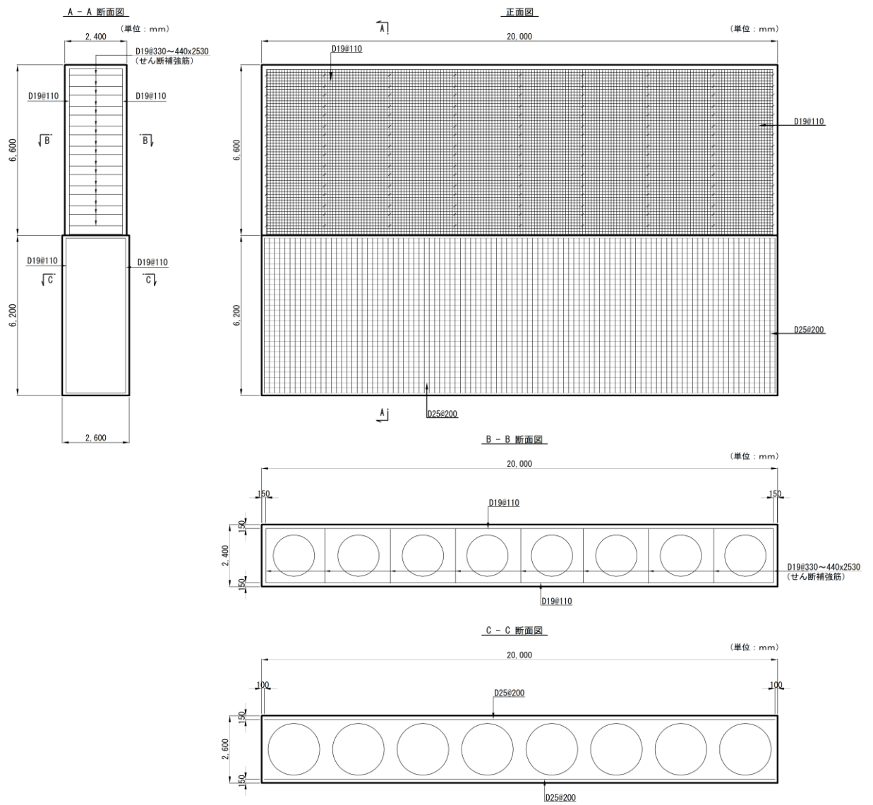
図 3.1-14 防波壁（多重鋼管杭式擁壁）の概略配筋図（③-③断面）
