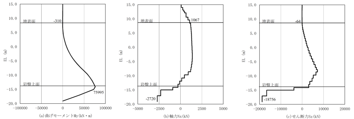
図 4.1.3-1(1) 鋼管杭のせん断破壊に対する照査における
