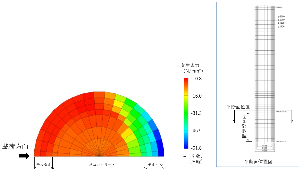
図 4-6(2) 中詰コンクリート及びモルタル（充填材）の応力図（平断面図） （実構造物スケール解析，降伏モーメント超過時，最小主応力）
