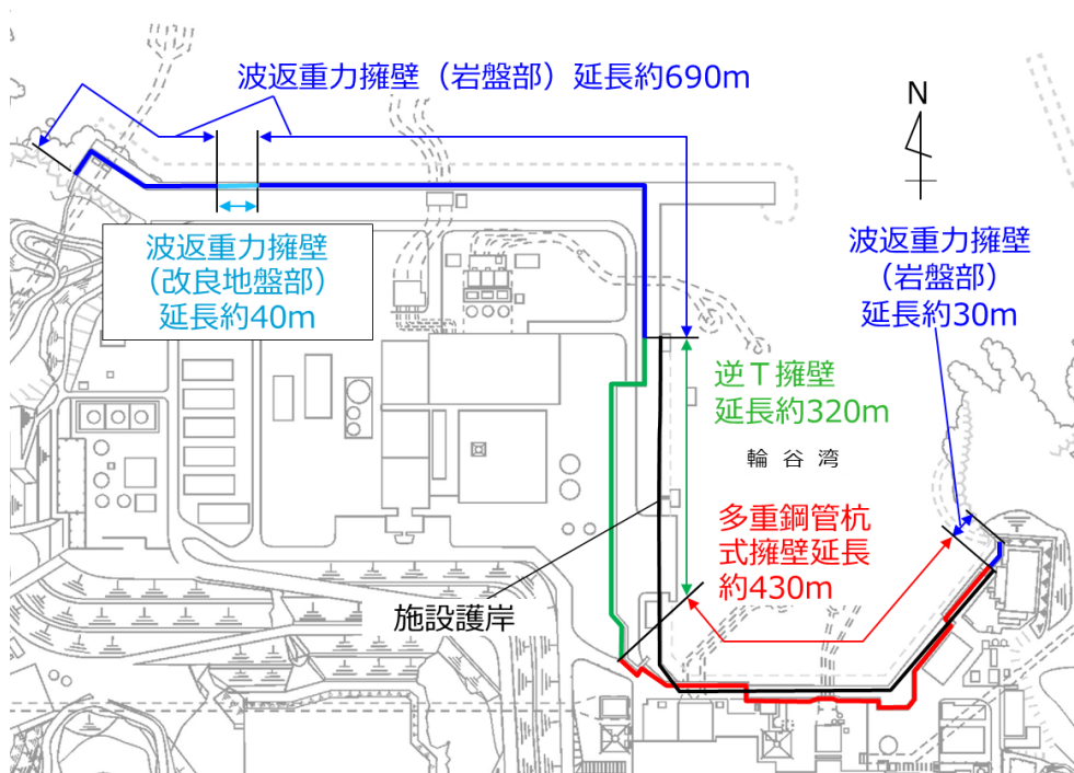
図 4.1.12-1 防波壁と施設護岸の配置（全体平面図）
