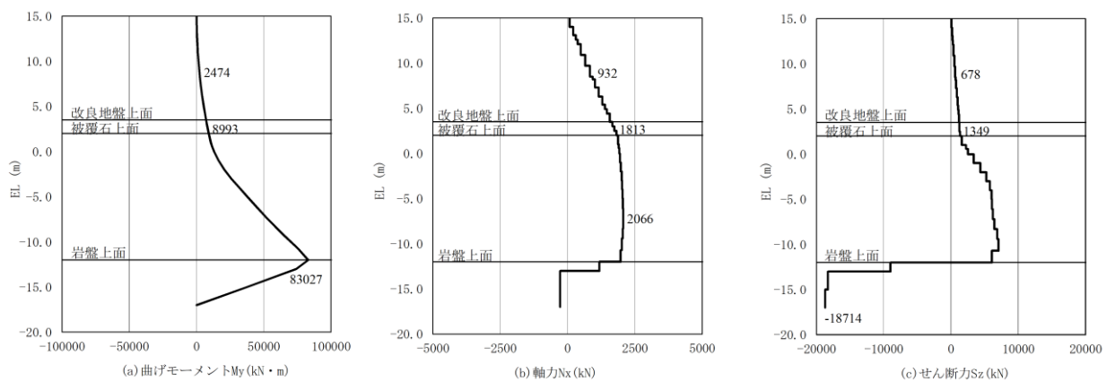
図 4.1.3-1(2) 鋼管杭のせん断破壊に対する照査における
