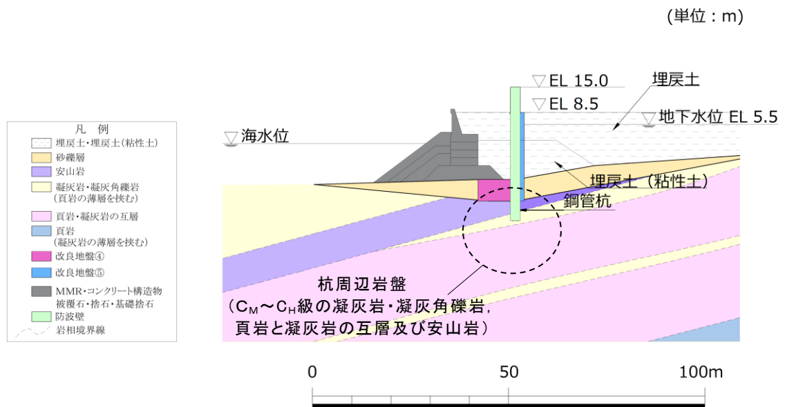
図 3.2.11-8 岩相区分図 (②-②断面)
