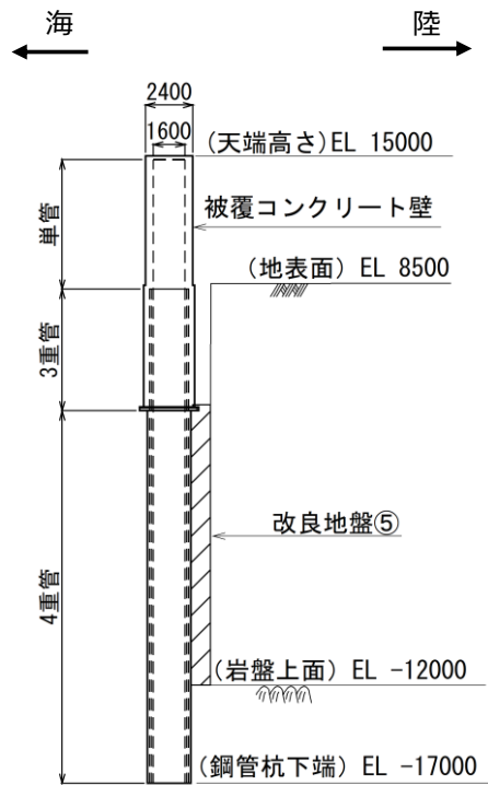
(断面図)
