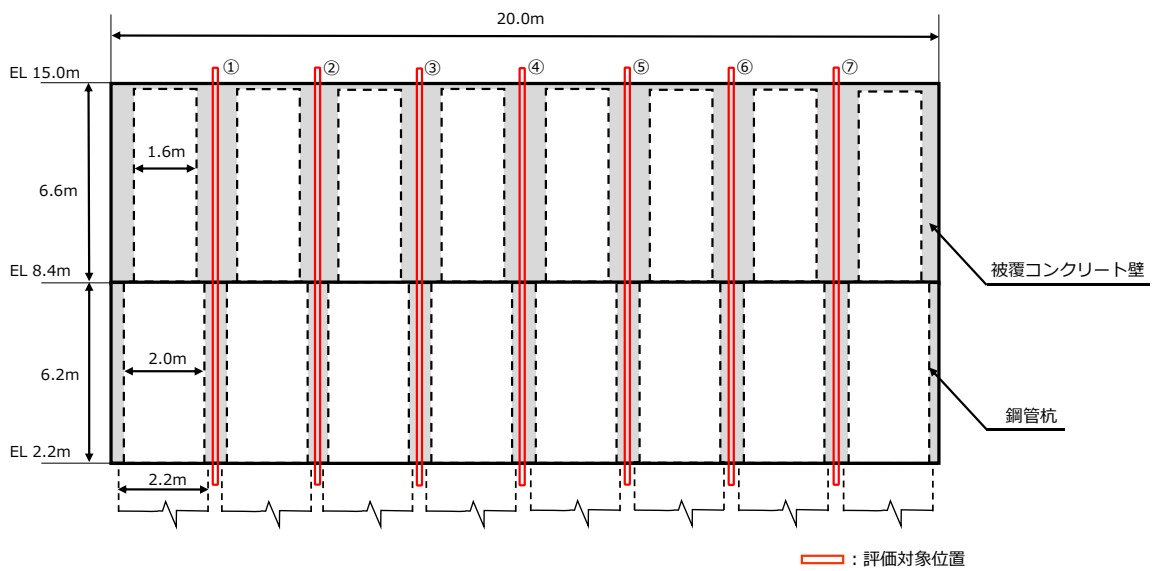
図 4.2.3-1(5) 評価対象位置図 (③-③断面 正面図)
