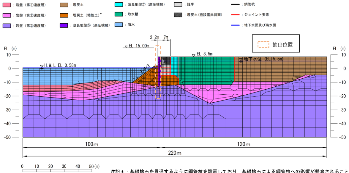
図 3.3.5-4(3) 応答加速度の抽出位置 (④-④断面)
