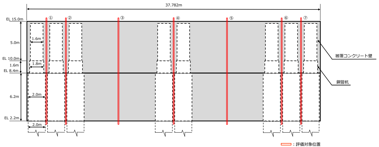
図 4.2.3-1(6) 評価対象位置図 (④-④断面 正面図)
