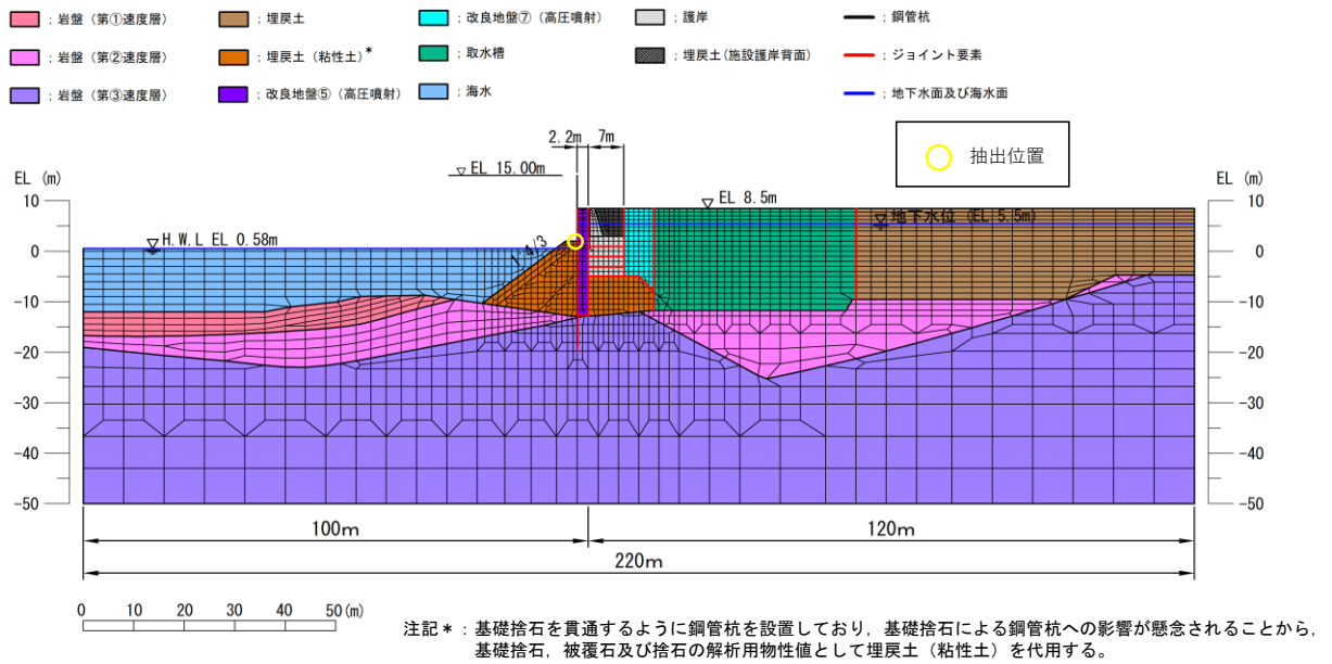
図 3.3.5-5(3) 鋼管杭変位の抽出位置（④-④断面）
