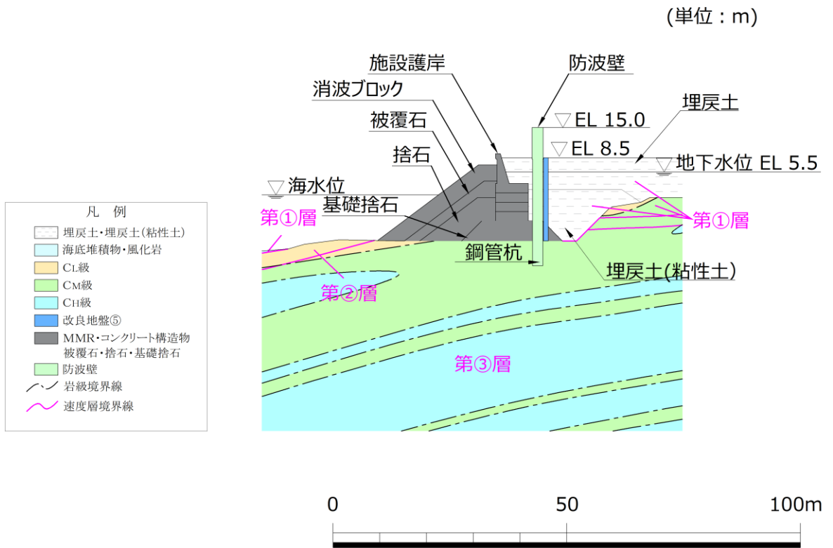
図 3.1-3 評価対象断面図 (①-①断面)
