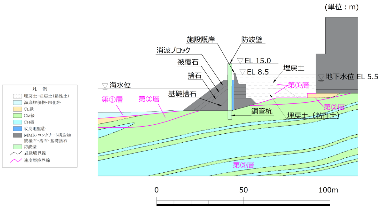
図 3.1-5 評価対象断面図 (③-③断面)
