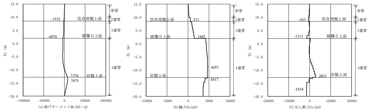
図 2.2-3(4) 4重管部の鋼管杭のせん断破壊に対する4重管部の照査
