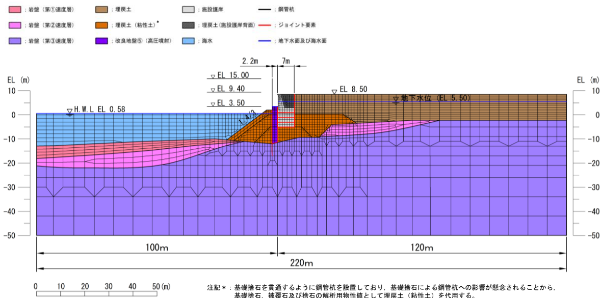
図 3.2.8-4 地震応答解析モデル (③-③断面)
