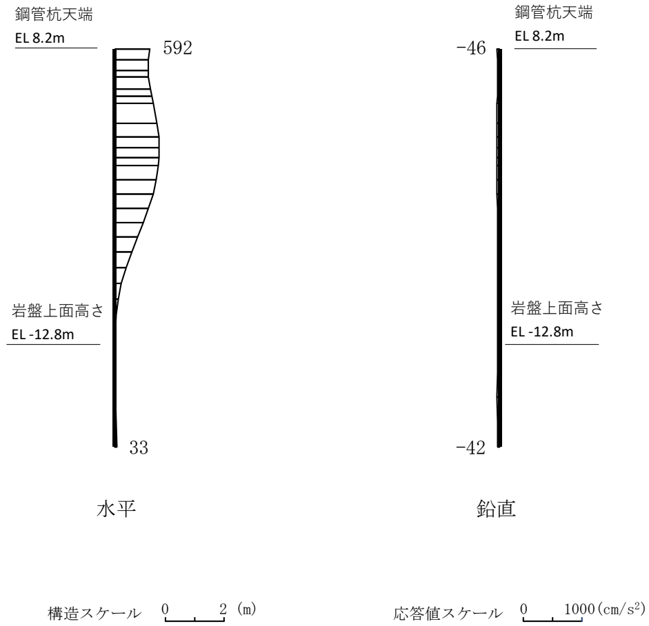
図 4.2.2-10 作用荷重分布図 (応答加速度分布) (解析ケース②, S s - D (+ -), ④-④断面, 陸側杭)
