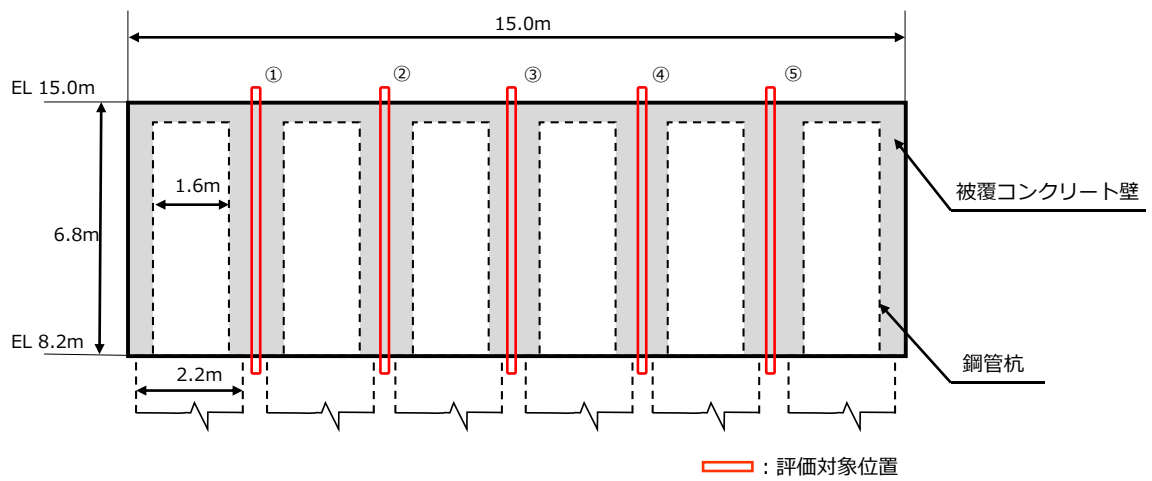
図 4.2.3-1(4) 評価対象位置図 (②-②断面 正面図)
