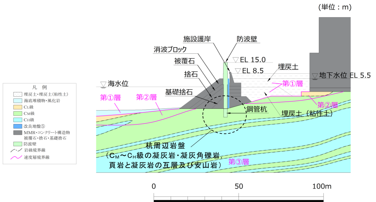
図 3.2.11-9 岩級区分図 (③-③断面)
