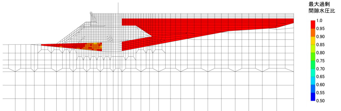
図 4.1.12-10 施設護岸等がある場合の過剰間隙水圧比最大値分布
