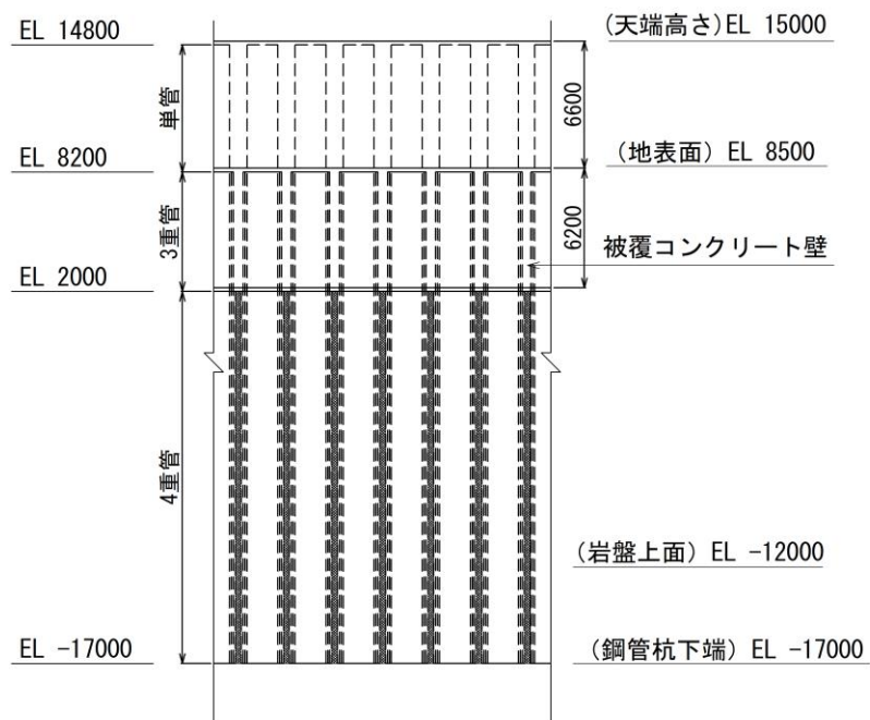
(正面図)
