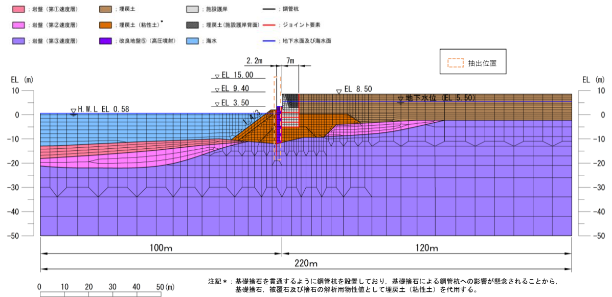
図 3.3.5-4(2) 応答加速度の抽出位置 (③-③断面)
