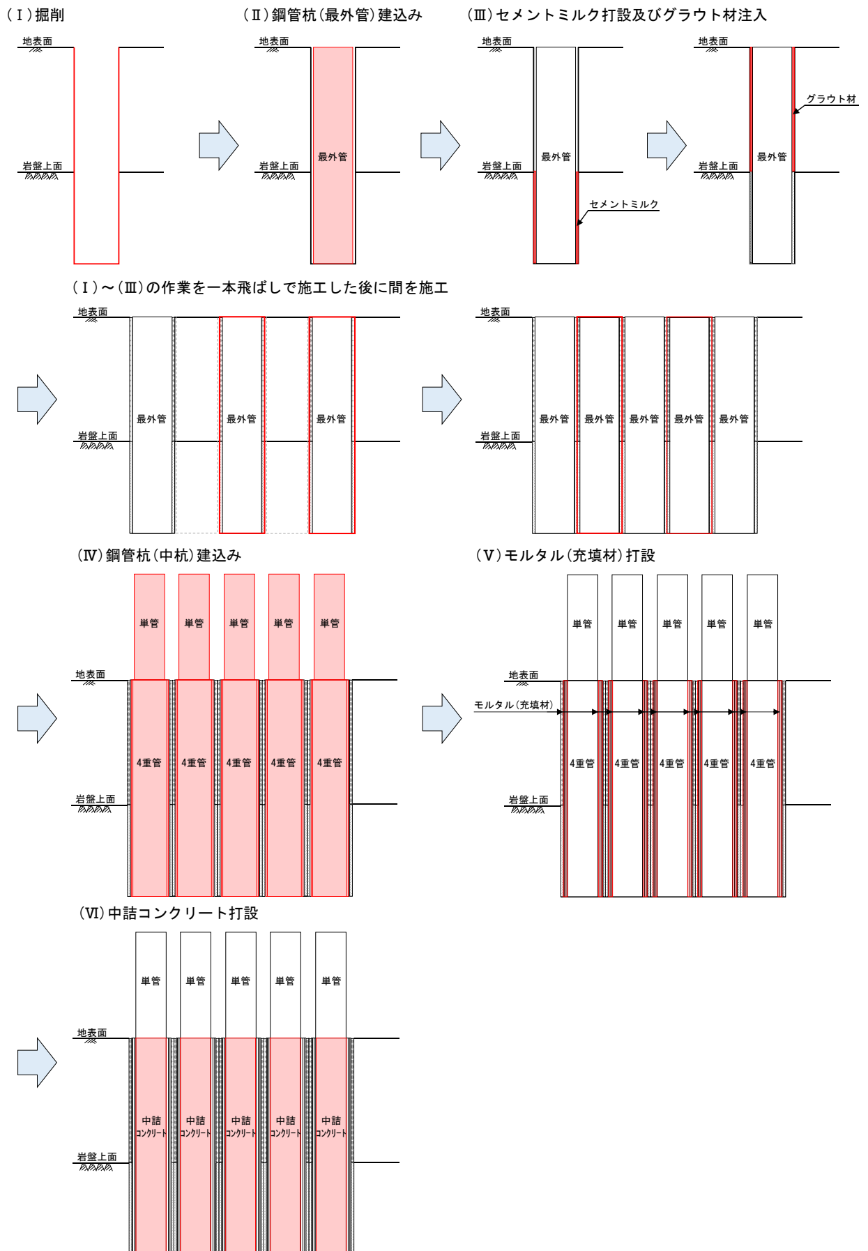
図 2.2-6 多重鋼管杭の施工ステップ図
