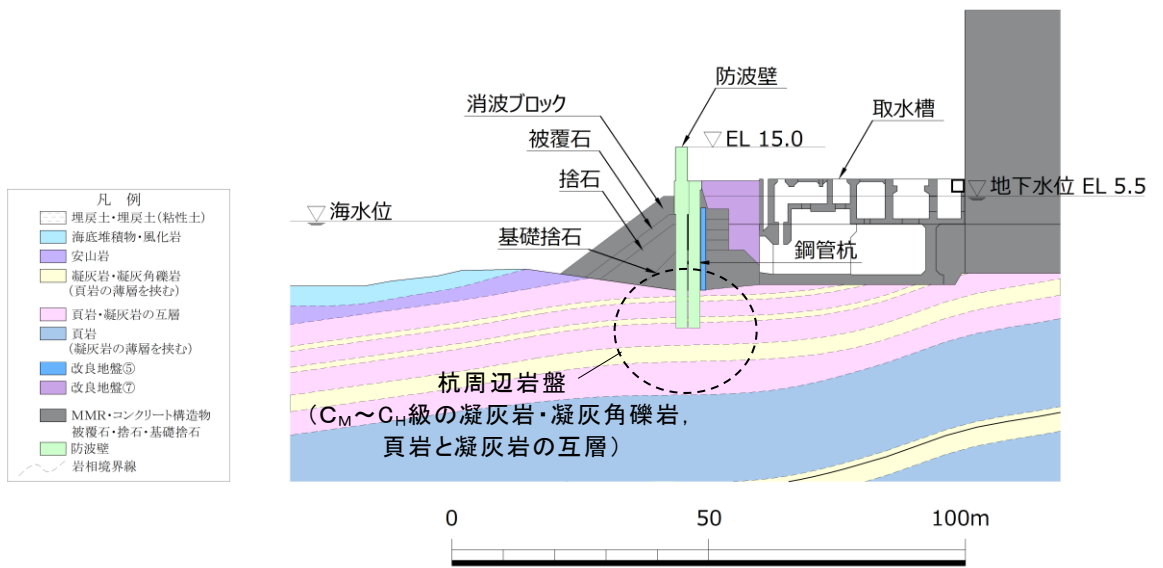
図 3.2.11-12 岩相区分図 (④-④断面)
