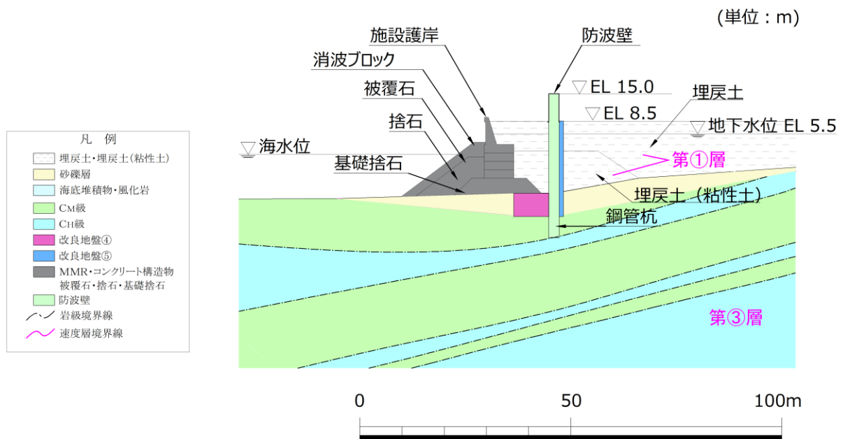
図 3.2.8-3 地質断面図 (②-②断面)
