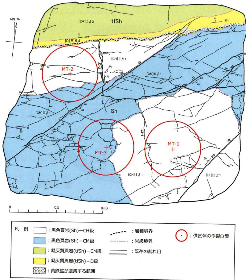
図 3.2.11-3 試験を実施したピット底盤の地質状況及び試験位置図 (南側)
