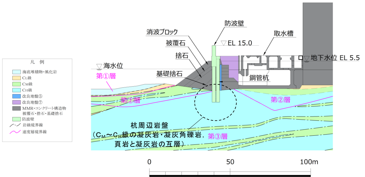
図 3.2.11-11 岩級区分図 (④-④断面)
