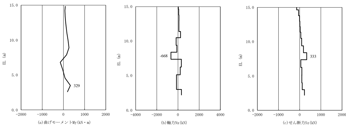
図 4.2.5-1 (3) コンクリートのせん断破壊に対する照査に用いる断面力 (④-④断面, S_s - D(+) , 評価対象位置①)
