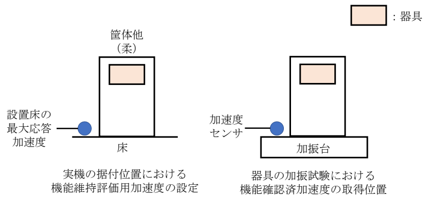
図 3-4 筐体他が柔な設備かつ筐体他を含めた加振試験を実施した場合
