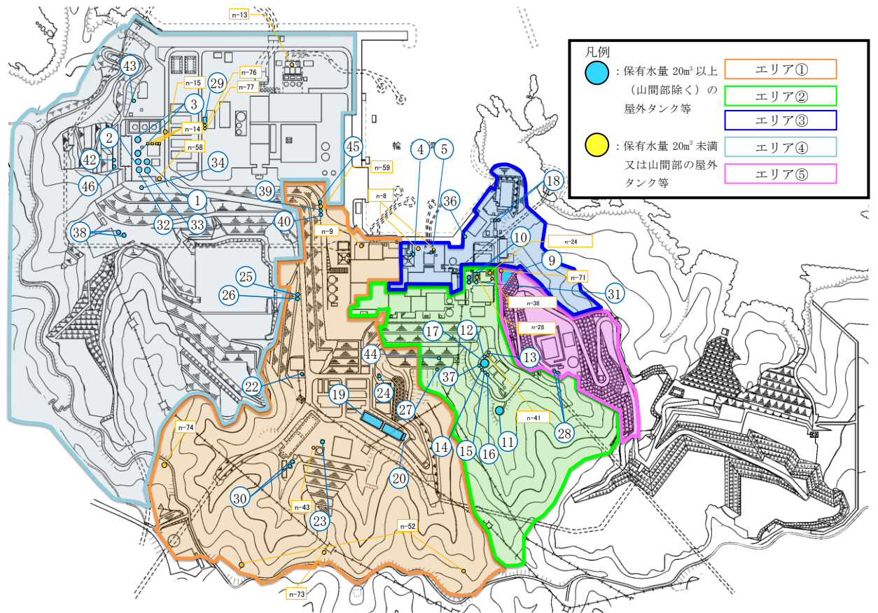
図 2-2 屋外タンク等の配置
