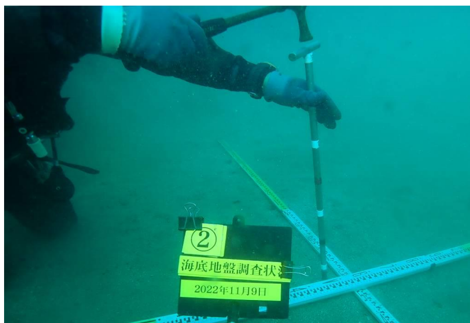
図 2-12 鉄筋棒貫入状況 (ハンマー使用) (参考) 19-10
