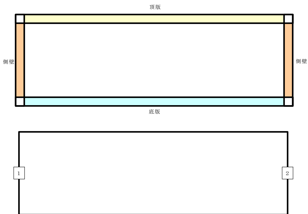
図 5-8 評価位置図 (B-B 断面)
