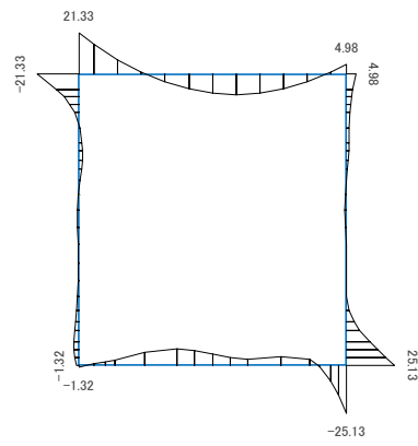
(a) 曲げモーメント (kN・m)
