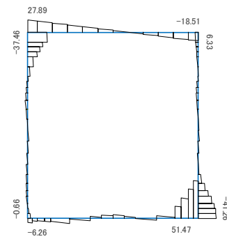
(c) せん断力 (kN)
