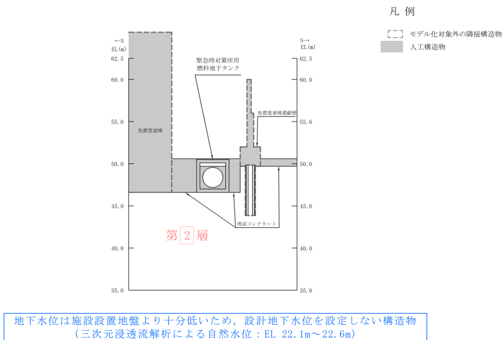
図3-7 評価対象地質断面図 (A-A断面)
