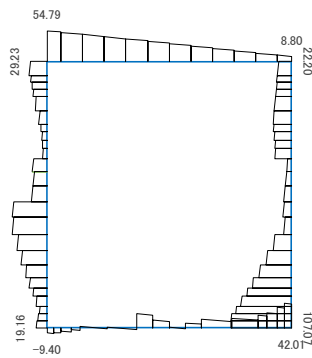
(a) 曲げモーメント (kN・m)
