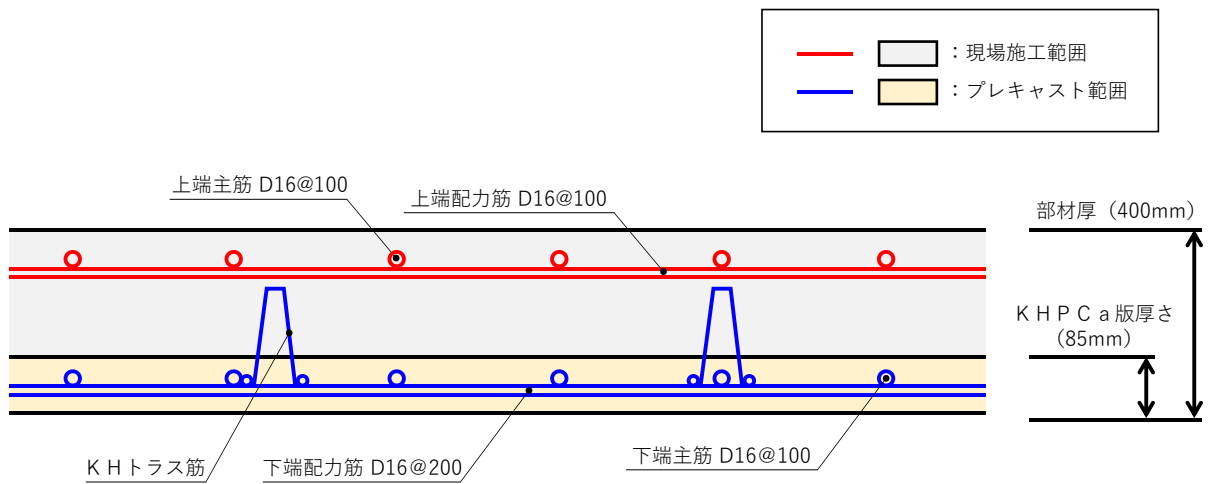
図 2-6 緊急時対策所用燃料地下タンク 概略配筋図 (B-B 断面)
