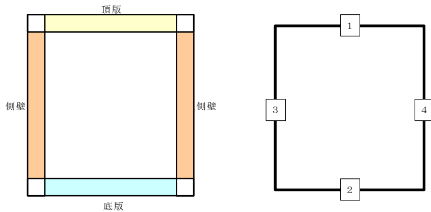
図 5-7 評価位置図（A-A 断面）
