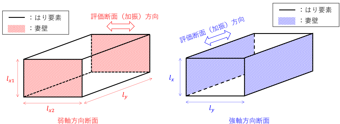
図 2-1 短スパン l_x 及び長スパン l_y の比率の考え方
