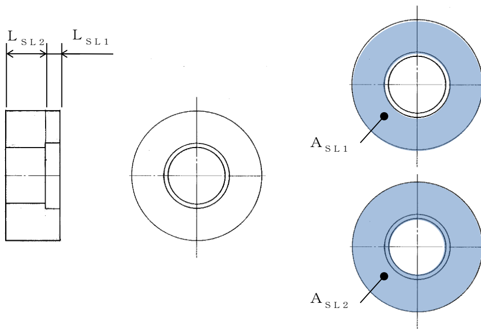
図 2.2.1.2.2-11 スリーブ概略図
