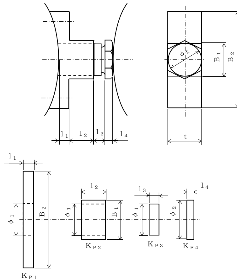
図 2.1.4-10 制御棒駆動機構ハウジング間及び制御棒駆動機構ハウジング/レストレントビーム間のラテラルレストレートの構成部材構造図
