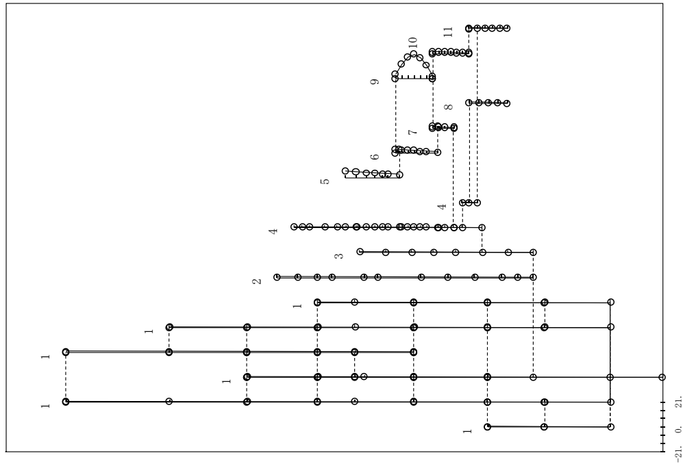
図 2.2.2-13 (21/40) 刺激関数 (第 1 次モード, E-W方向) : 影響検討モデル 3
