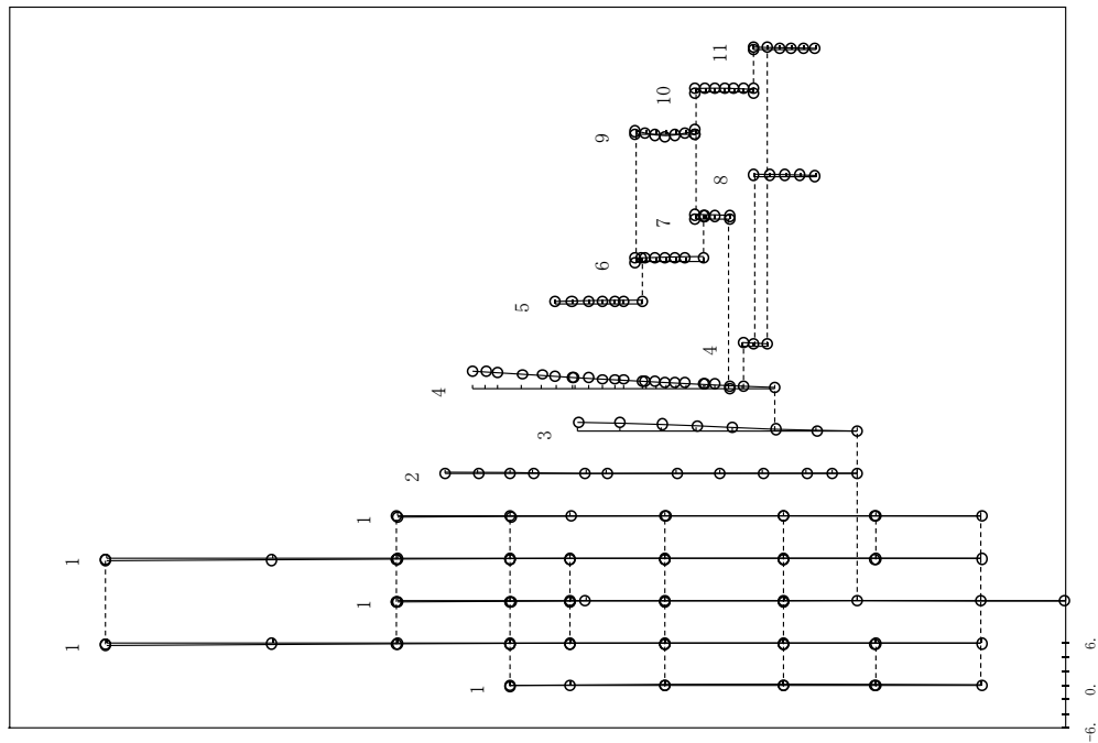
図 2.2.2-8 (8/40) 刺激関数 (第 4 次モード, NS 方向)
