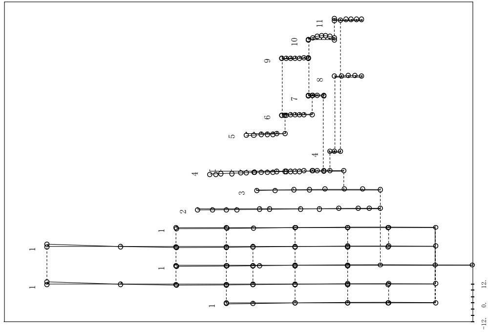
図 2.2.2-8 (11/40) 刺激関数 (第 6 次モード, N S 方向) : 影響検討モデル 2
