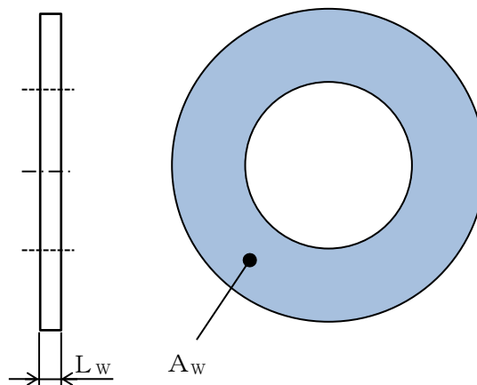
図 2.2.1.2.2-13 ワッシャ概略図
