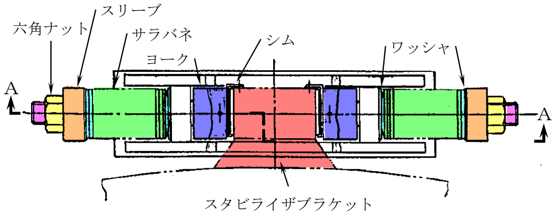
原子炉圧力容器スタビライザ平面図
