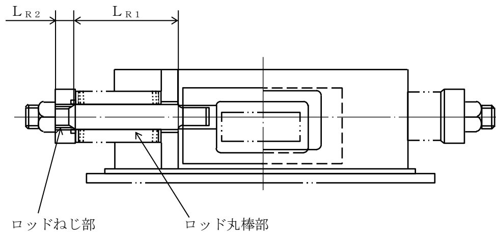
図 2.2.1.2.2-7 ロッド概略図
