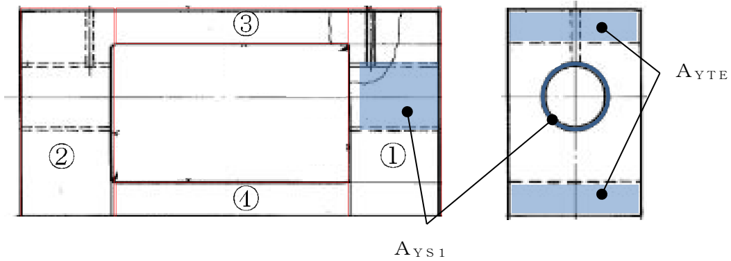
図 2.2.1.2.2-9 ヨークのばね定数算定のための計算モデル分割
