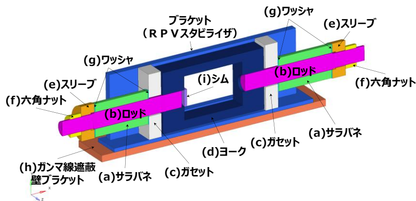
断面図
