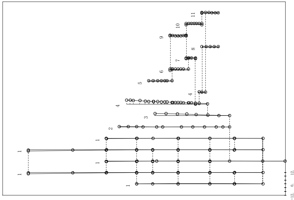
図 2.2.2-8 (7/40) 刺激関数 (第 4 次モード, NS 方向)
