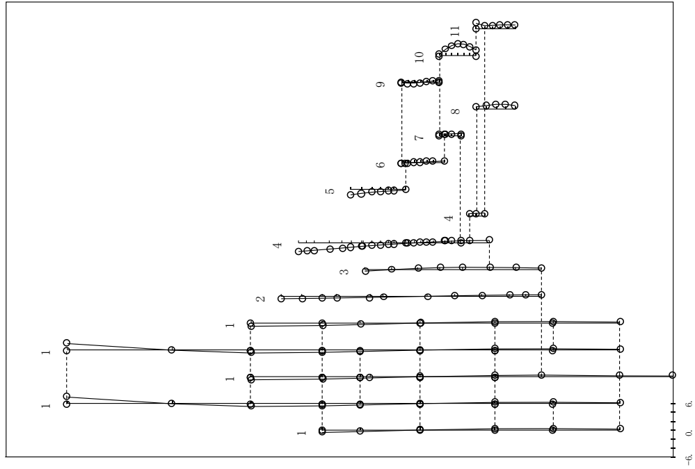
図 2.2.2-8 (12/40) 刺激関数 (第 6 次モード, N S 方向) : 今回工認モデル
