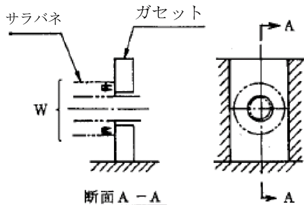
図 2.2.1.2.2-8 ガセットの構造
