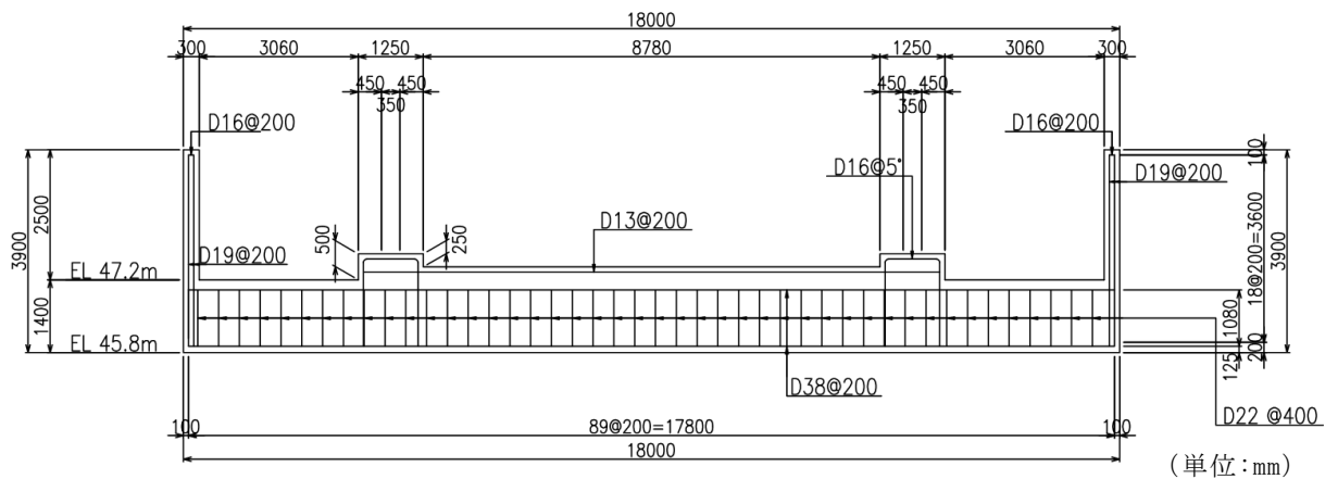
図 2-4 ガスタービン発電機用軽油タンク基礎 概略配筋図
