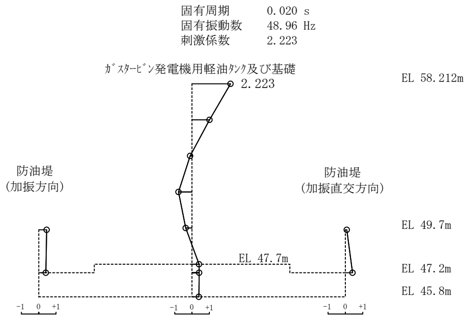
図 3-10(4) 刺激関数図 (解析ケース①, 水平方向, 4次モード)
