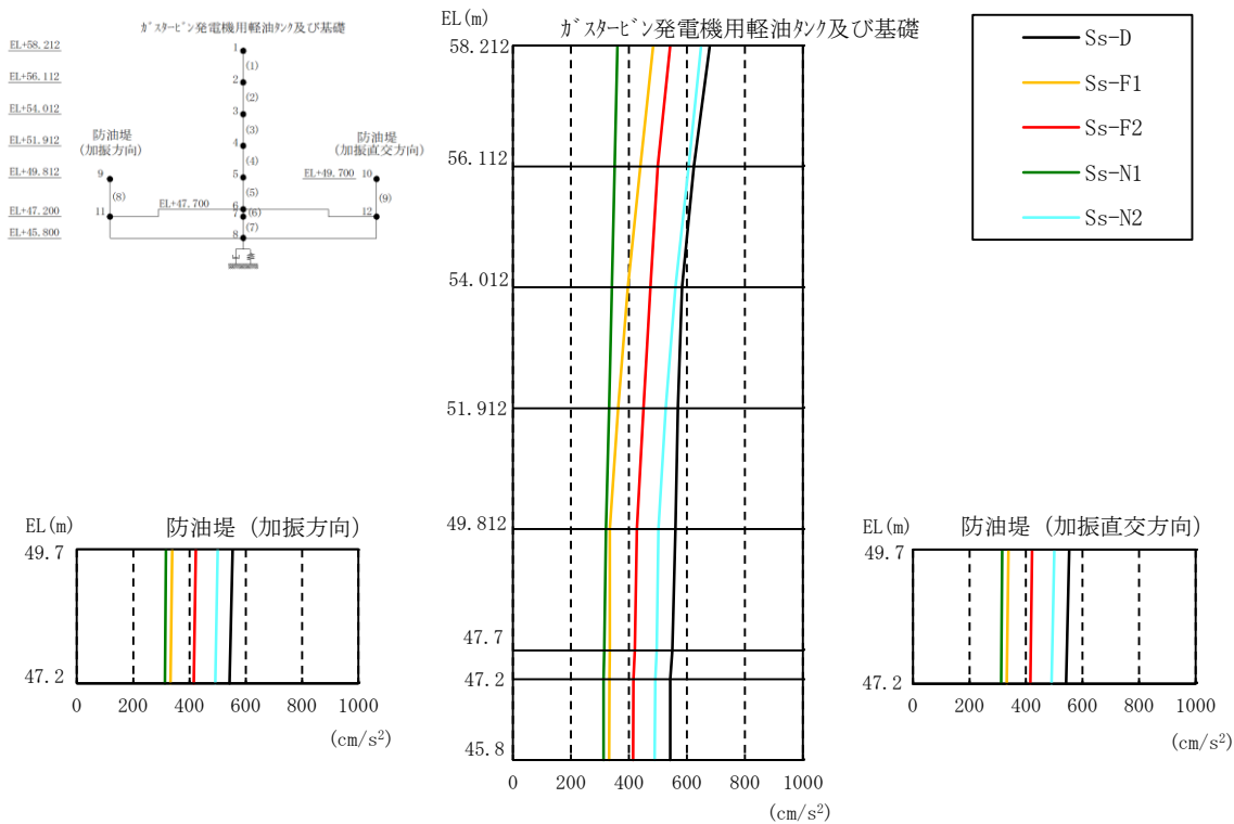
図 3-61 最大応答加速度（鉛直方向，解析ケース②）
