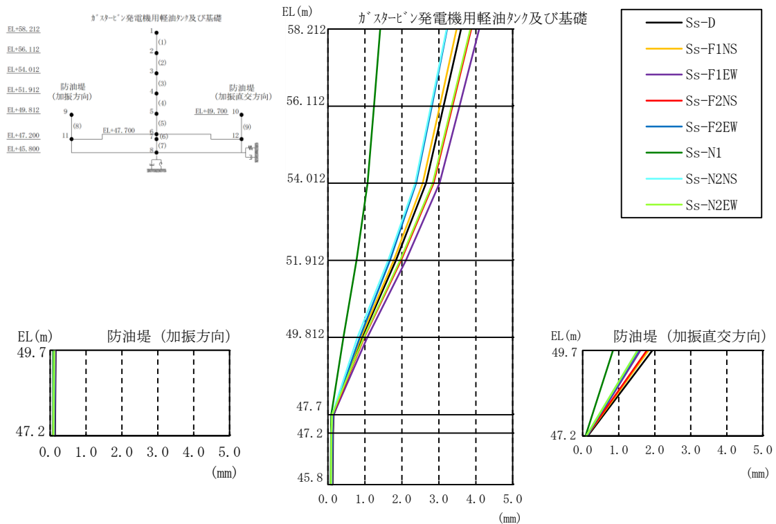
図 3-62 最大応答変位（水平方向，解析ケース②）
