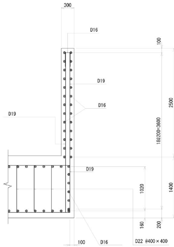
图 3-2 防油堤 概略配筋图 (A-A 断面)
