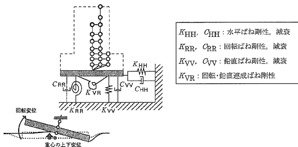
図3-4 誘発上下動を考慮した多質点系モデルの概念図
