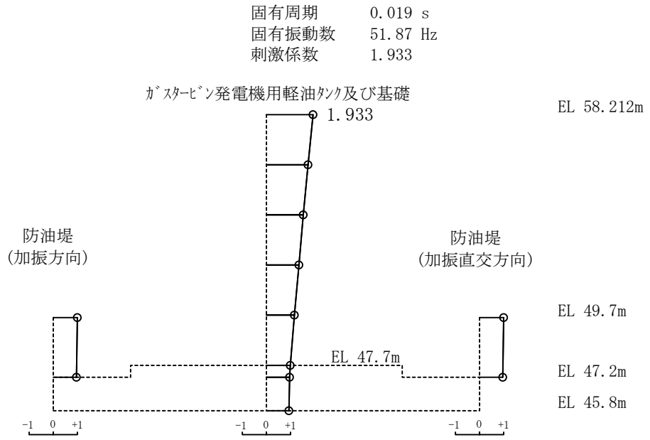
図 3-11(1) 刺激関数図 (解析ケース①, 鉛直方向, 1次モード)
