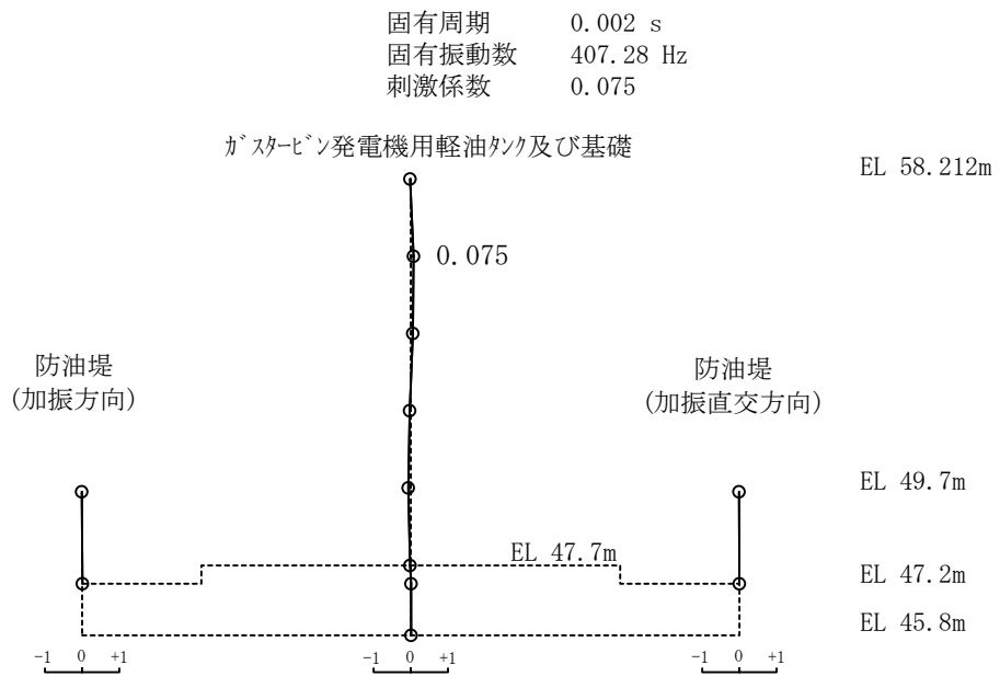
図 3-11 (6) 刺激関数図 (解析ケース①, 鉛直方向, 6 次モード)
