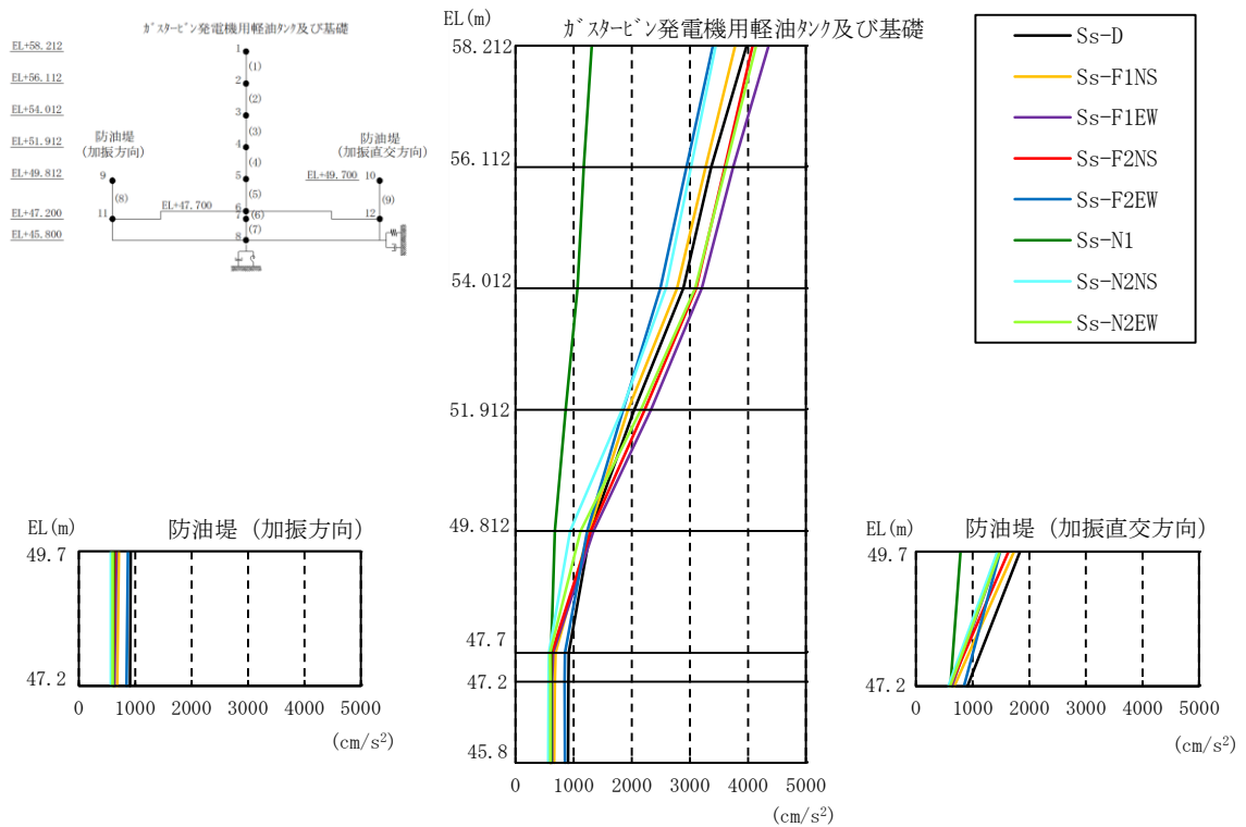
図 3-60 最大応答加速度（水平方向，解析ケース②）
