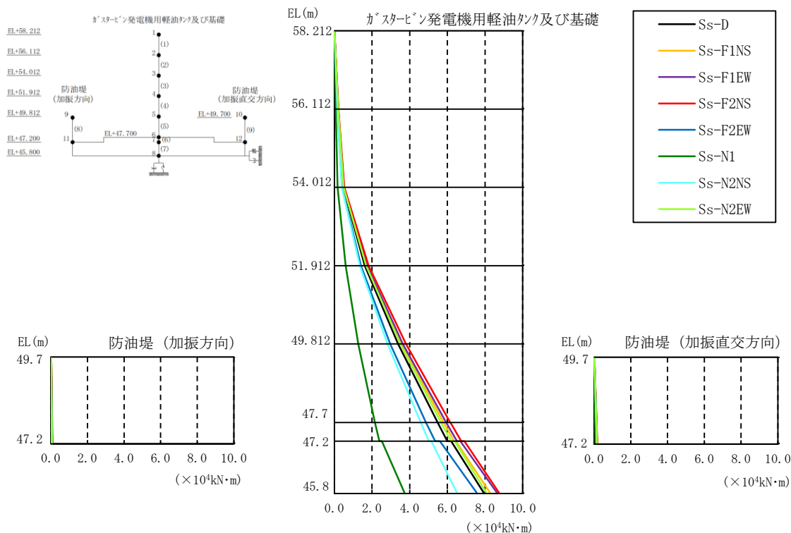
図 3-58 最大応答曲げモーメント（解析ケース①）
