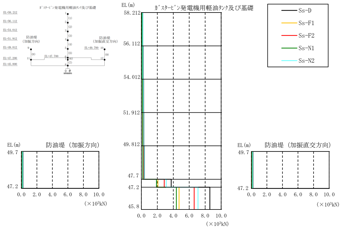
図 3-73 最大応答軸力（解析ケース③）
