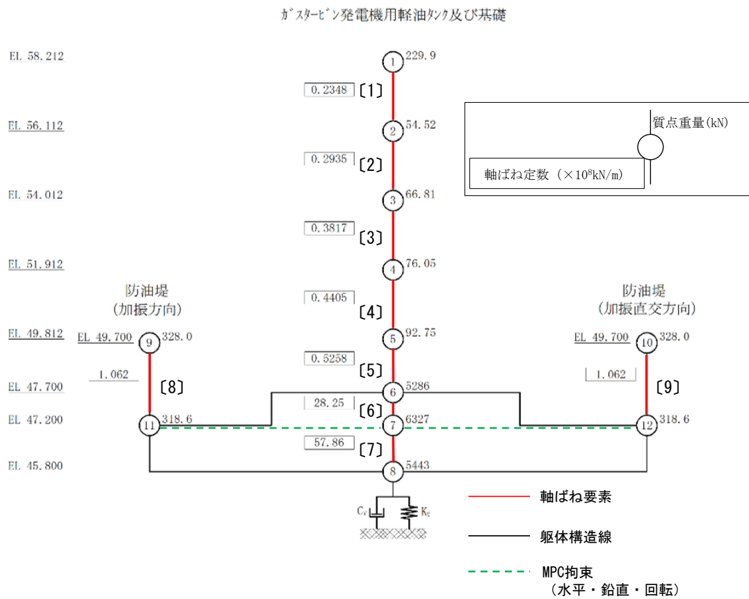
図 3-9 地震応答解析モデル (鉛直方向)
