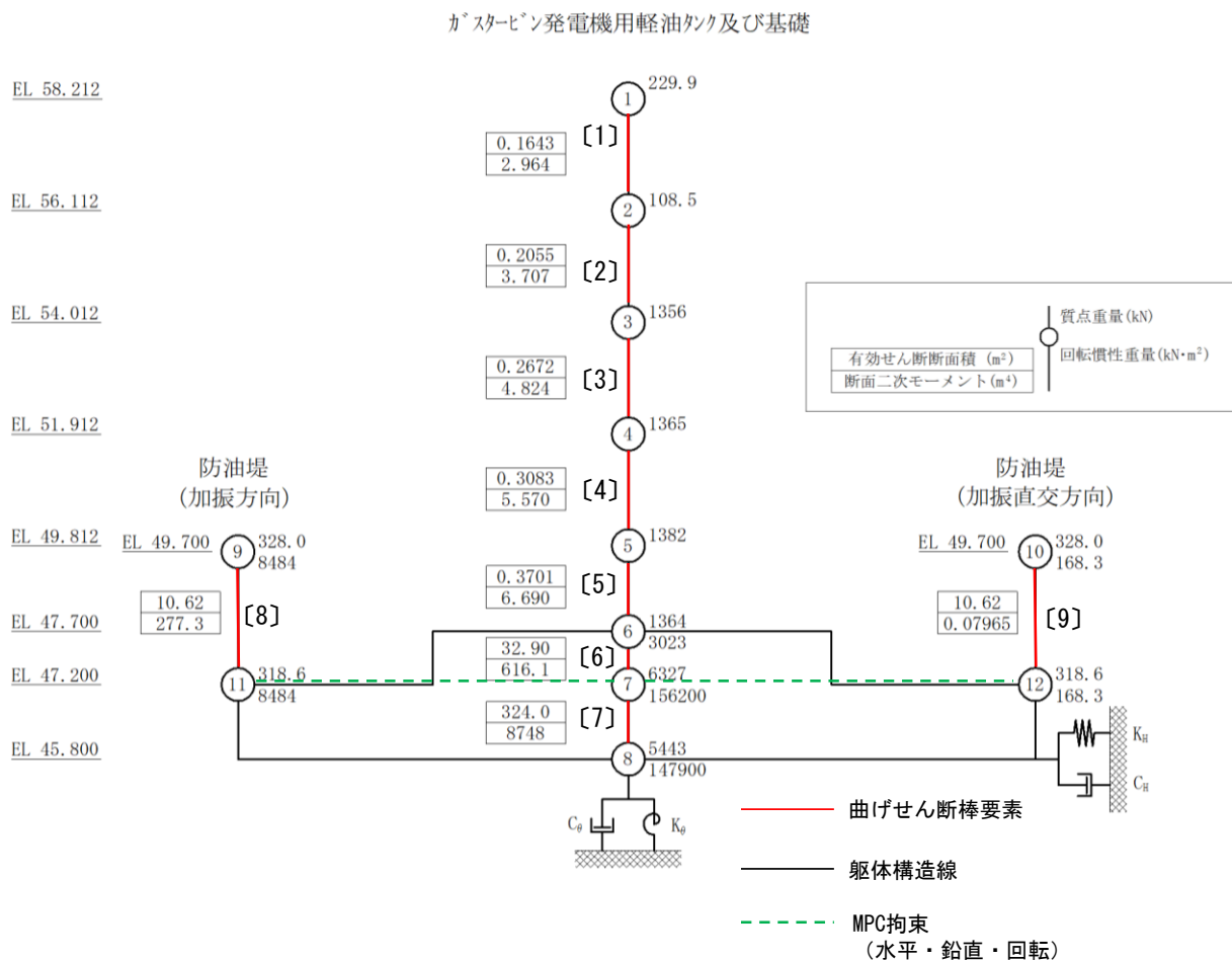
図3-5 地震応答解析モデル（水平方向）
