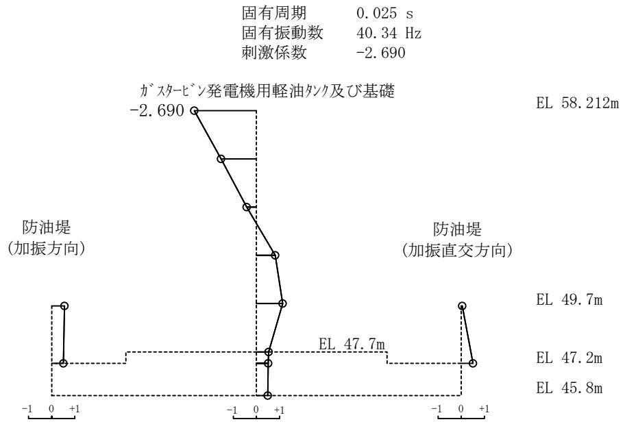
図 3-10(3) 刺激関数図 (解析ケース①, 水平方向, 3次モード)
