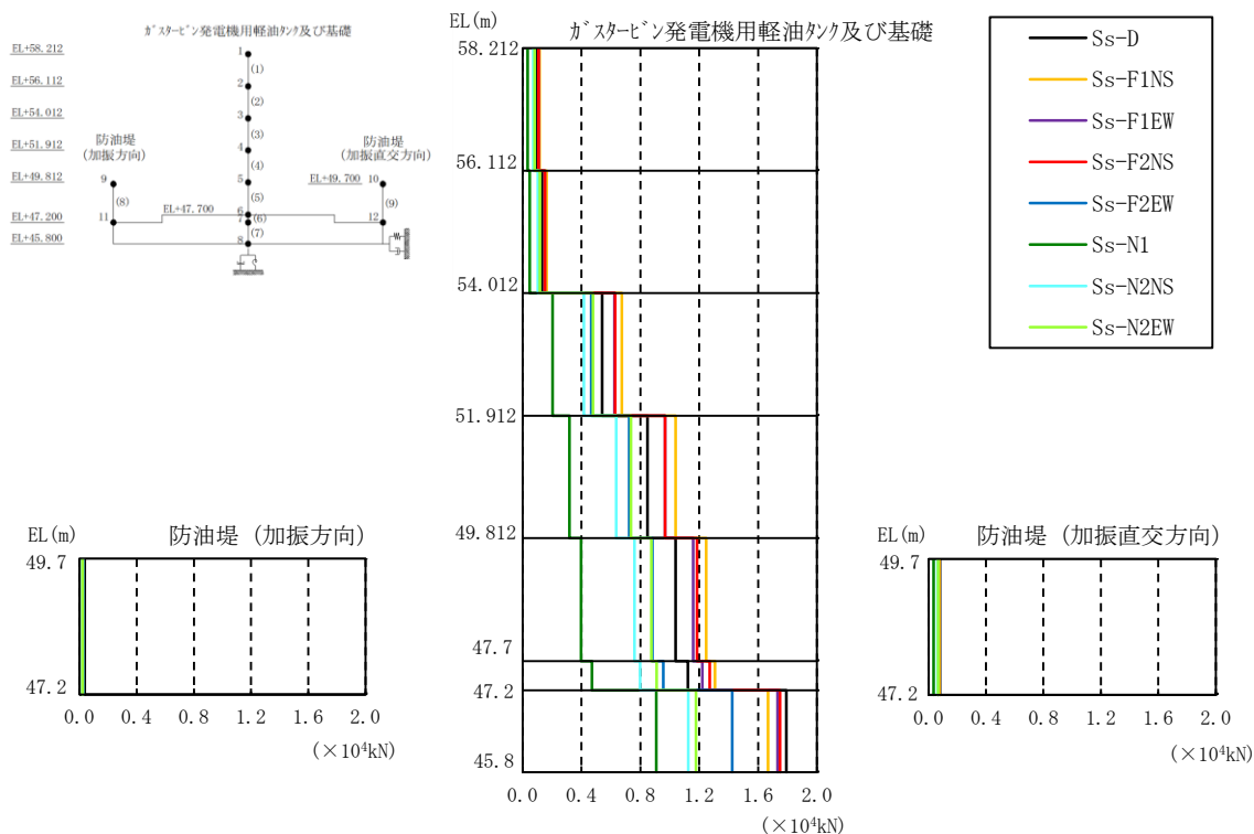
図 3-71 最大応答せん断力（解析ケース③）
