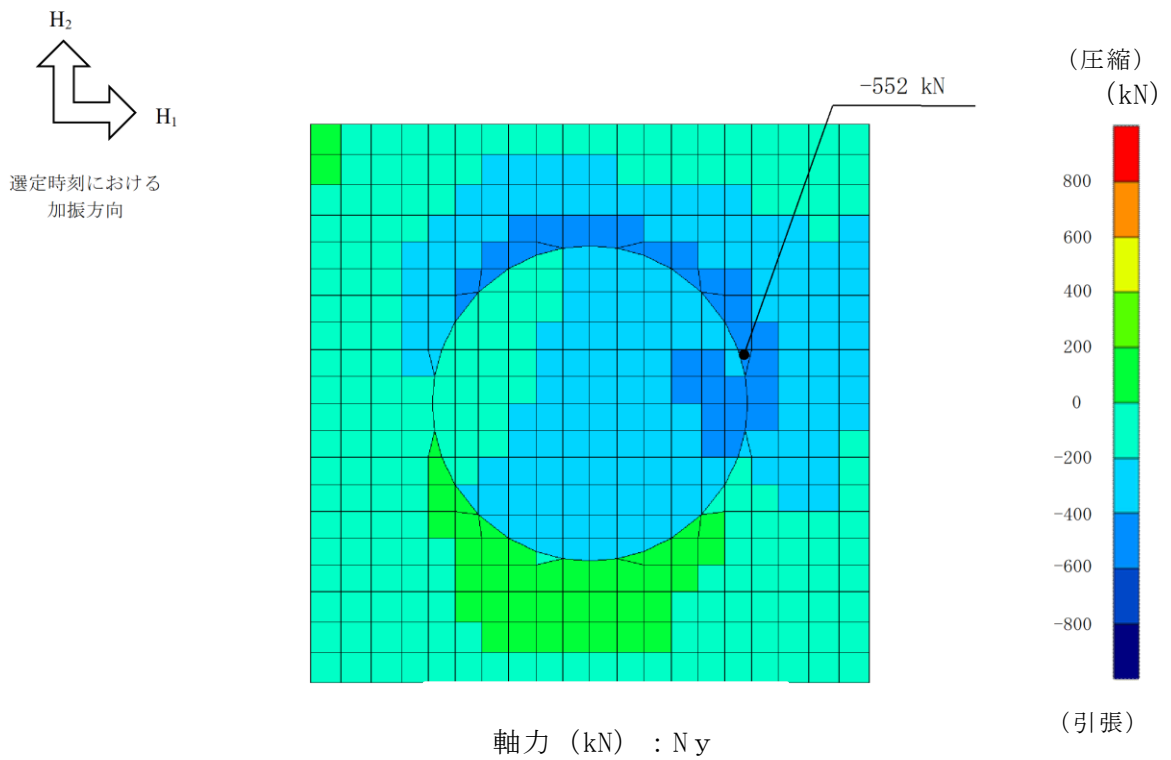
図 6-2 照査時刻における断面力図 (解析ケース①, S_s - N_2 (EW), 26.780 秒)
