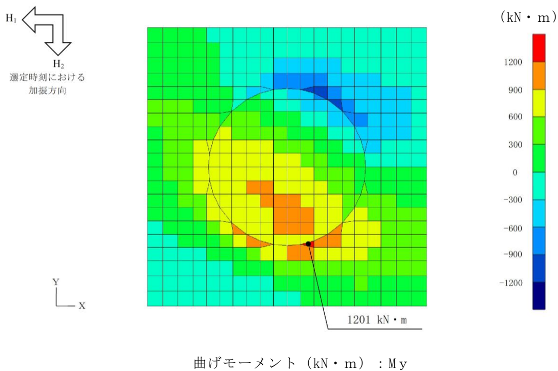
図 6-4 曲げ・軸力系の破壊に対する断面力分布図 (解析ケース③, S_s - D , t = 15.268\text{s} )
