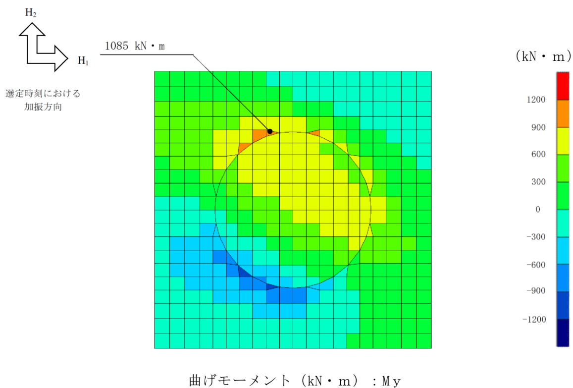
図 6-1 照査時刻における断面力図 (解析ケース①, S_s - N2 (EW), 26.780 秒)
