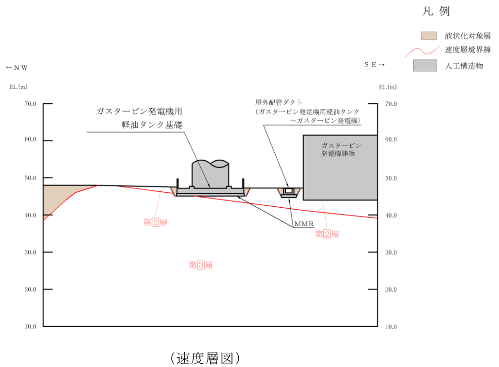
図 2-6 ガスタービン発電機用軽油タンク基礎 地質断面図 (B-B断面)
