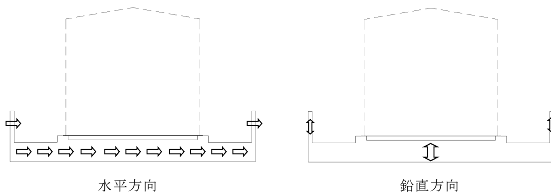
図4-4 躯体に作用する慣性力の作用概念図
