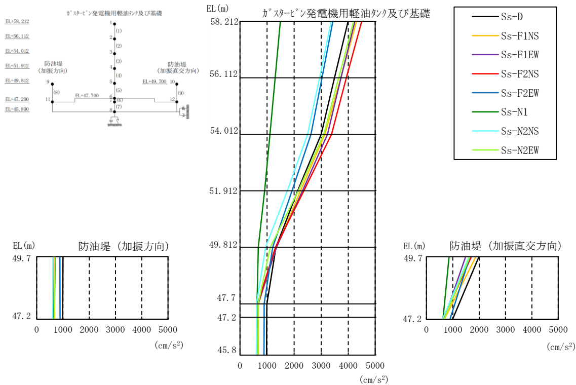
図 3-53 最大応答加速度（水平方向，解析ケース①）
