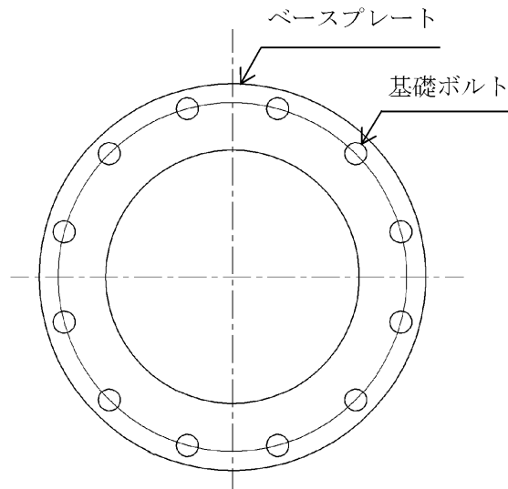
図4-5 基礎ボルトの配置の概念図
