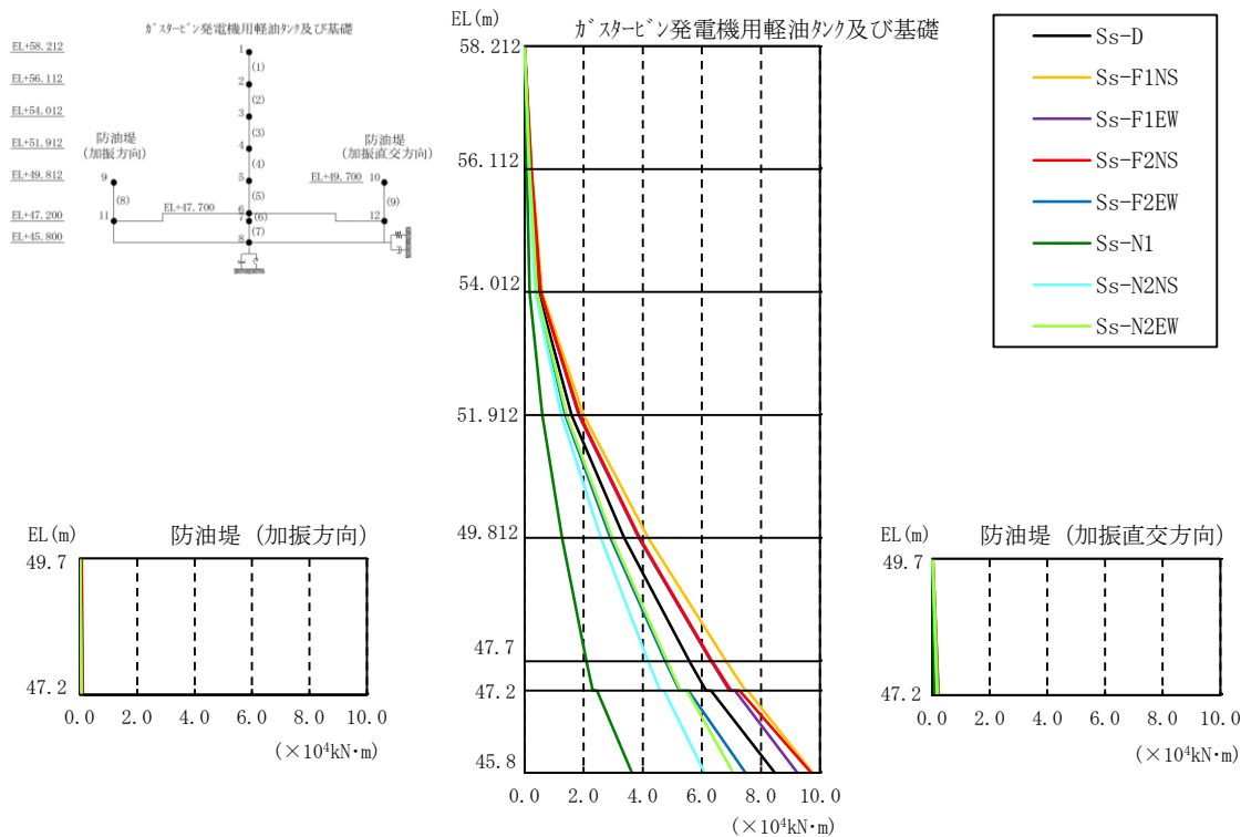
図 3-72 最大応答曲げモーメント（解析ケース③）
