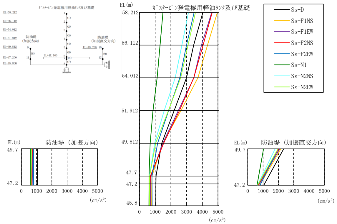
図 3-67 最大応答加速度（水平方向，解析ケース③）
