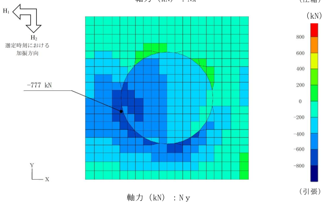
図 6-5 曲げ・軸力系の破壊に対する断面力分布図 (解析ケース③, S_s - D , t = 15.268s )
