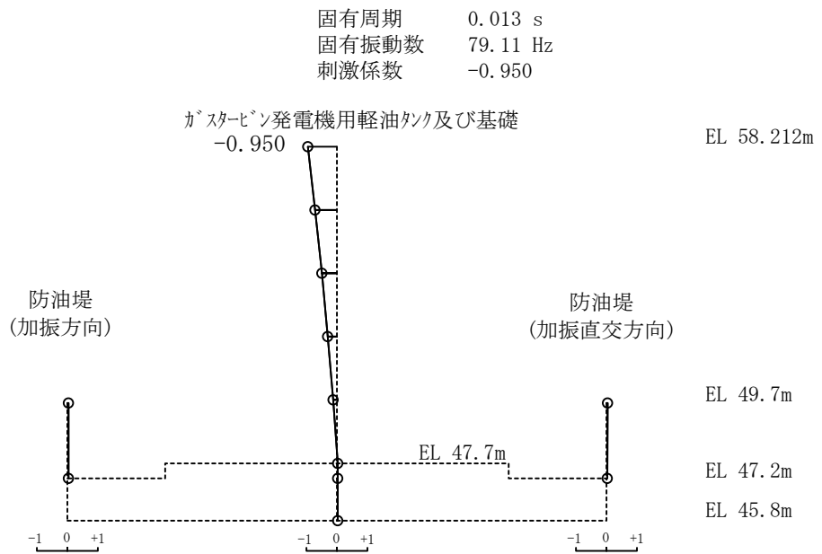
図 3-11(2) 刺激関数図 (解析ケース①, 鉛直方向, 2次モード)
