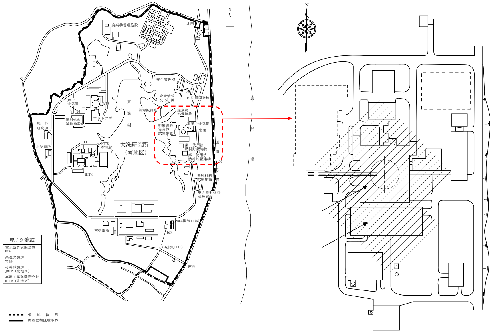
第 1 図 影響評価対象施設の配置
