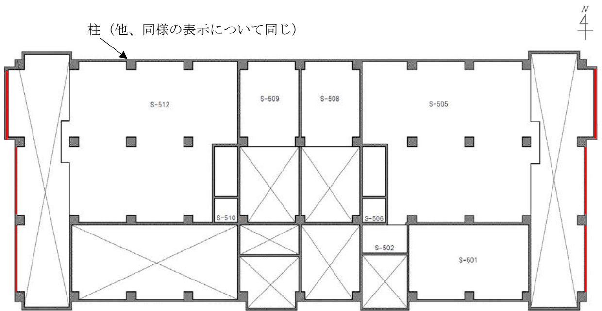
第5図 主冷却機建物の外壁のうち、貫通防止対策を実施する範囲の概略図 (2F 平面図)
