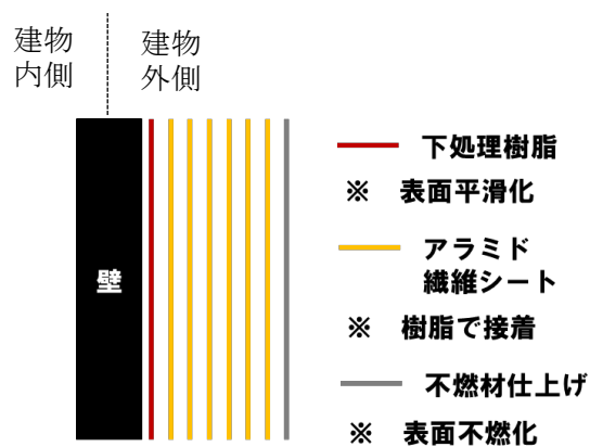
第14図 貫通防止用アラミド繊維シートのイメージ
