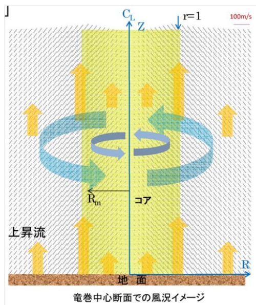
第 1.2 図 ランキン渦モデルの風況場イメージ
