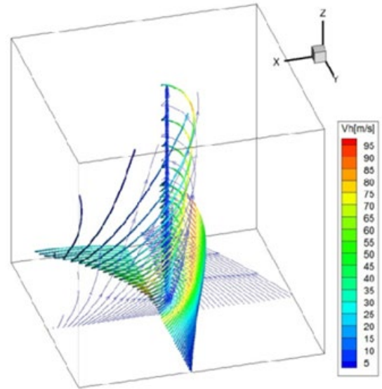
第 2.2 図 ランキン渦モデルの風速場
