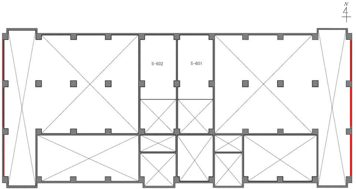
第 6 図 主冷却機建物の外壁のうち、貫通防止対策を実施する範囲の概略図（3F 平面図）
