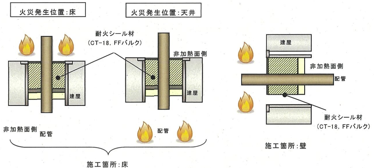
図4 試験概要図
