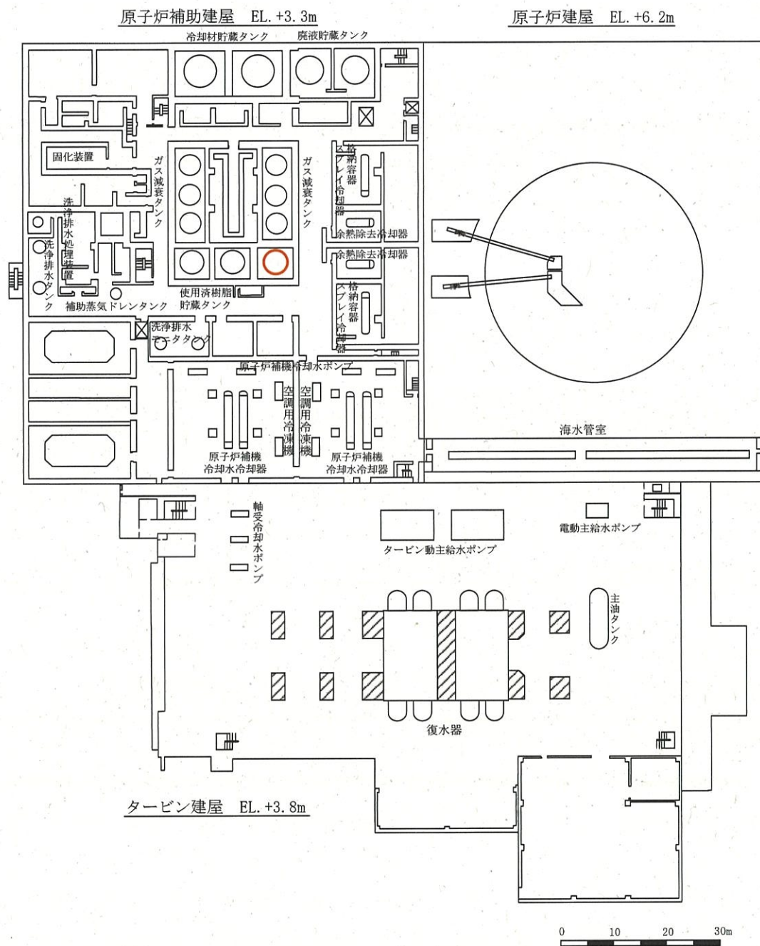
第29-2-1図 主要建屋平面図（地下1階） ( ○ : 使用済樹脂貯蔵タンク【増設】 )
