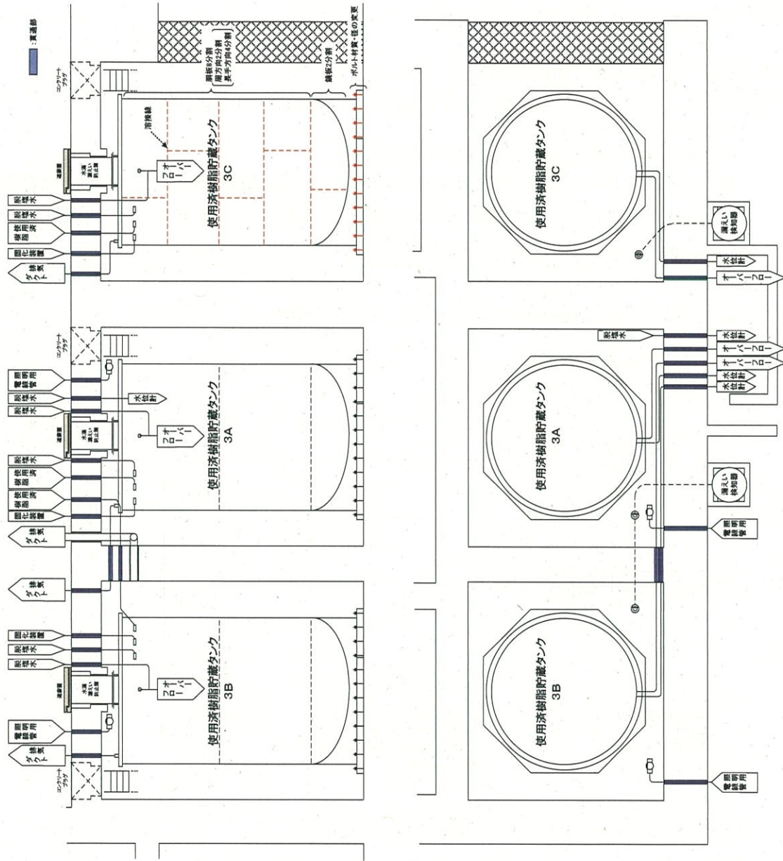
図 3-2 使用済樹脂貯蔵タンクおよび周辺状況 (増設後)
