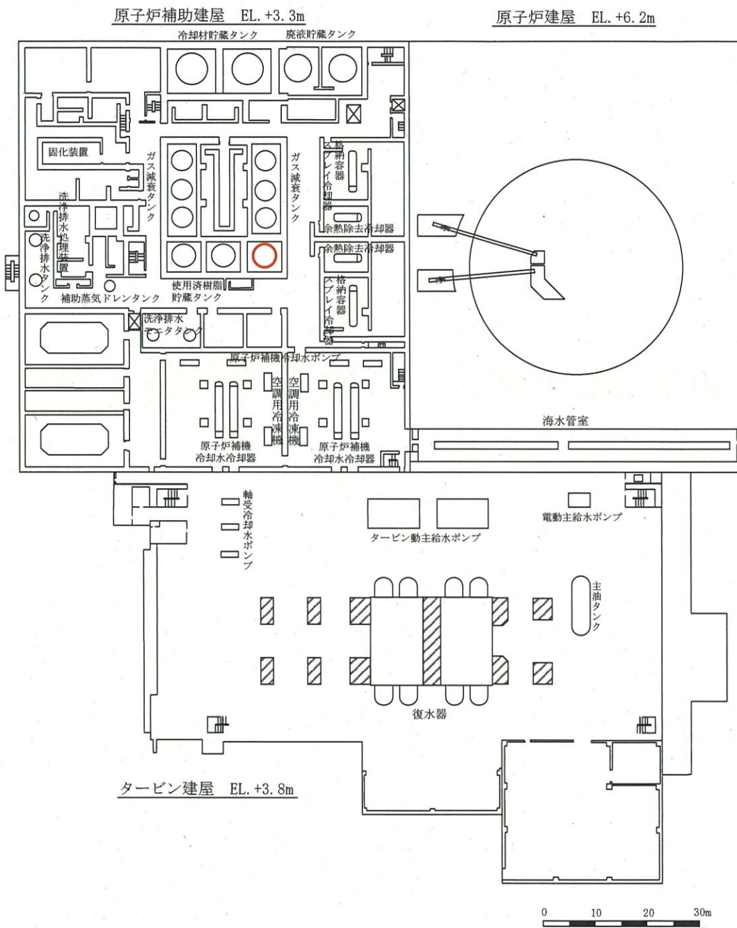
第29-2-1図 主要建屋平面図（地下1階）
