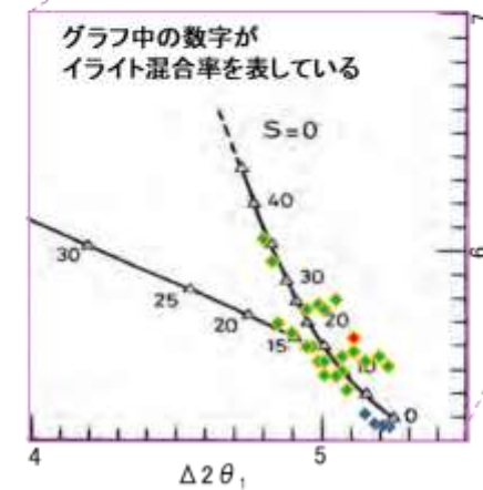
EG処理スメクタイトのピーク回折角
