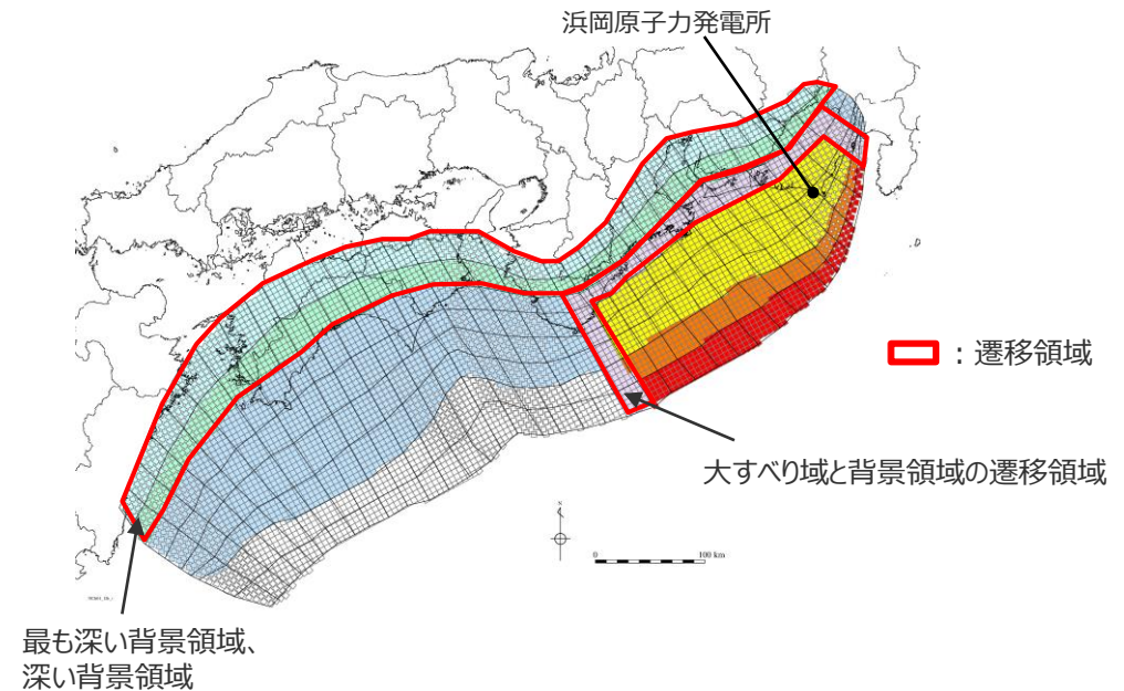
検討波源モデルA
