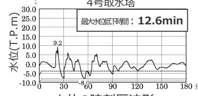
水位の時刻歴波形・期望平均干潮位 T.P.-0.93mを考慮
