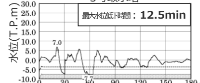
最大下降水位分布 敷地前面
