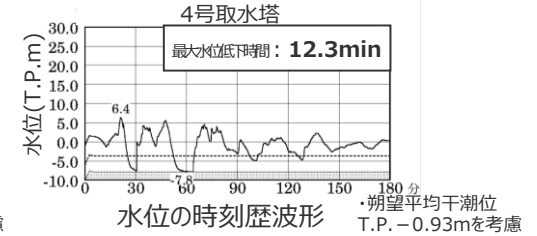
最大下降水位(T.P.m)(水位低下時間)
