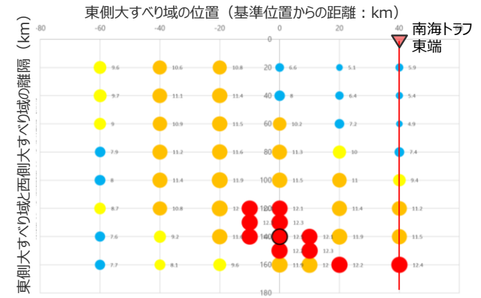
検討波源モデルD 大すべり域 2つのケース
