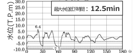
最大下降水位分布 敷地前面
