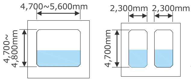
1連部 2連部 5号放水路標準断面図
