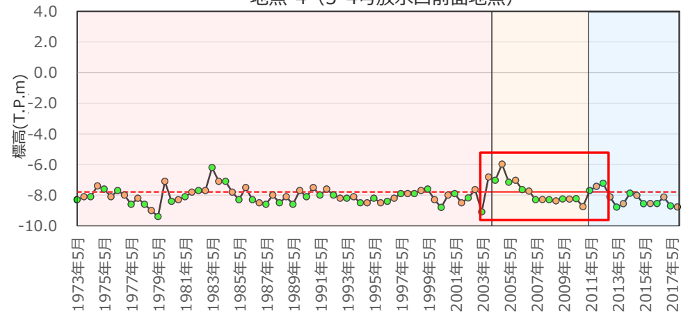
地点-8（3・4号放水口前面より約500m沖合地点）
