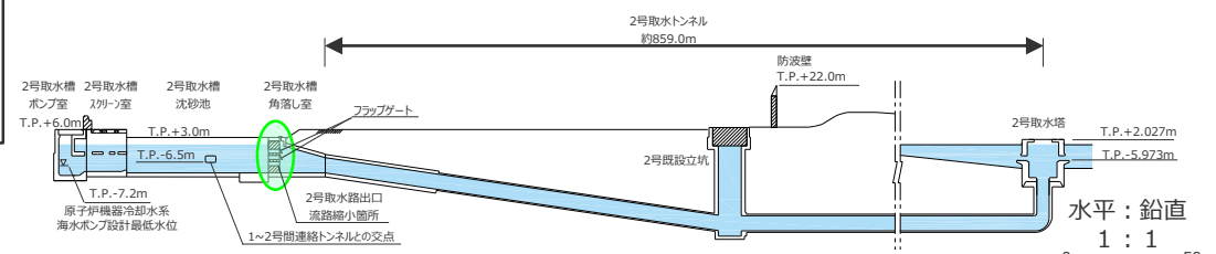
2号取水塔～2号取水トンネル～2号取水槽縦断面図
