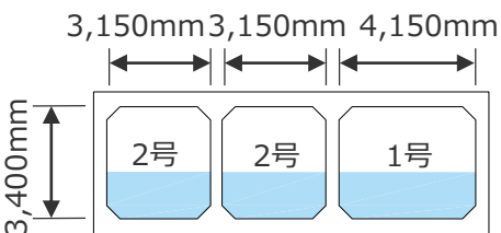
1,2号放水路標準断面図
