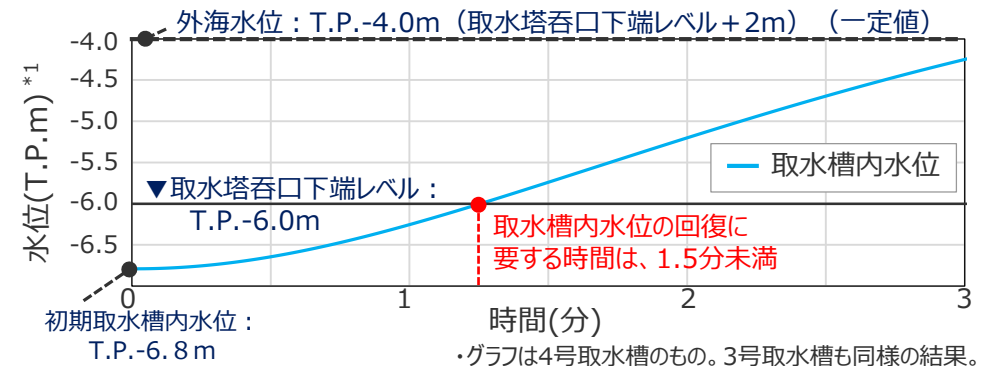
管路解析による取水槽内水位の時間変化
