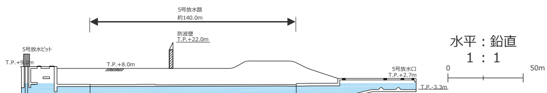
5号放水口～5号放水路～5号放水ピット縦断面図
