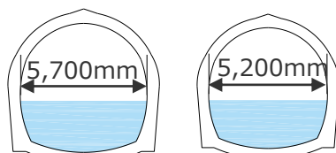
3号 4号 3,4号放水路標準断面図
