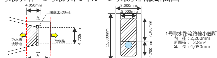
1号取水塔～1号取水トンネル～1号取水槽縦断面図
