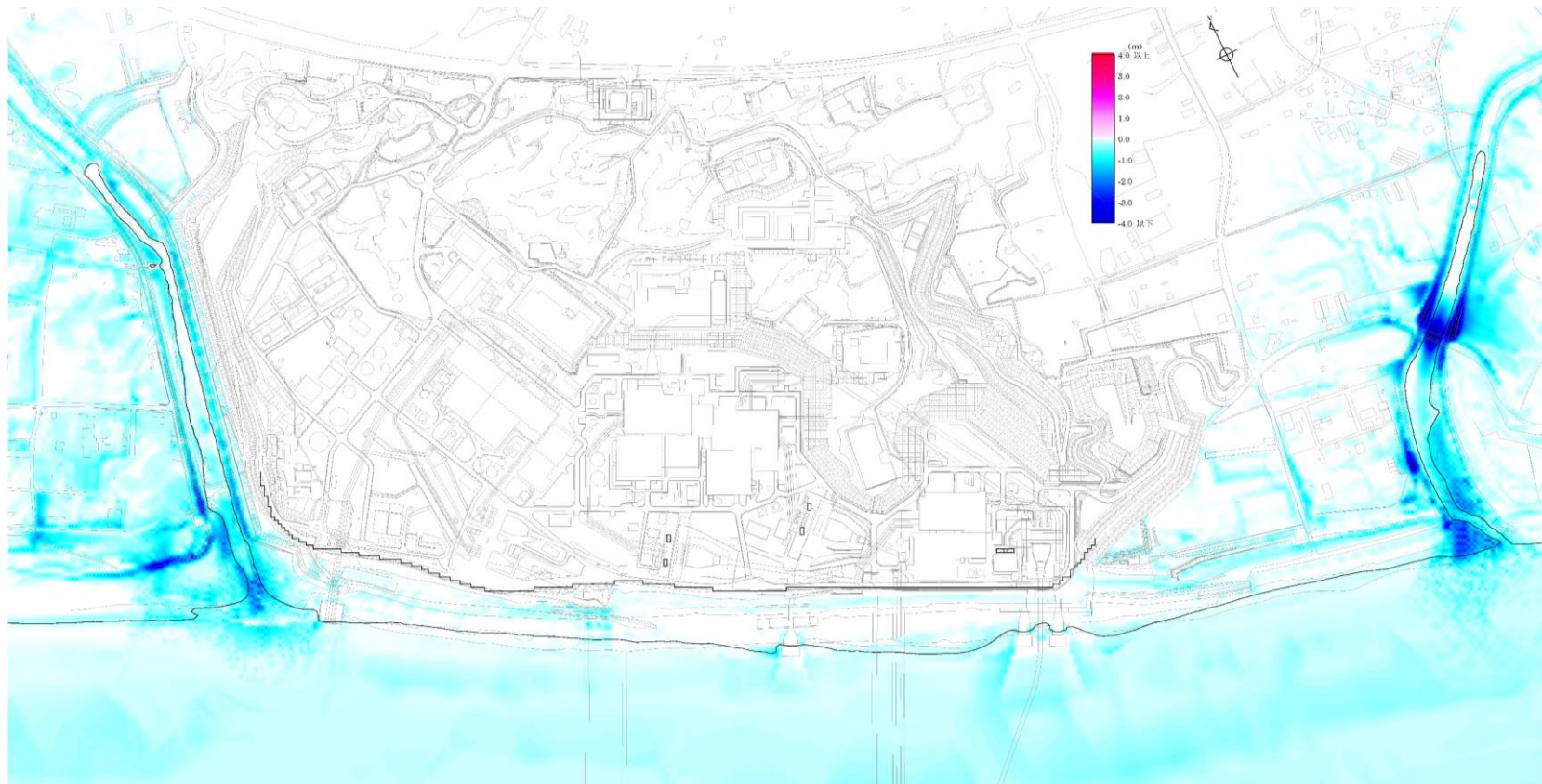
内閣府の最大クラスモデル（ケース①）による地震発生から6時間後までの最大洗掘量分布
