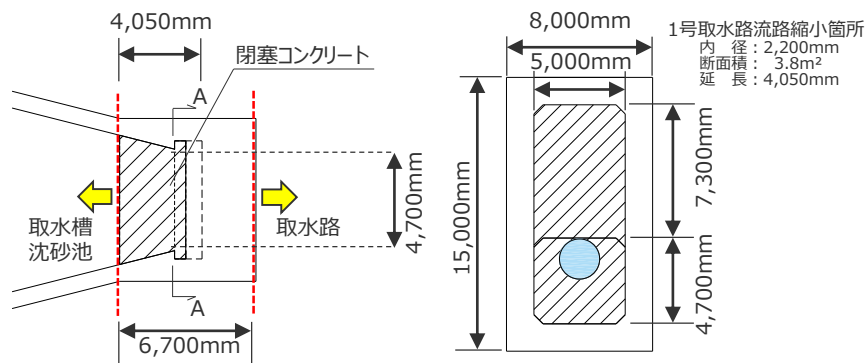
1号取水路出口流路縮小箇所 平面図・A-A断面図
