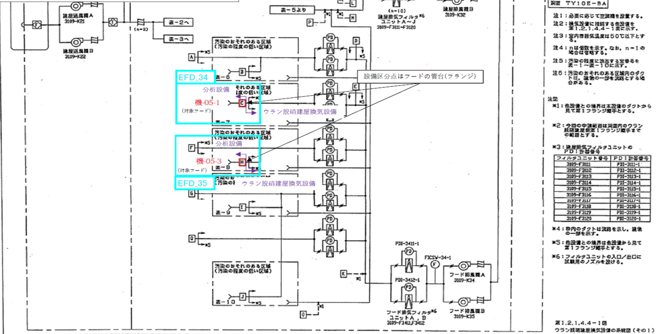
第3-14図 分析設備（ウラン脱硝建屋）系統概要図(放射性物質を保持する系統の負圧維持)
