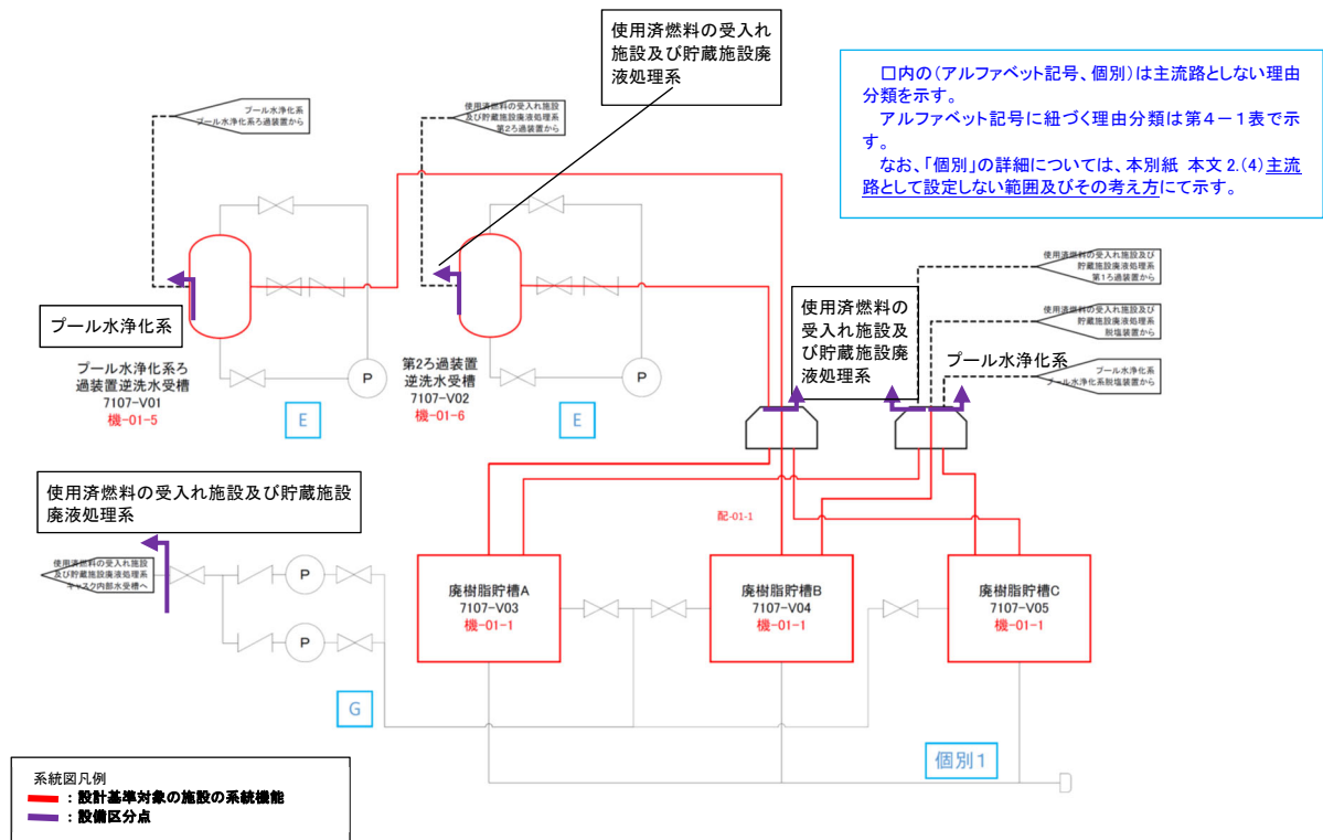
第 4 - 1 図 廃樹脂貯蔵系（使用済燃料受入れ・貯蔵建屋）に係る主流路の範囲及び主流路として設定しない範囲の概要図
