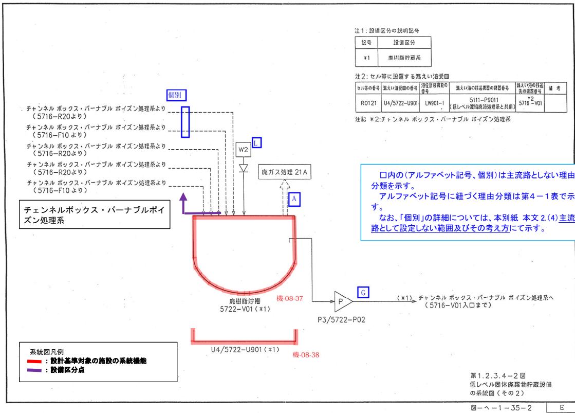
第4-3図 廃樹脂貯蔵系（チャンネルボックス・バーナブルポイズン処理建屋）に係る主流路の範囲及び主流路として設定しない範囲の概要図
