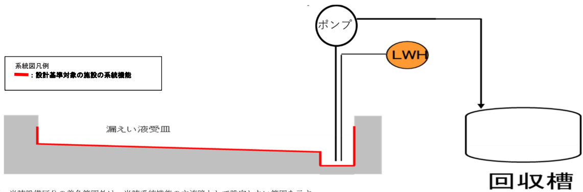
第2-4図 低レベル廃液の漏えい液の保持（漏えいした溶液の保持）
