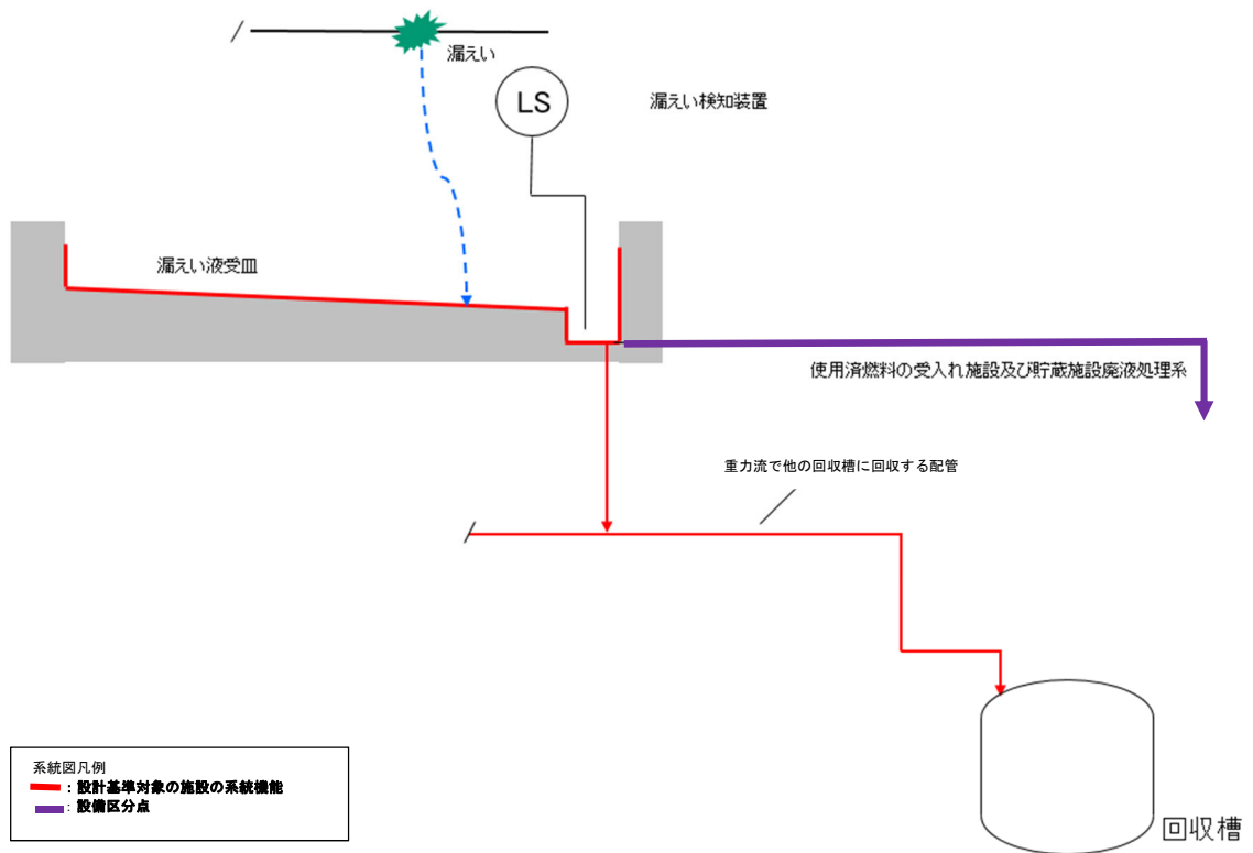
第2-5図 低レベル廃液の漏えい液の保持（漏えいした溶液の保持、重力流による回収）
