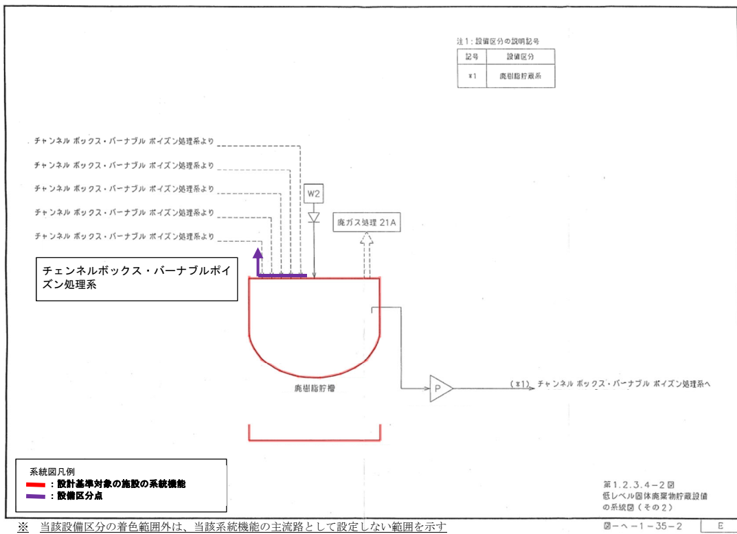
第 2 - 3 図 廃樹脂貯蔵系（チャンネルボックス・バーナブルポイズン処理建屋）系統図
