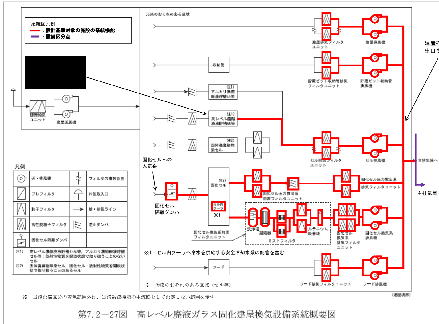
第2-1図 高レベル廃液ガラス固化建屋換気設備 系統概要図 (放射性物質の保持機能) (事業変更許可申請書 添付書類六 第7.2-27図抜粋)
