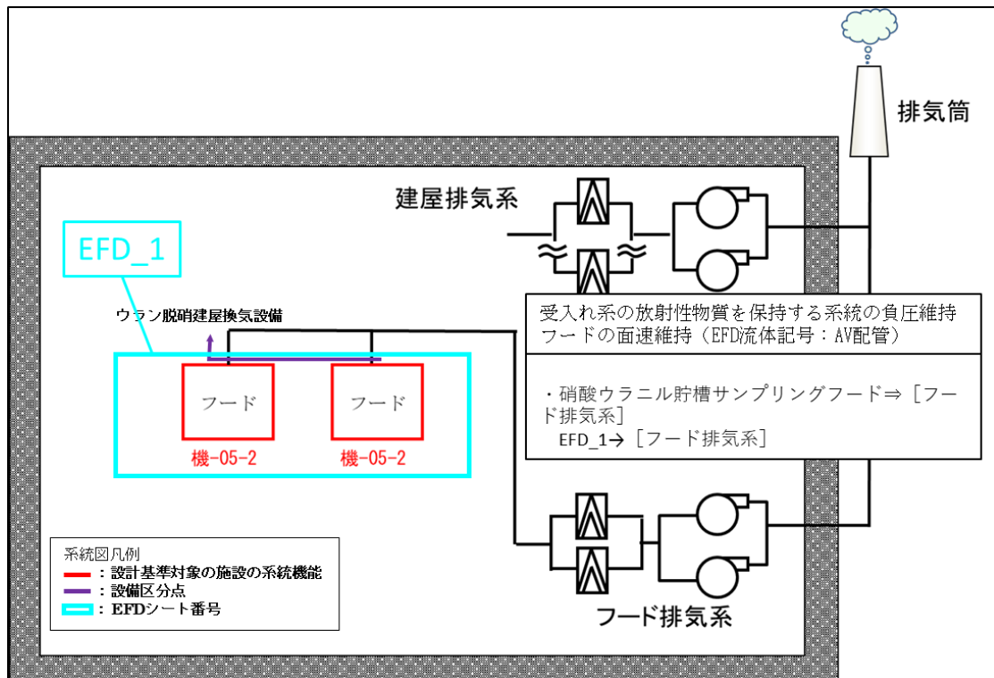
第3-3図 受入れ系 フード図
