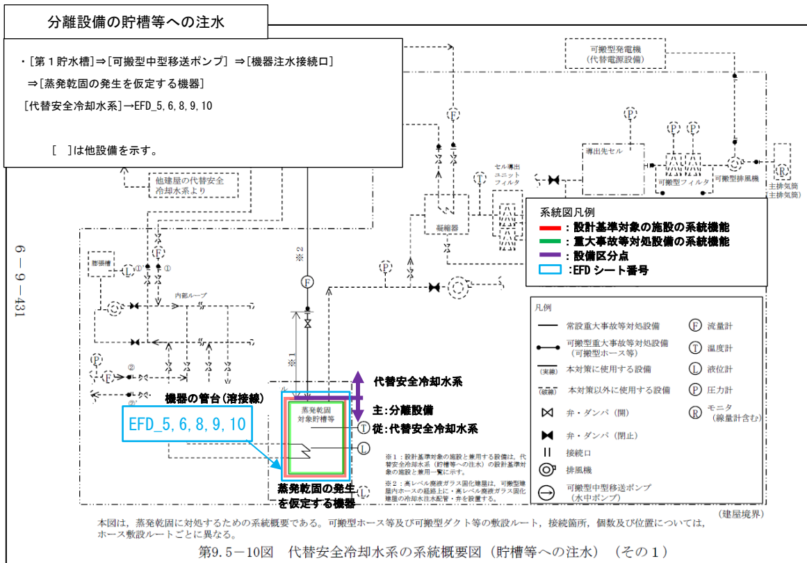
第3-10図（1） 代替安全冷却水系 系統概要図（貯槽等への注水） （兼用配管を含まない場合） （事業変更許可申請書 添付書類六 第9.5-10図抜粋）
