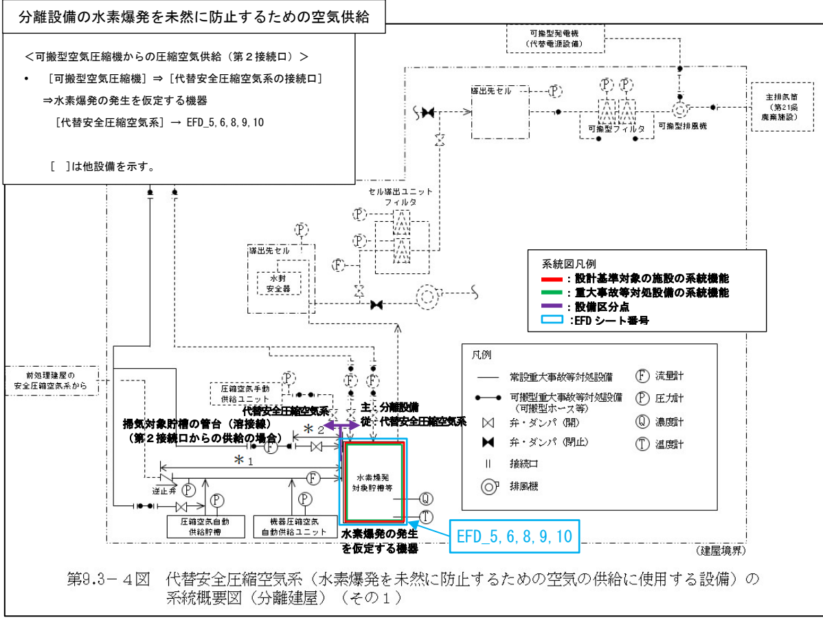
* 1 : 水素掃気配管・弁、* 2 : 機器圧縮空気供給配管・弁 第 3 - 15 図 代替安全圧縮空気系（水素爆発を未然に防止するための空気供給に使用する設備）の系統概要図（兼用配管を含まない場合） （事業変更許可申付書類六 第9. 3-7図抜粋）
