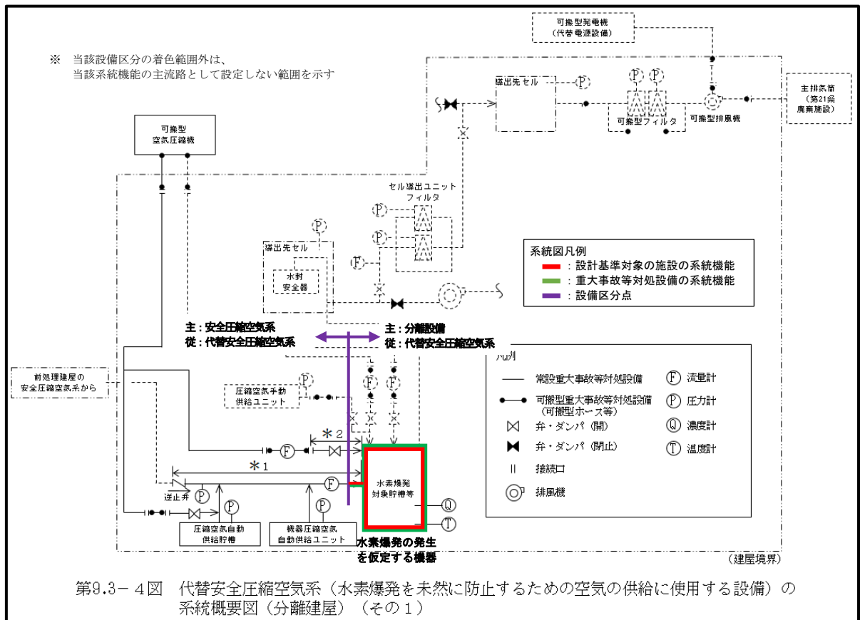
第2-16図 代替安全圧縮空気系 (水素爆発を未然に防止するための空気供給に使用する設備) の系統概要図 (兼用配管を含む場合) (事業変更許可申付書類六 第9.3-4図抜粋)
