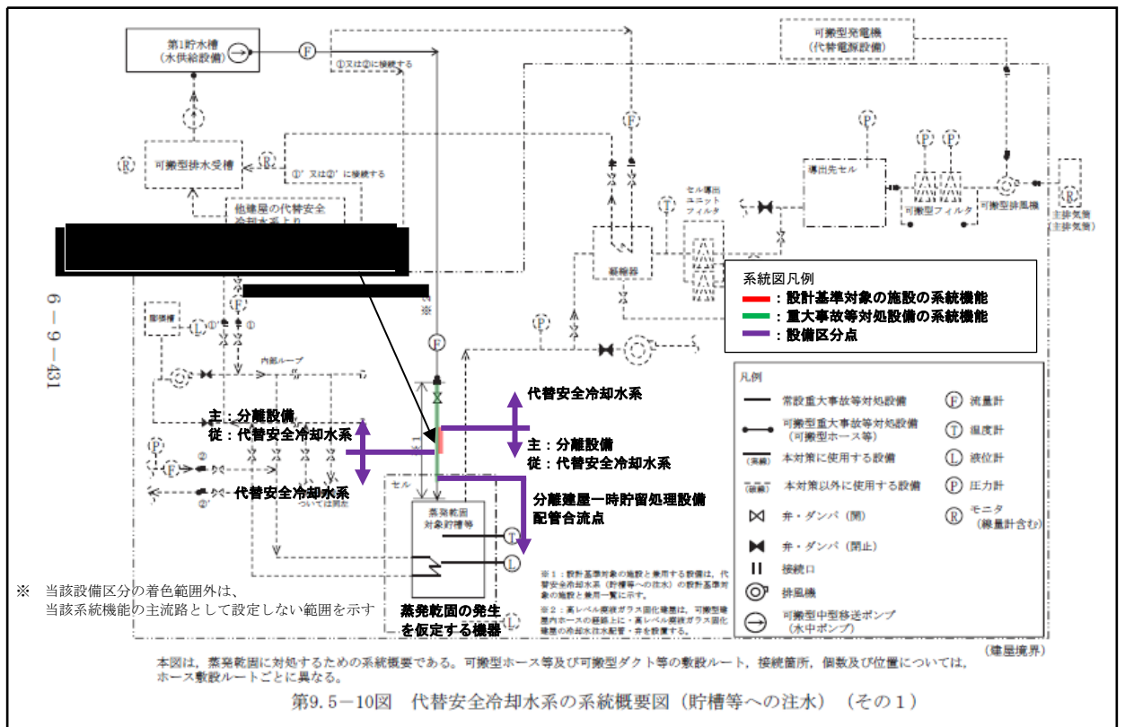
第2-12図 代替安全冷却水系 系統概要図(貯槽等への注水) (兼用配管を含む場合) (計装用空気ライン以外からの貯槽等への注水その1) (事業変更許可申請書 添付書類六 第9.5-10図抜粋)
