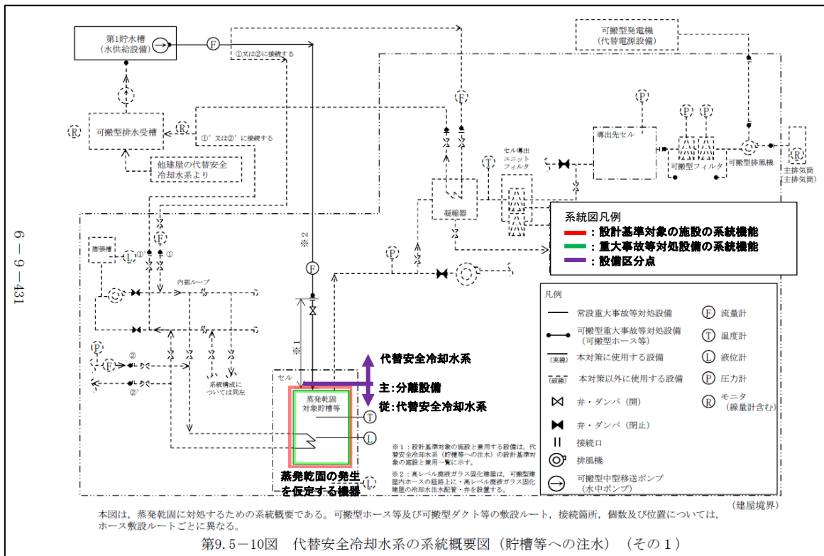
第2-11図 代替安全冷却水系 系統概要図 (貯槽等への注水)
