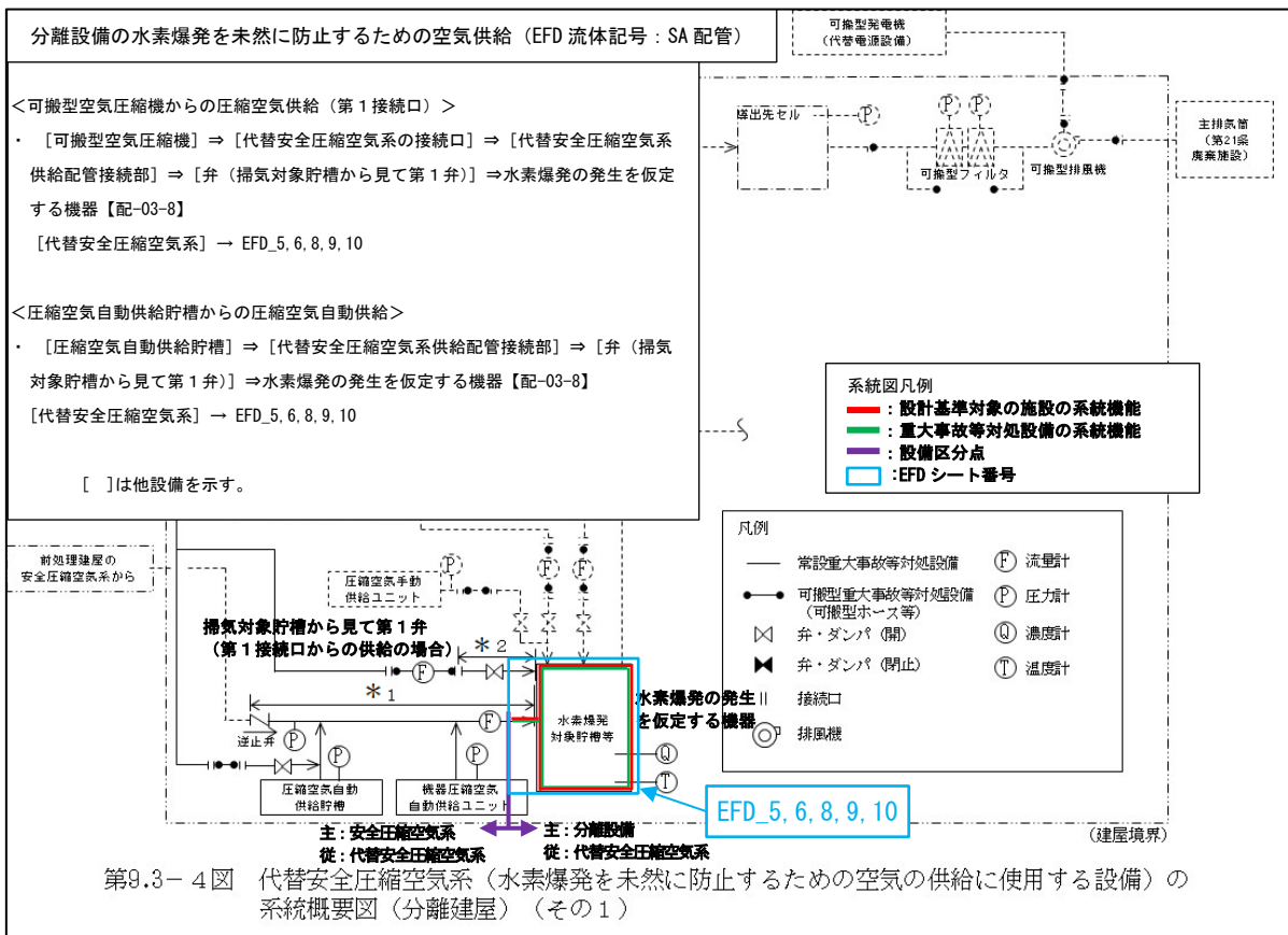
* 1 : 水素掃気配管・弁、* 2 : 機器圧縮空気供給配管・弁 第 3 - 14 図 代替安全圧縮空気系 (水素爆発を未然に防止するための空気供給に使用する設備) の系統概要図 (兼用配管を含む場合) (事業変更許可申付書類六 第9. 3-7図抜粋)
