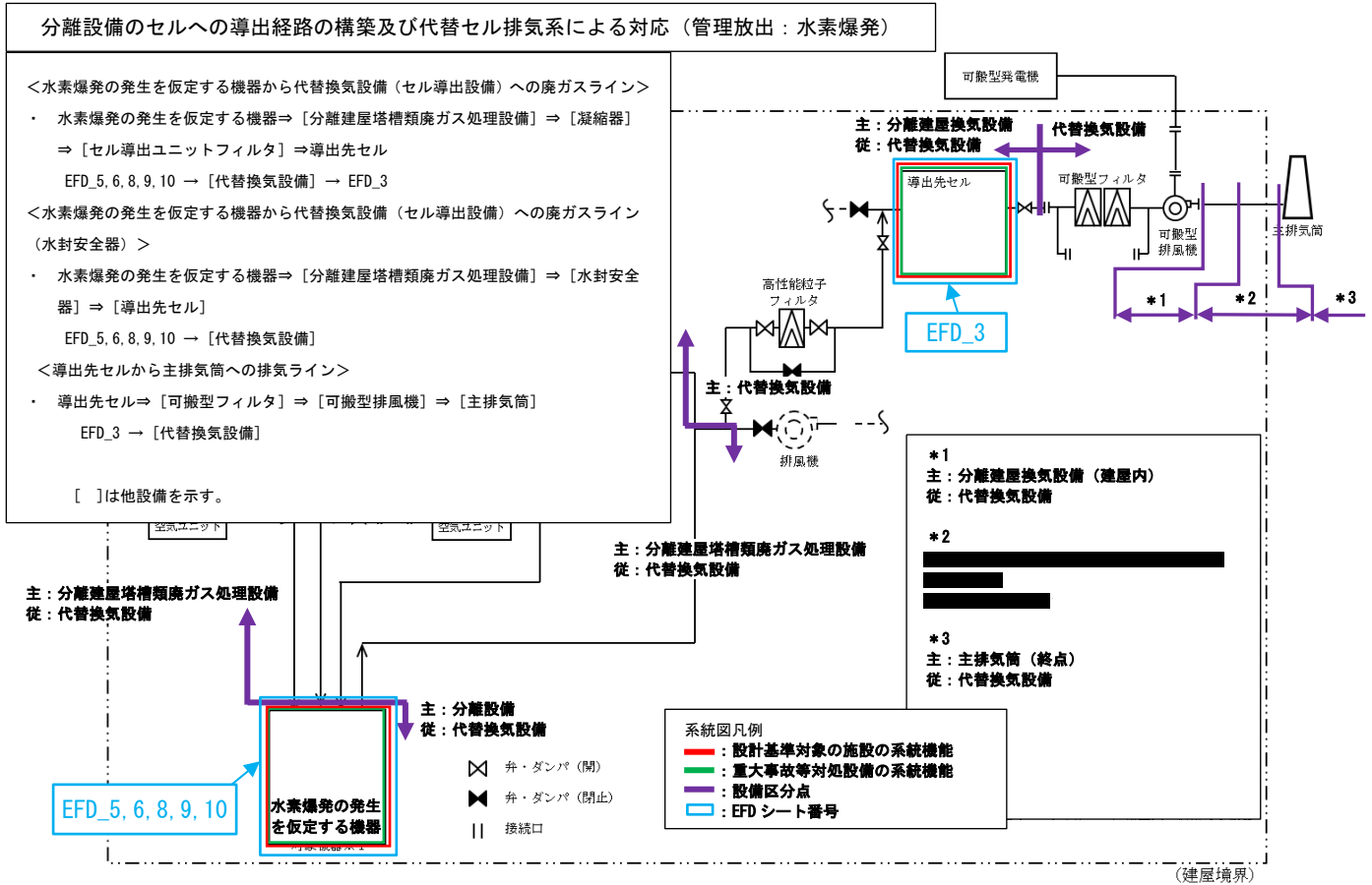
第3-17図 代替換気設備 系統概要図
