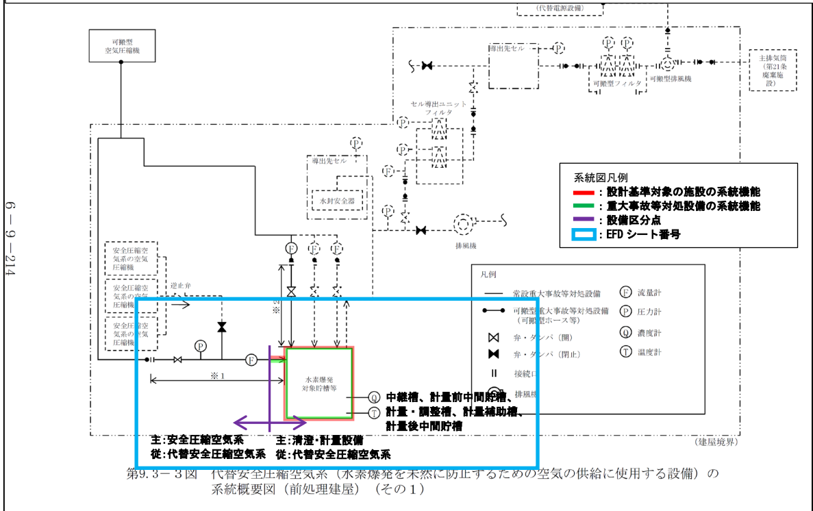
第3-10(1)図 代替圧縮空気系の系統概要図
