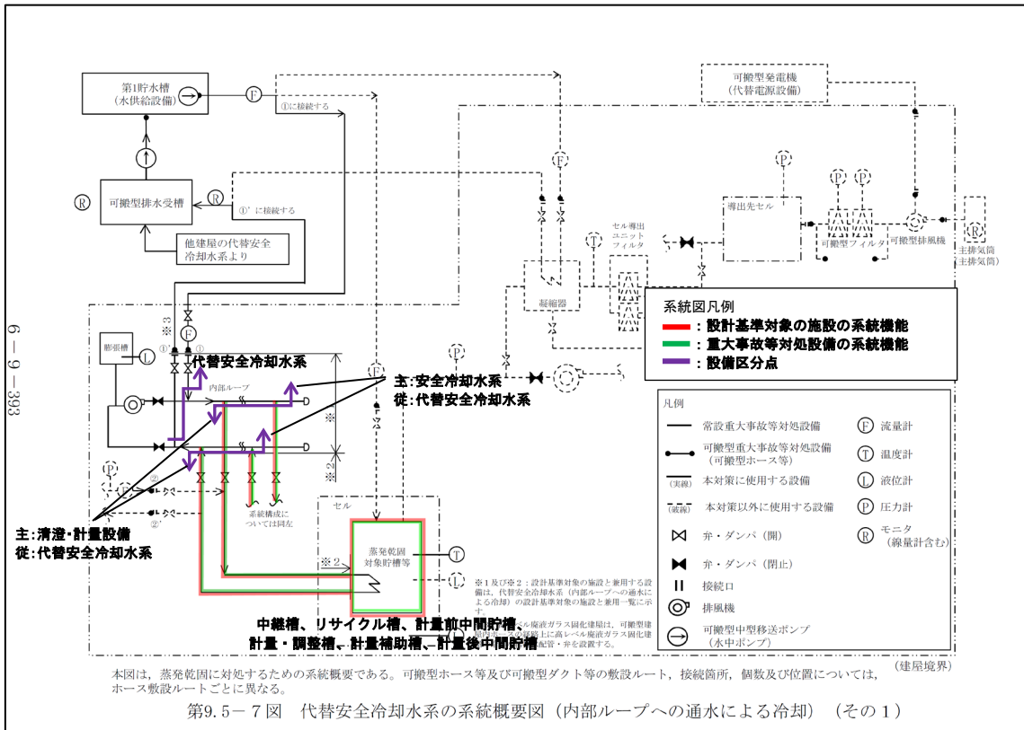
第2-6図 代替安全冷却水系 系統概要図 (内部ループへの通水による冷却) (事業変更許可申請書 添付書類六 第9.5-7図抜粋)
