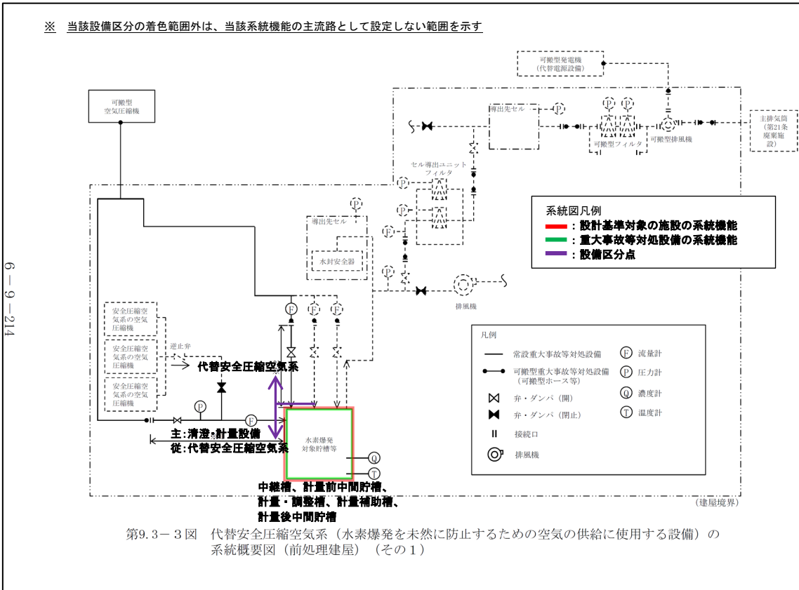
第2-10(1)図 代替安全圧縮空気系の系統概要図
