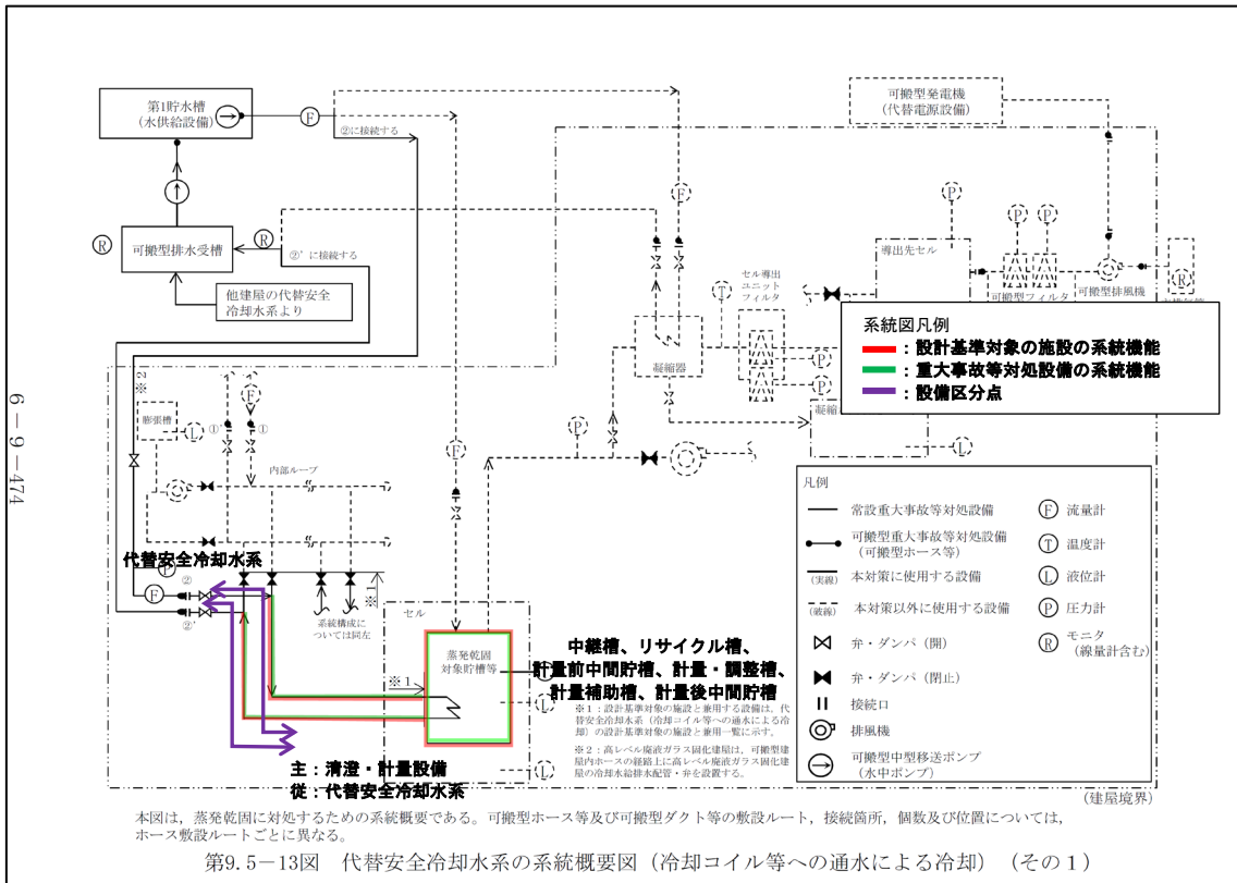
第2-8図 代替安全冷却水 系統概要図 (冷却コイル等への通水による冷却) (事業変更許可申請書 添付書類六 第9.5-13図抜粋)
