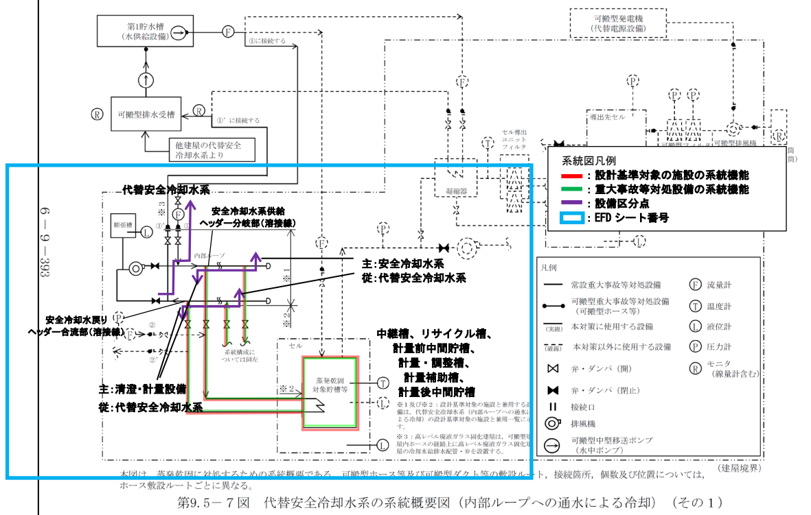
第3-5図 代替安全冷却水系 系統概要図 (内部ループ通水)
