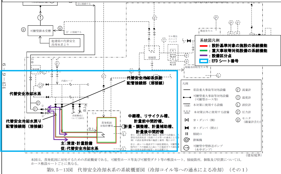
第3-8図 代替安全冷却水 系統概要図 (冷却コイル等への通水による冷却) (事業変更許可申請書 添付書類六 第9.5-13図抜粋)
