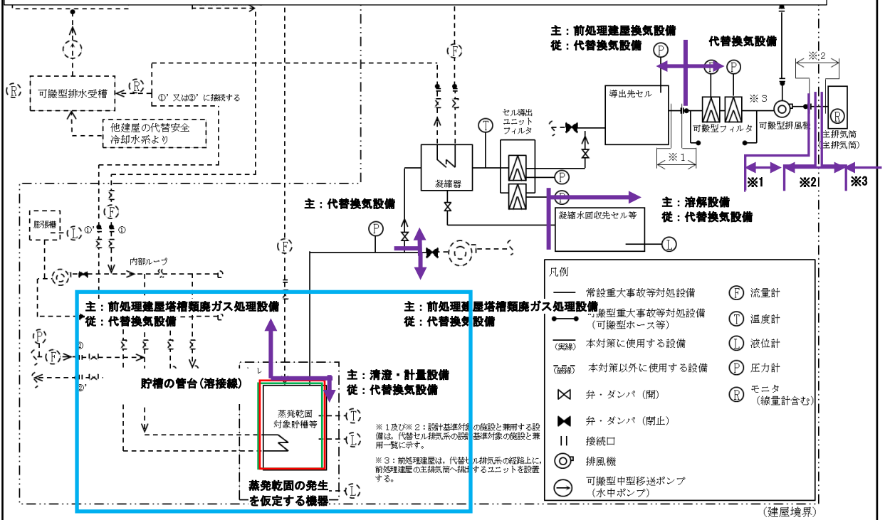
第7.2-38図(1) 代替セル排気系の系統概要図 (その1)
