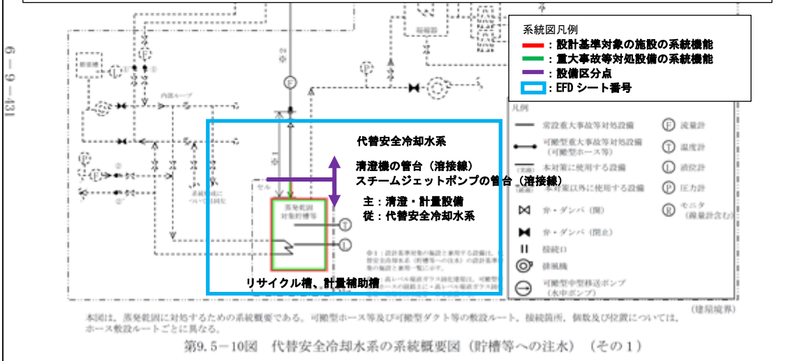
第3-6(2)図 代替安全冷却水系 系統概要図 (計装用空気ライン以外からの貯槽等への注水) (兼用配管を含む場合) (事業変更許可申請書 添付書類六 第9.5-10図抜粋)
