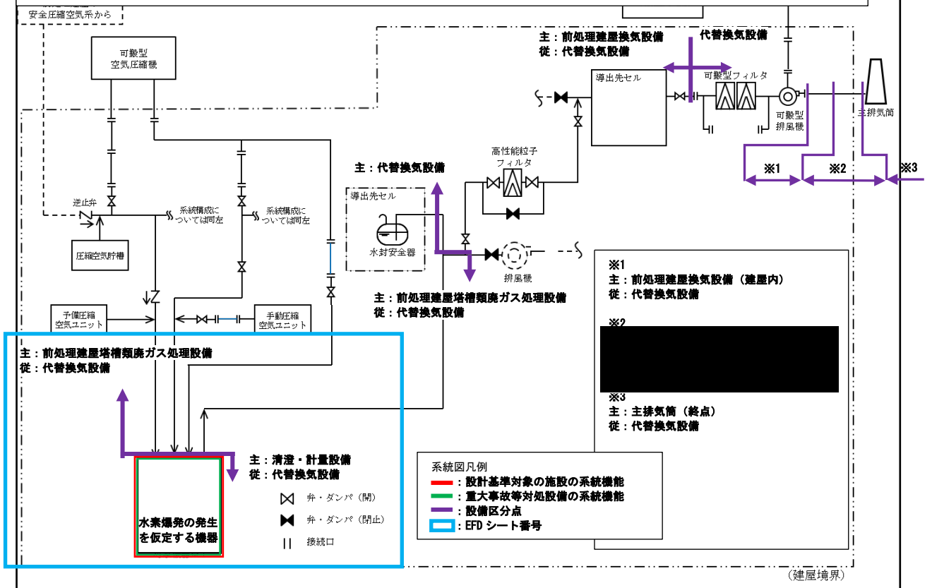
第 3-13 図 代替換気設備 系統概要図
