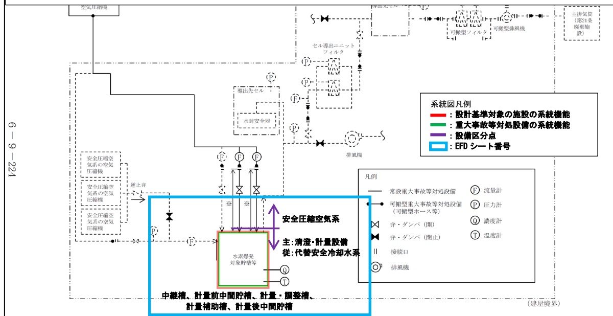
第9.3-8図 代替安全圧縮空気系 (水素爆発の再発を防止するための空気の供給に使用する設備) の系統概要図 (前処理建屋) (その1)
