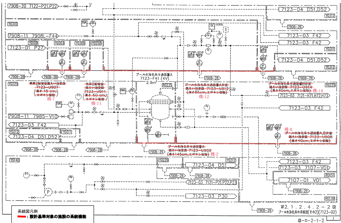
第3-2図 プール水浄化系 系統図(室等の漏えい拡大防止)(2/5)
