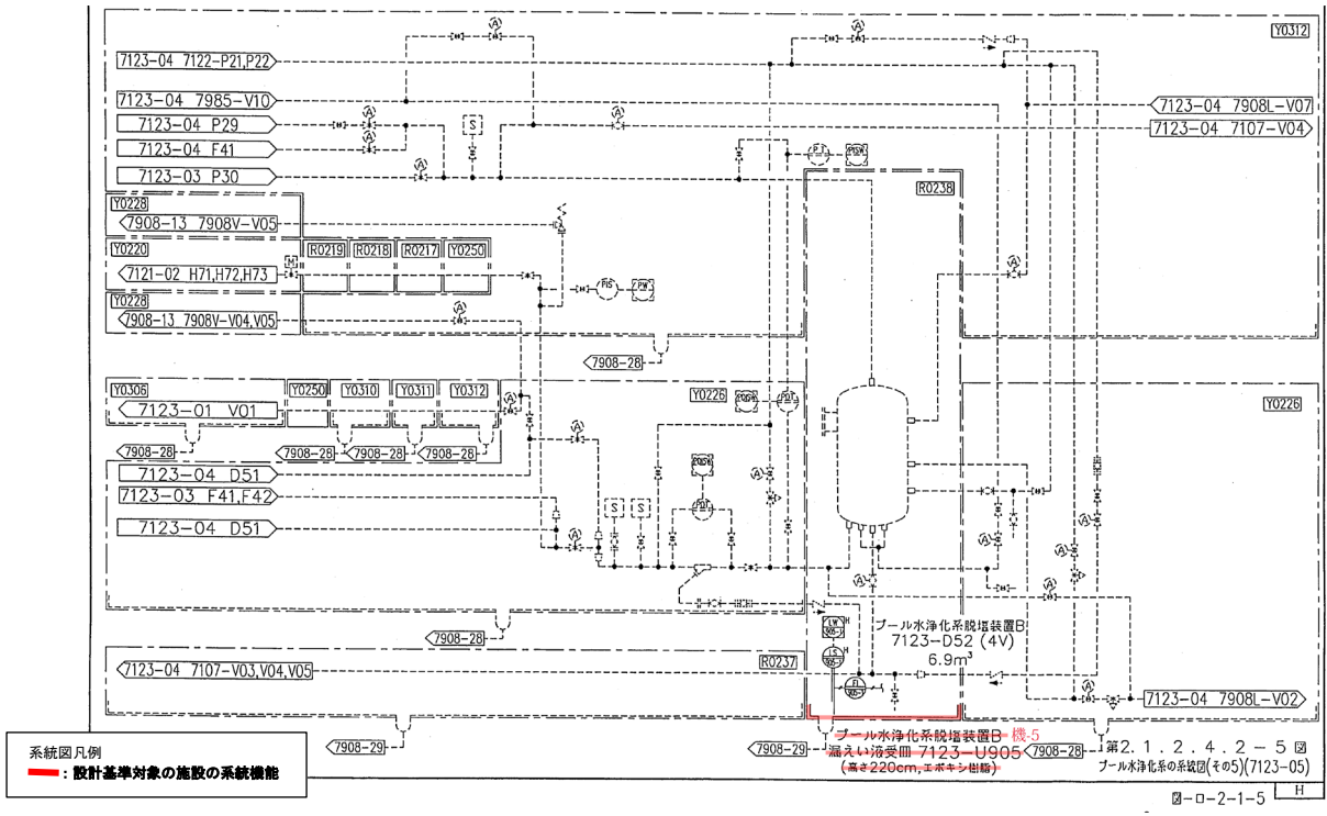
第3-2図 プール水浄化系 系統図 (室等の漏えい拡大防止) (5/5)
