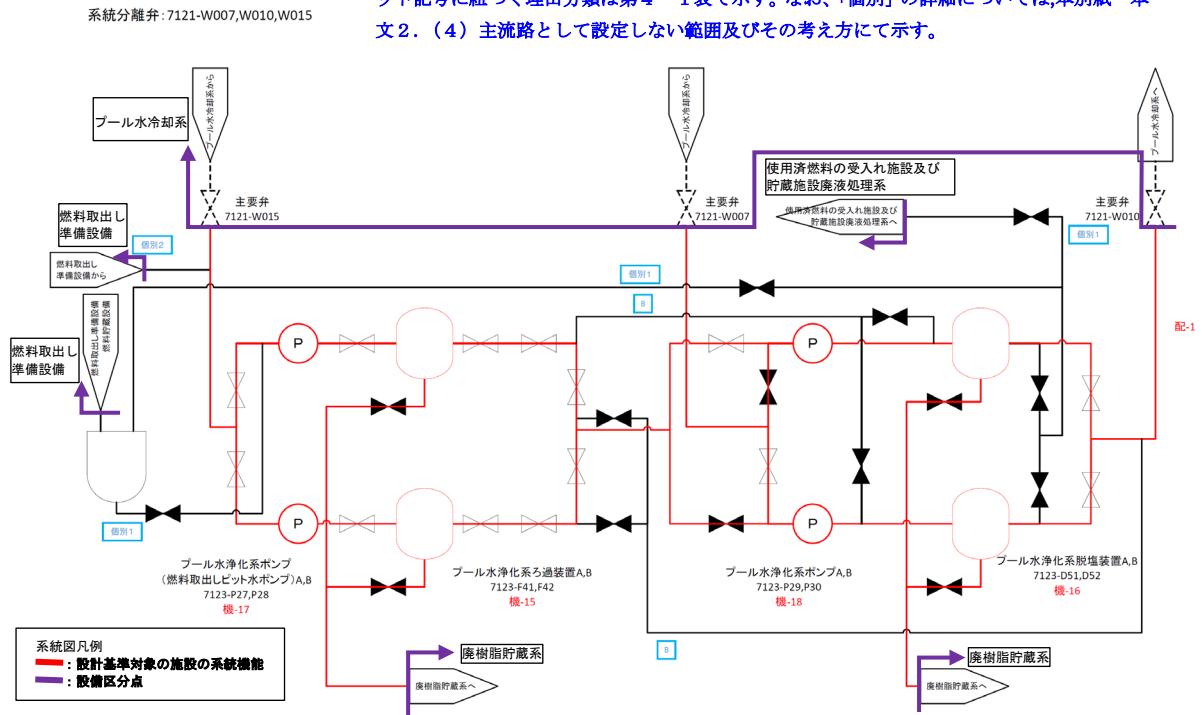
第4-1図 プール水浄化系に係る主流路の範囲及び主流路としていない範囲の概要図
