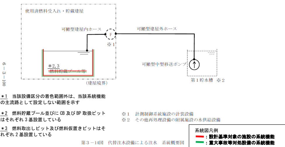
第 2 - 2 図 使用済燃料受入れ設備及び使用済燃料貯蔵設備 系統概要図
