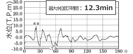
最大下降水位分布 3号取水塔
