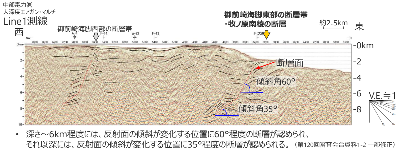
御前崎海脚東部の断層帯・牧ノ原南稜の断層に係る活断層評価結果 (上: Line10測線、下: Line1測線) (第120回審査会合資料)
