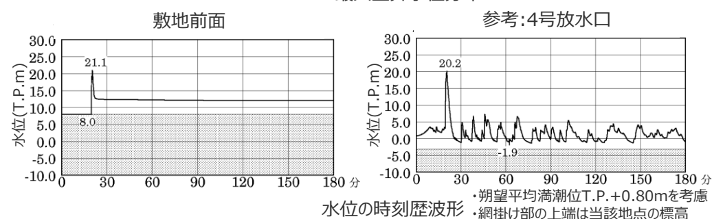
内閣府の最大クラスモデル（ケース①）の敷地への影響
