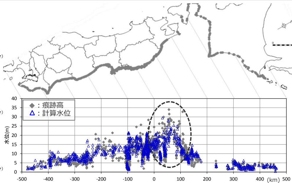
東北沖地震の痕跡高との比較 3)
