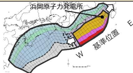
駿河湾内のトラフ軸付近の超大すべり無し (第662回審査会合)
