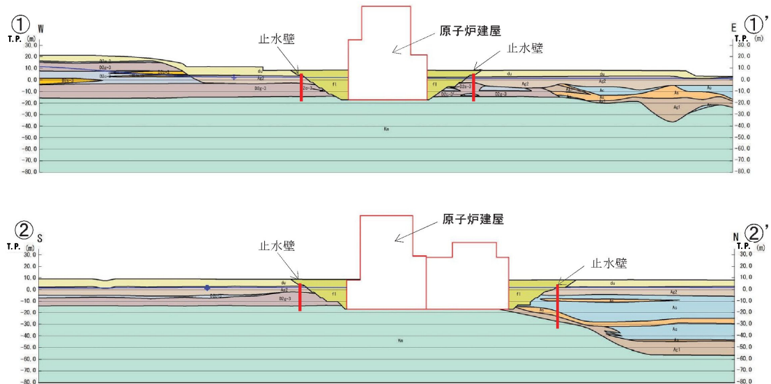
第 2-4 図 原子炉建屋周りの止水壁の設置位置図
