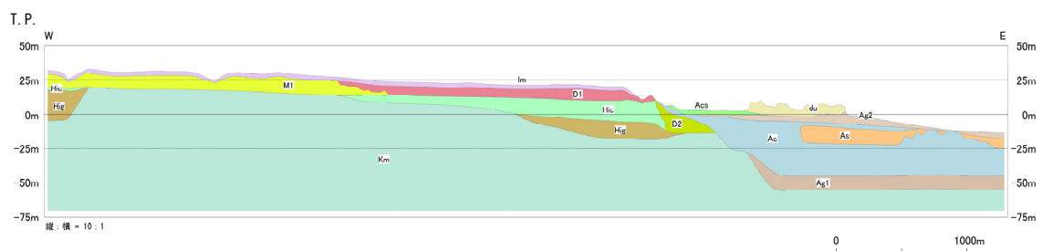
第 1.2-2 図 (3) 敷地及び敷地近傍の地質断面図 (E W 断面)
