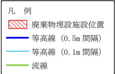
第 1.6.4-6 図 (2) 地下水位等高線図 (D-5-1~D-3-3 ; 動水勾配平均時)
