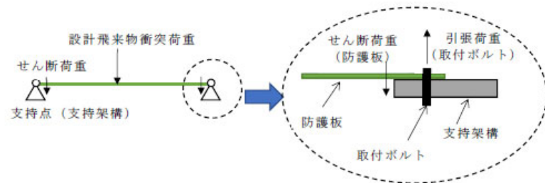
第2-23図 設計飛来物接触直後の荷重
