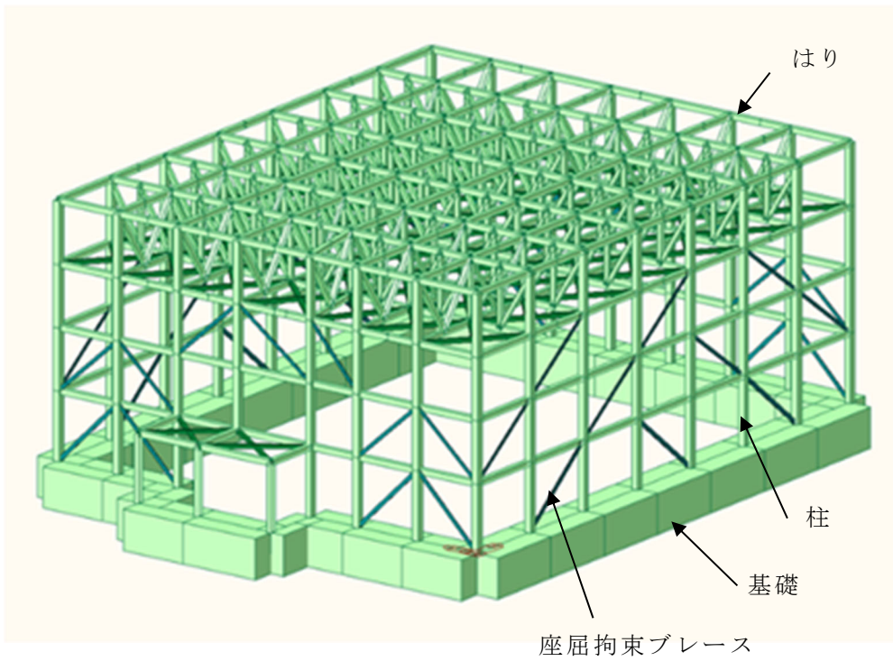
第 2 -32 図 支持架構の構造概要
