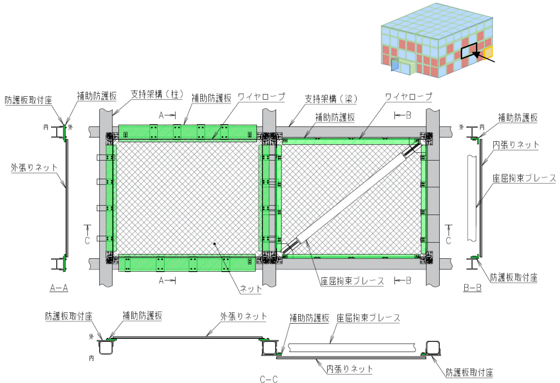
第2-6図 補助防護板と防護ネットの位置関係
