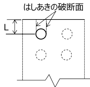
第2-26図 はしあきの破断面
