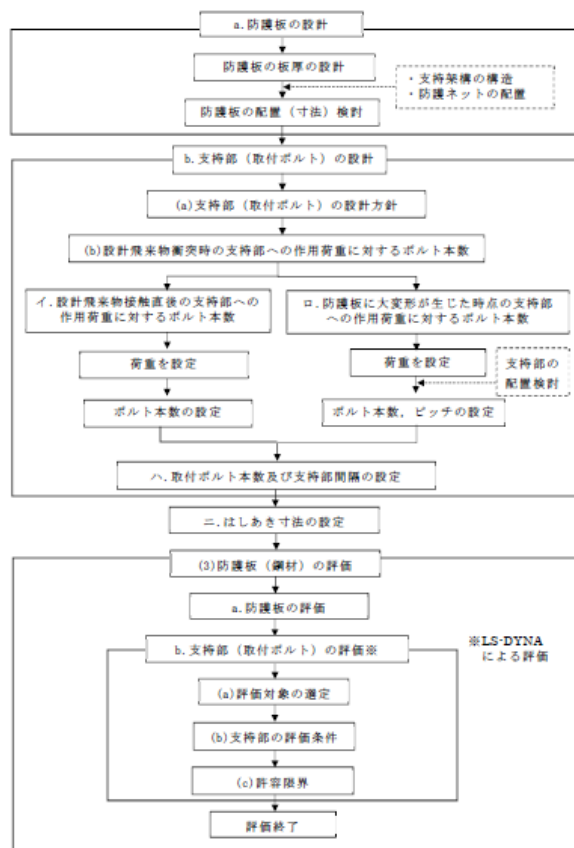
第2-19図 防護板(鋼材)の設計フロー
