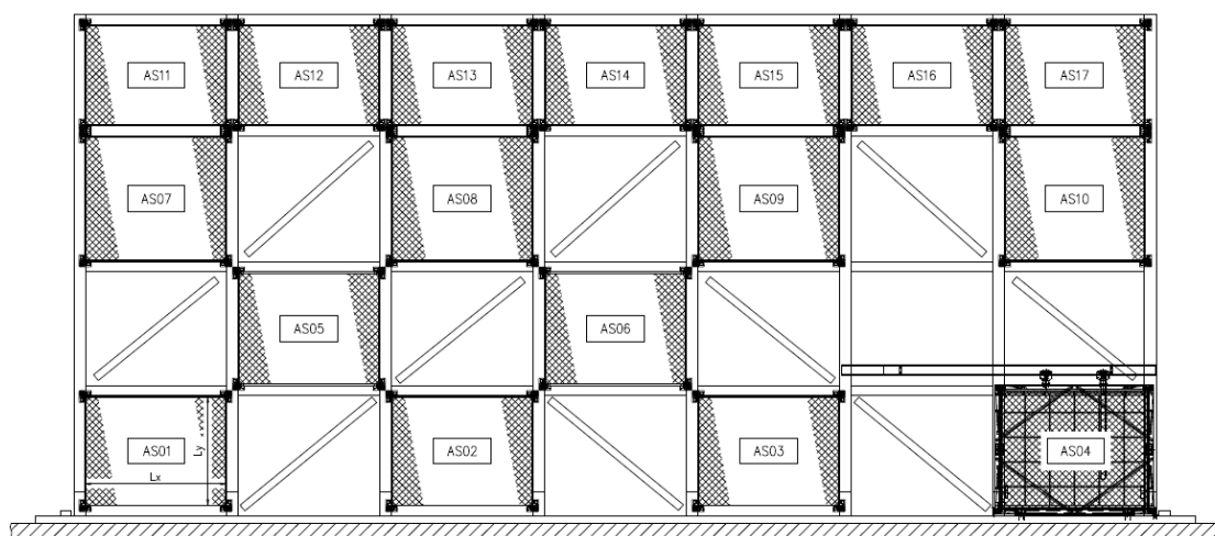
第2.2-1図 ネット割付展開図(南側外面) (2/10)
