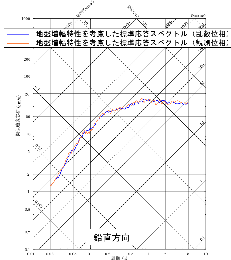
地盤増幅特性を考慮した標準応答スペクトル
