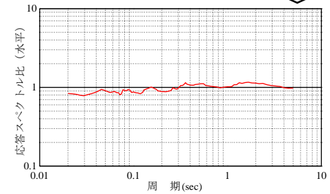
応答スペクトル比 (基準地震動 / 基準地震動の引戻し波)
