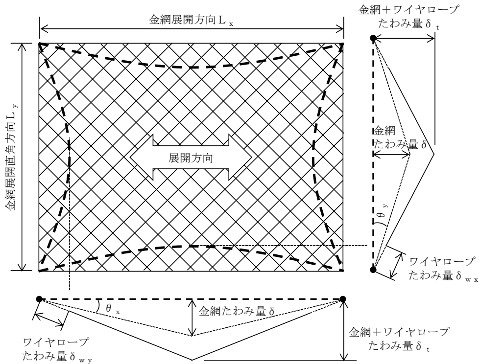
第6.1-10図 ネット及びワイヤロープ変形図
