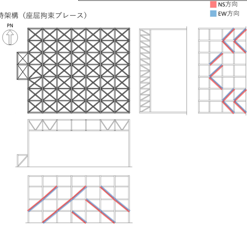
(e) 支持架構(座屈拘束ブレース)
