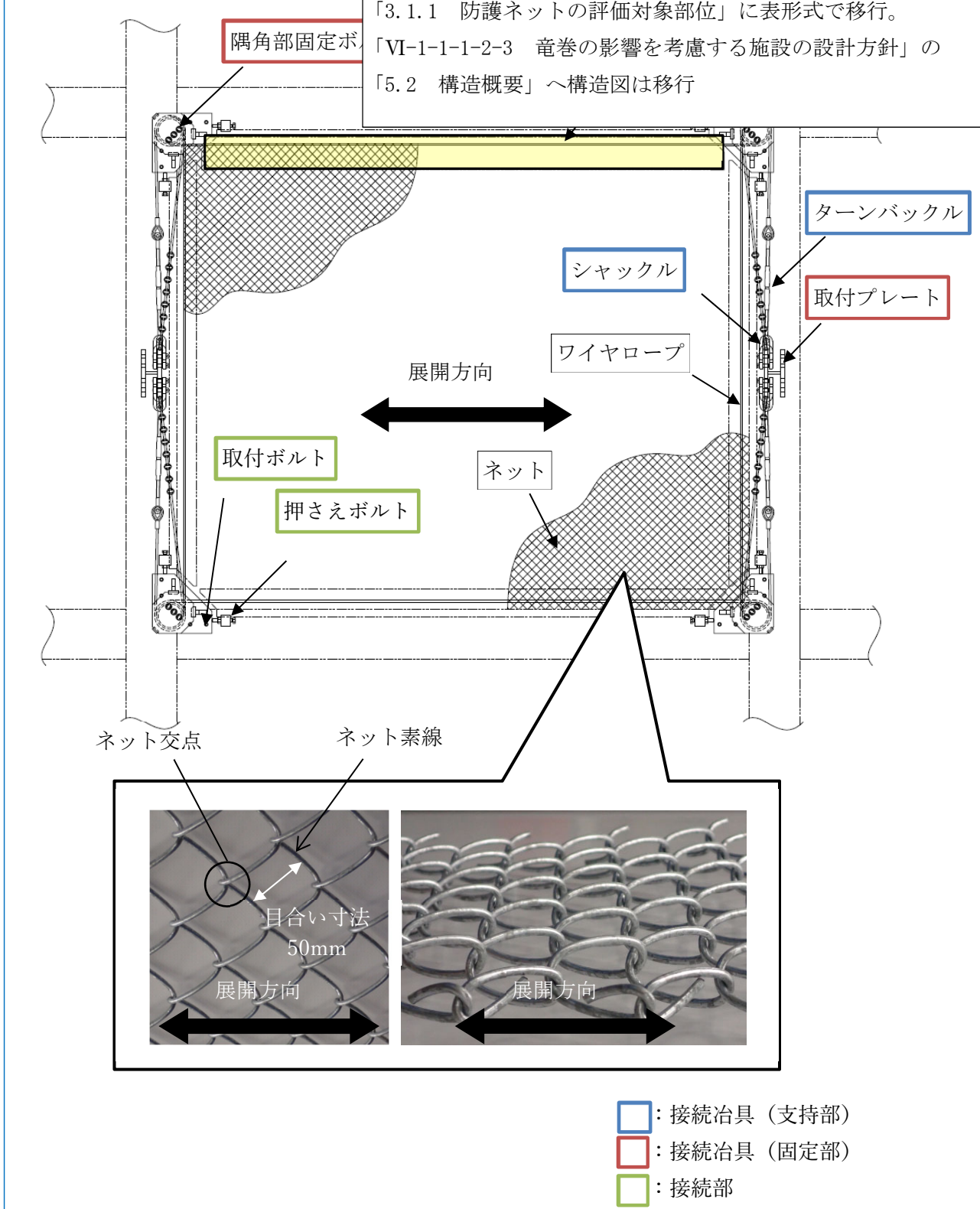
第3.1.1-1図 防護ネット(支持架構に直接設置)の評価対象部位
