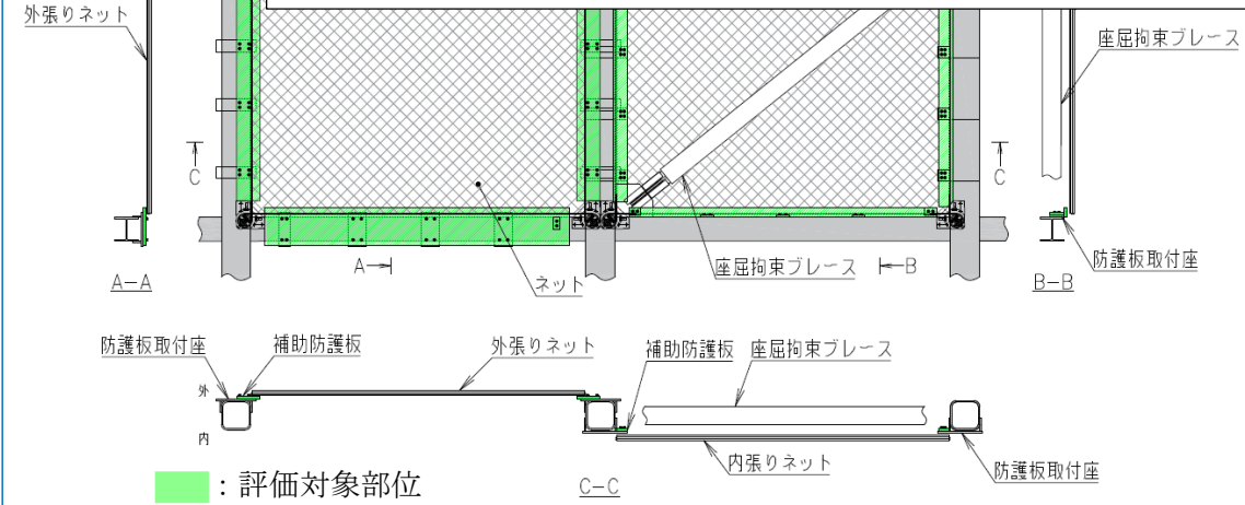
第 3.1.1-6 図 補助防護板の評価対象部位
