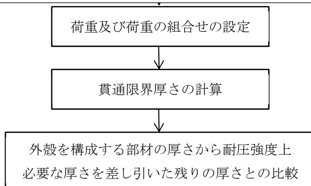
第2.3-1図 配管の衝突評価フロー
