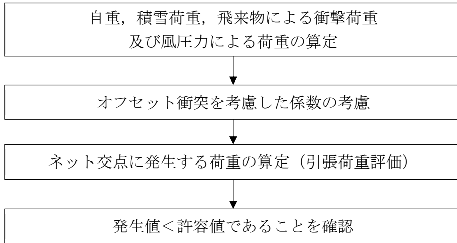
第3.5.1-1図 ネットの破断評価フロー
