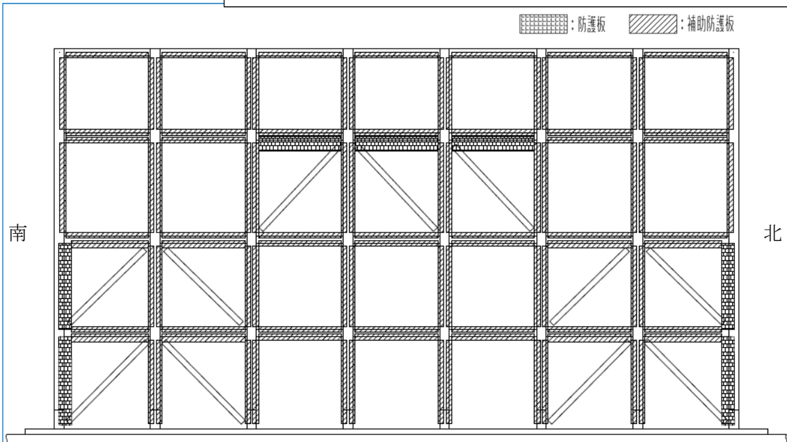
第4.3-1図 防護板及び補助防護板 配置図(東面) (4/6)
