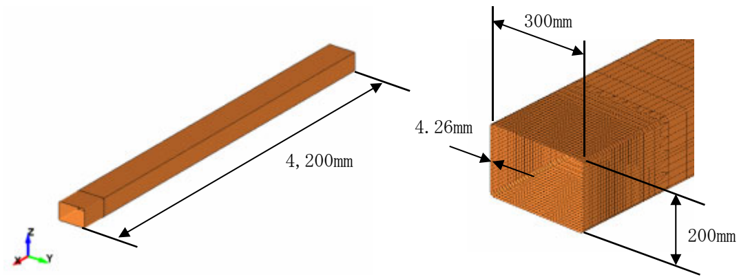
第2.5-2図 飛来物の解析モデル図
