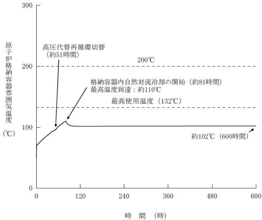
第 7. 1. 2. 26 図 原子炉格納容器雰囲気温度の長期間の推移 (RCP シール LOCA が発生する場合)
