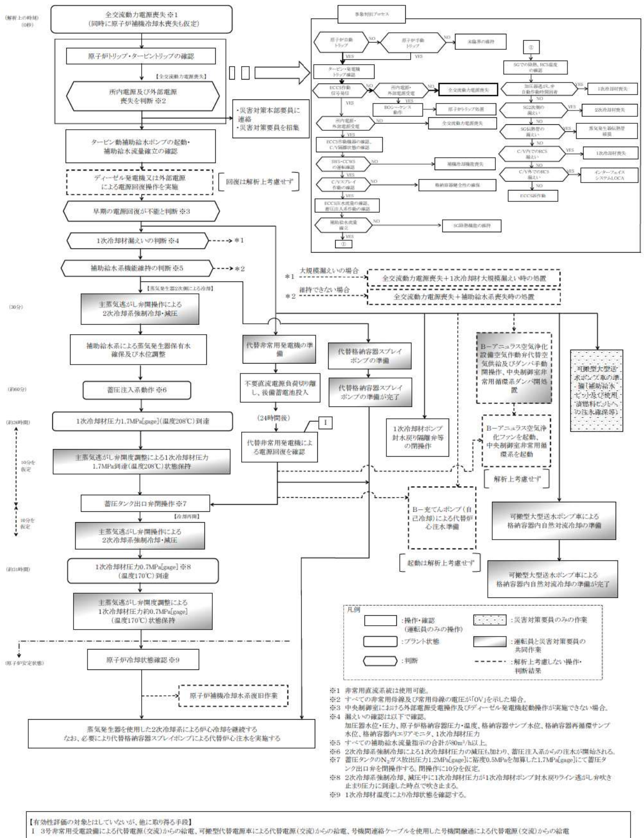
第7.1.2.3 図 「全交流動力電源喪失」の対応手順の概要 (「外部電源喪失時に非常用所内交流電源が喪失し、 原子炉補機冷却機能が喪失する事故」の事象進展)
