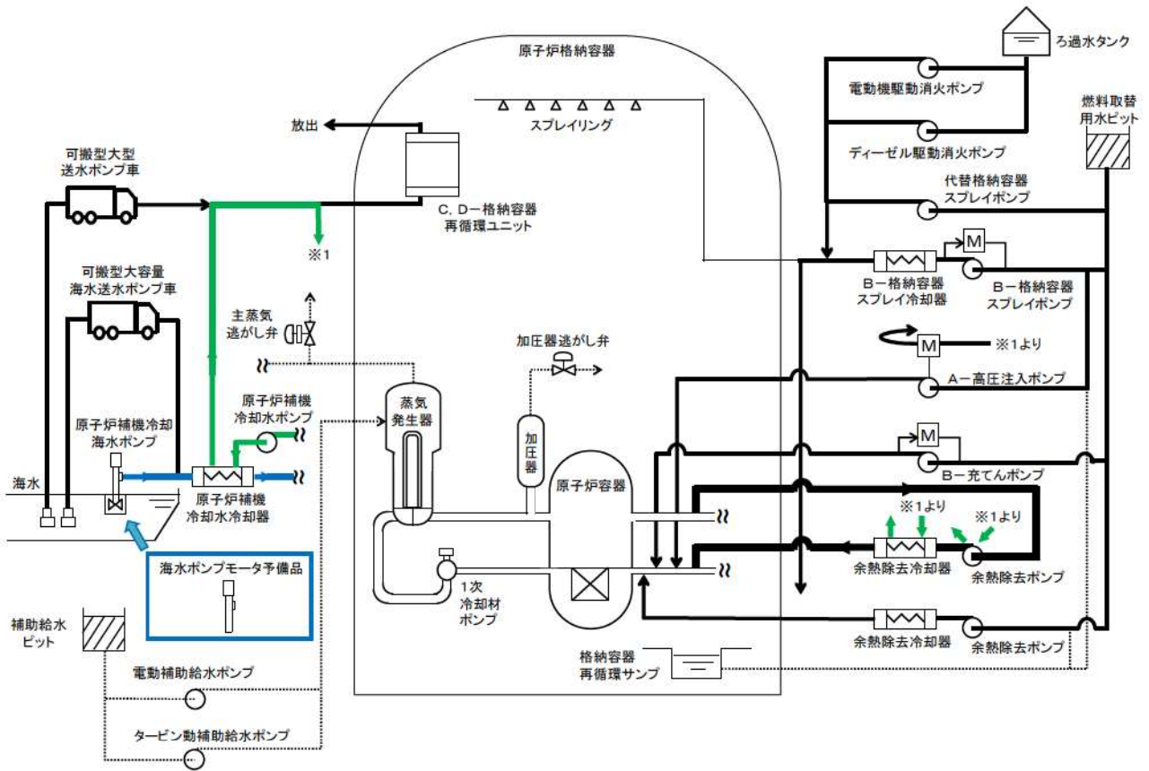
図5 概略系統図
