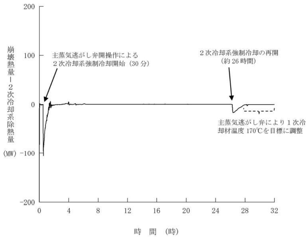
第7.1.2.41図 崩壊熱量と2次冷却系除熱量の推移 (RCP シール LOCA が発生しない場合)
