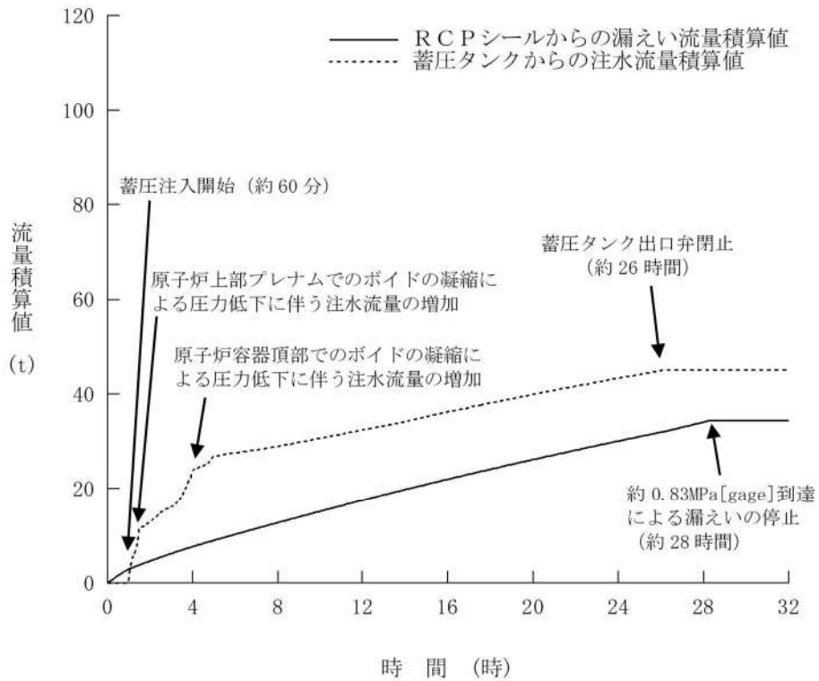
第 7. 1. 2. 30 図 漏えい流量と注水流量の積算値の推移 (RCP シール LOCA が発生しない場合)
