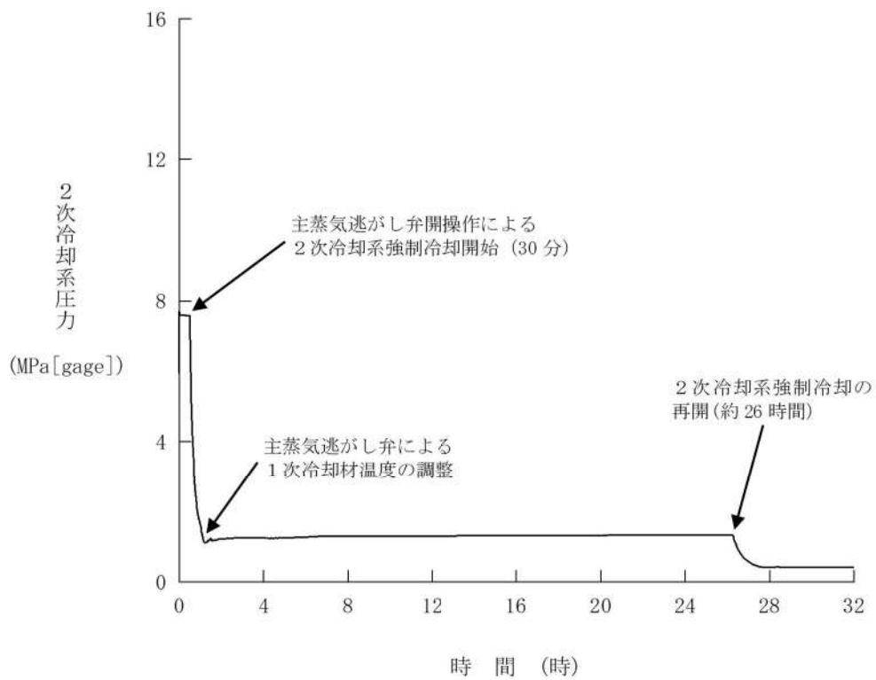
第 7. 1. 2. 36 図 2次冷却系圧力の推移 (RCP シール LOCA が発生しない場合)
