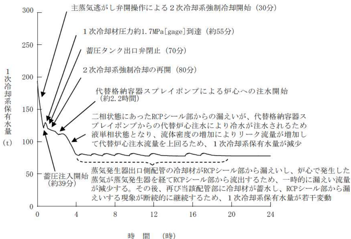
第 7. 1. 2. 8 図 1 次冷却系保有水量の推移 (RCP シール LOCA が発生する場合)
