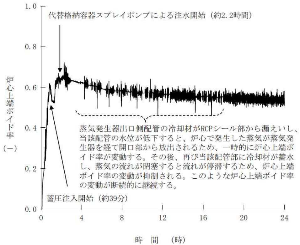
第 7.1.2.14 図 炉心上端ボイド率の推移 (RCP シール LOCA が発生する場合)
