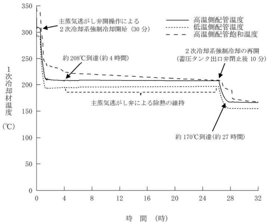
第 7.1.2.28 図 1 次冷却材温度の推移 (RCP シール LOCA が発生しない場合)
