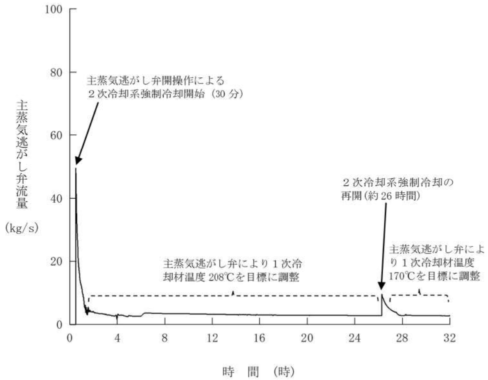
第 7. 1. 2. 37 図 主蒸気逃がし弁流量の推移 (RCP シール LOCA が発生しない場合)
