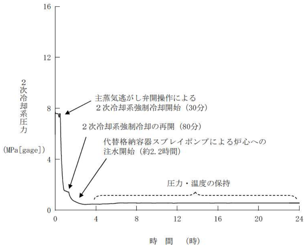
第 7. 1. 2. 17 図 2次冷却系圧力の推移 (RCP シール LOCA が発生する場合)
