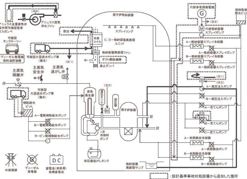
図 2 「外部電源喪失時に非常用所内交流電源が喪失し、原子炉補機冷却機能の喪失及びRCPシールLOCAが発生する事故」の重大事故等対策の概略系統図 (格納容器内自然対流冷却及び高压代替再循環)
