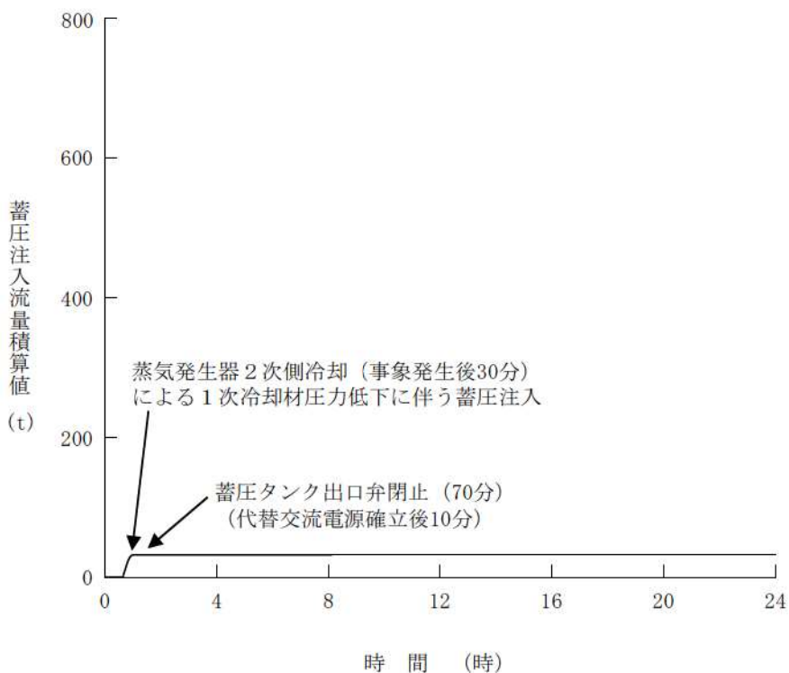
第 7. 1. 2. 9 図 蓄圧注入流量積算値の推移 (RCP シール LOCA が発生する場合)
