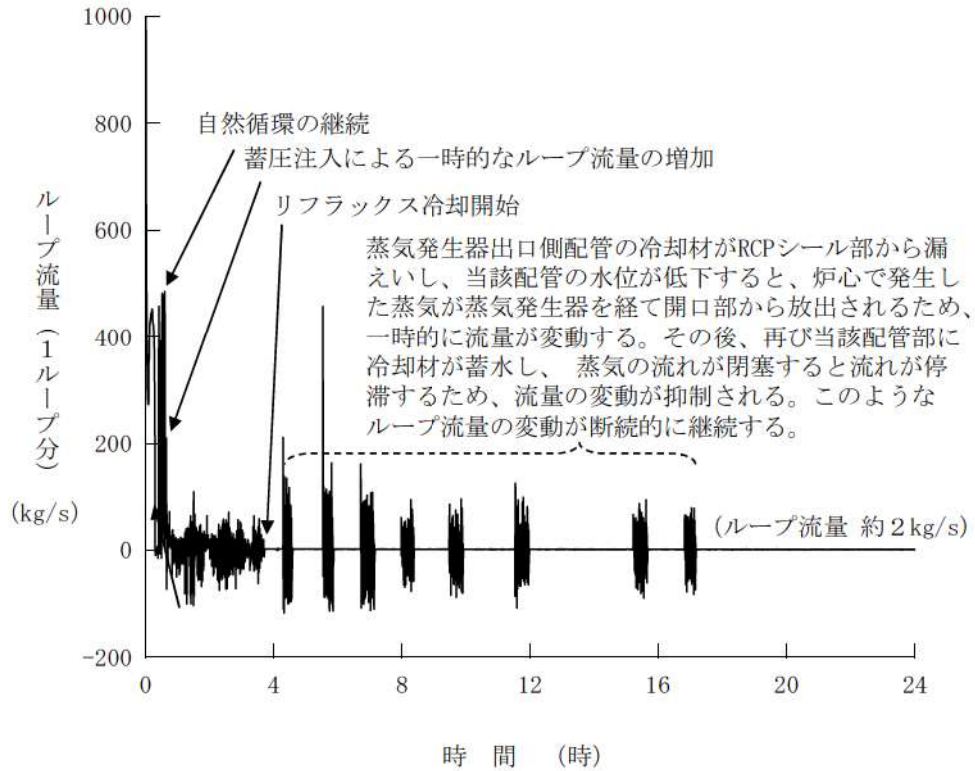
第 7. 1. 2. 12 図 1 次冷却材流量の推移 (RCP シール LOCA が発生する場合)
