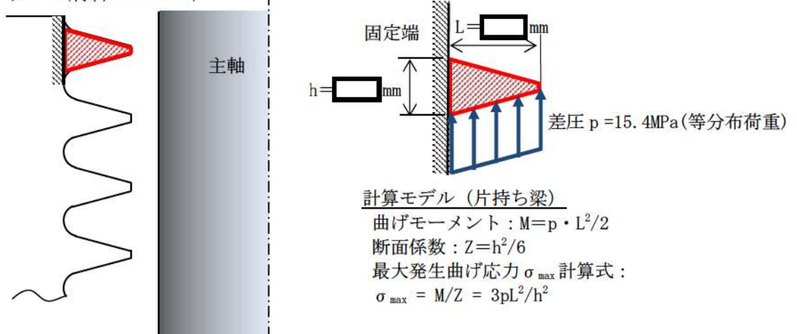
ラビリンス (材料: SUSF304)
