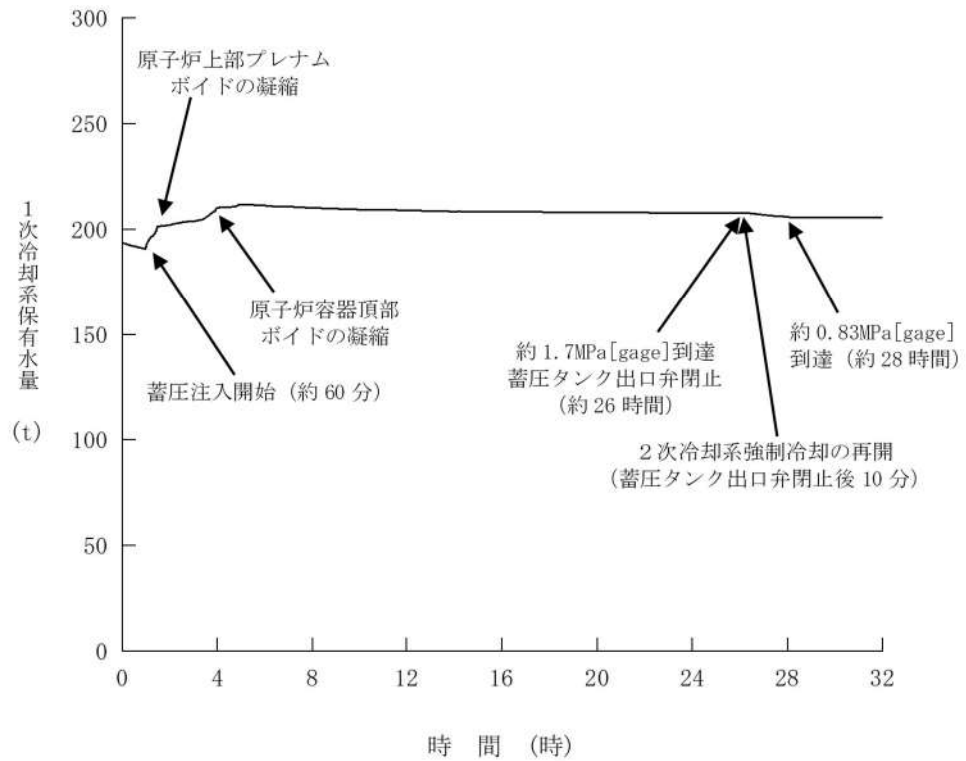
第 7. 1. 2. 29 図 1 次冷却系保有水量の推移 (RCP シール LOCA が発生しない場合)
