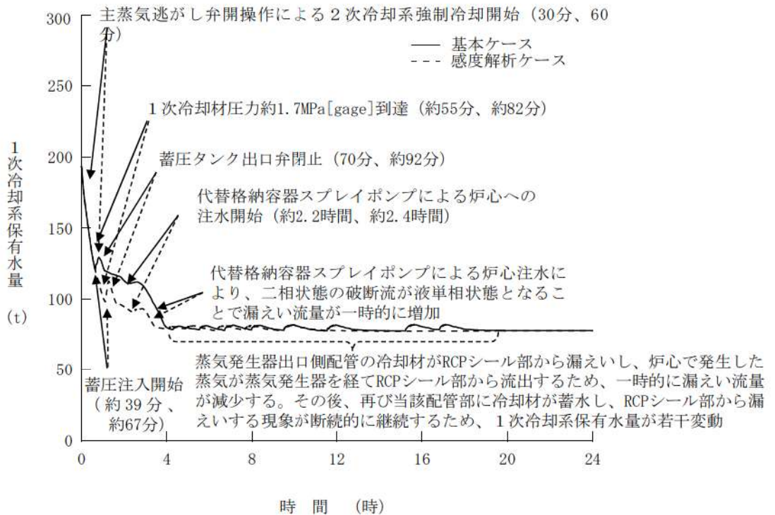
第 7.1.2.45 図 1次冷却系保有水量の推移 (RCP シール LOCA が発生する場合) (主蒸気逃がし弁操作時間余裕確認)
