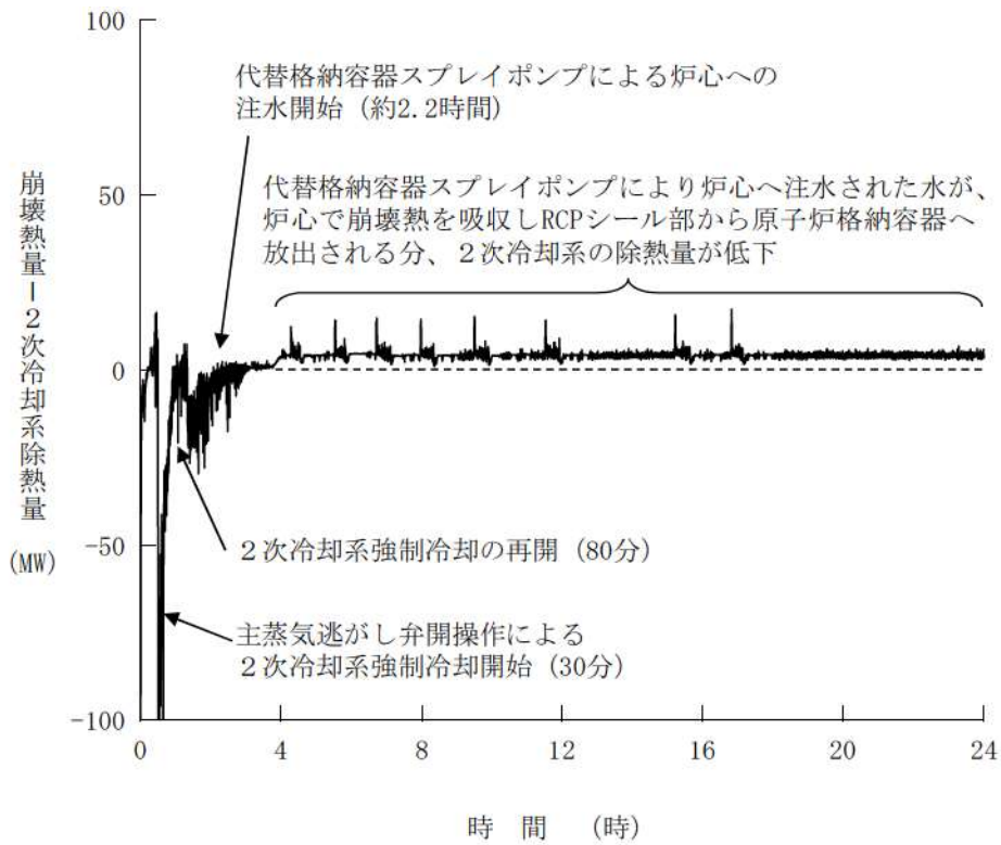
第 7. 1. 2. 22 図 崩壊熱量と 2 次冷却系除熱量の推移 (RCP シール LOCA が発生する場合)
