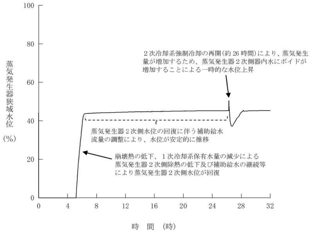
第 7.1.2.39 図 蒸気発生器狭域水位の推移 (RCP シール LOCA が発生しない場合)
