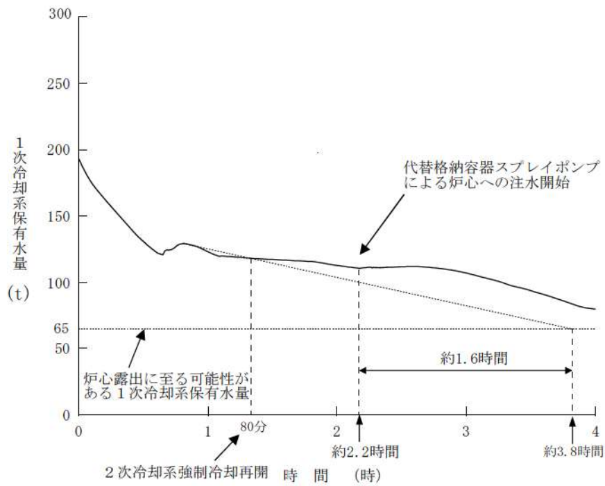
第 7.1.2.47 図 1次冷却系保有水量の推移 (RCP シール LOCA が発生する場合) (代替炉心注水操作時間余裕確認)
