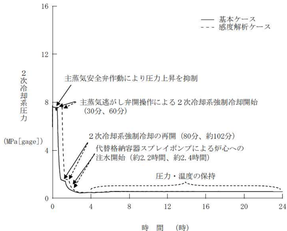
第 7.1.2.43 図 2 次冷却系圧力の推移 (RCP シール LOCA が発生する場合) (主蒸気逃がし弁操作時間余裕確認)
