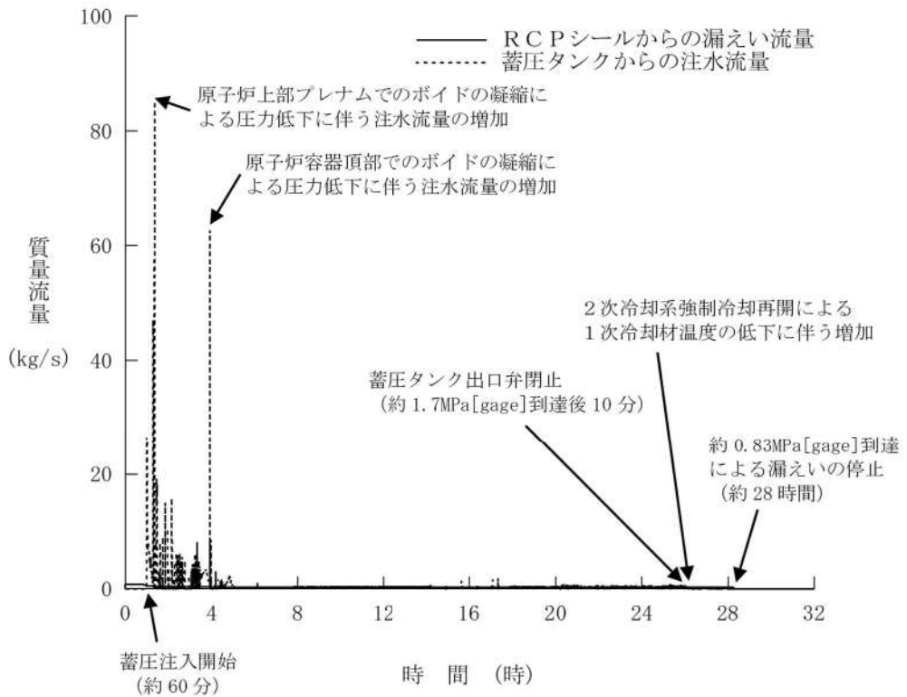
第 7.1.2.31 図 漏えい流量と注水流量の推移 (RCP シール LOCA が発生しない場合)
