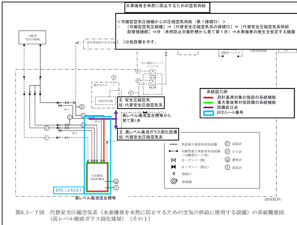
第3-13図 代替安全圧縮空気系 （水素爆発を未然に防止するための空気の供給に使用する設備）の系統概要図 （第1接続口） （事業変更許可申請書 添付書類六 第9.3-7図抜粋）
