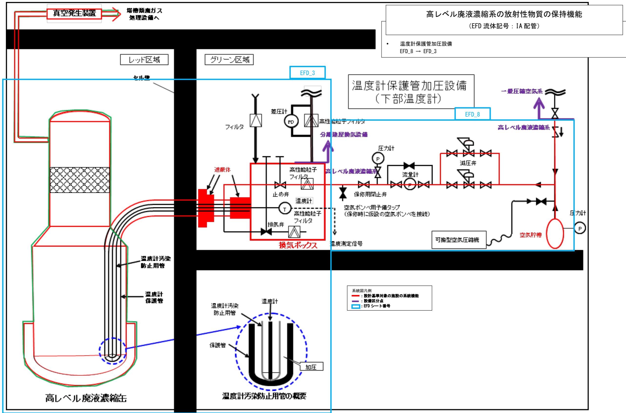
第3-1図(3) 高レベル廃液濃縮缶 温度計保護管加圧設備 (下部温度計) 系統概要図 (放射性物質の保持機能)
