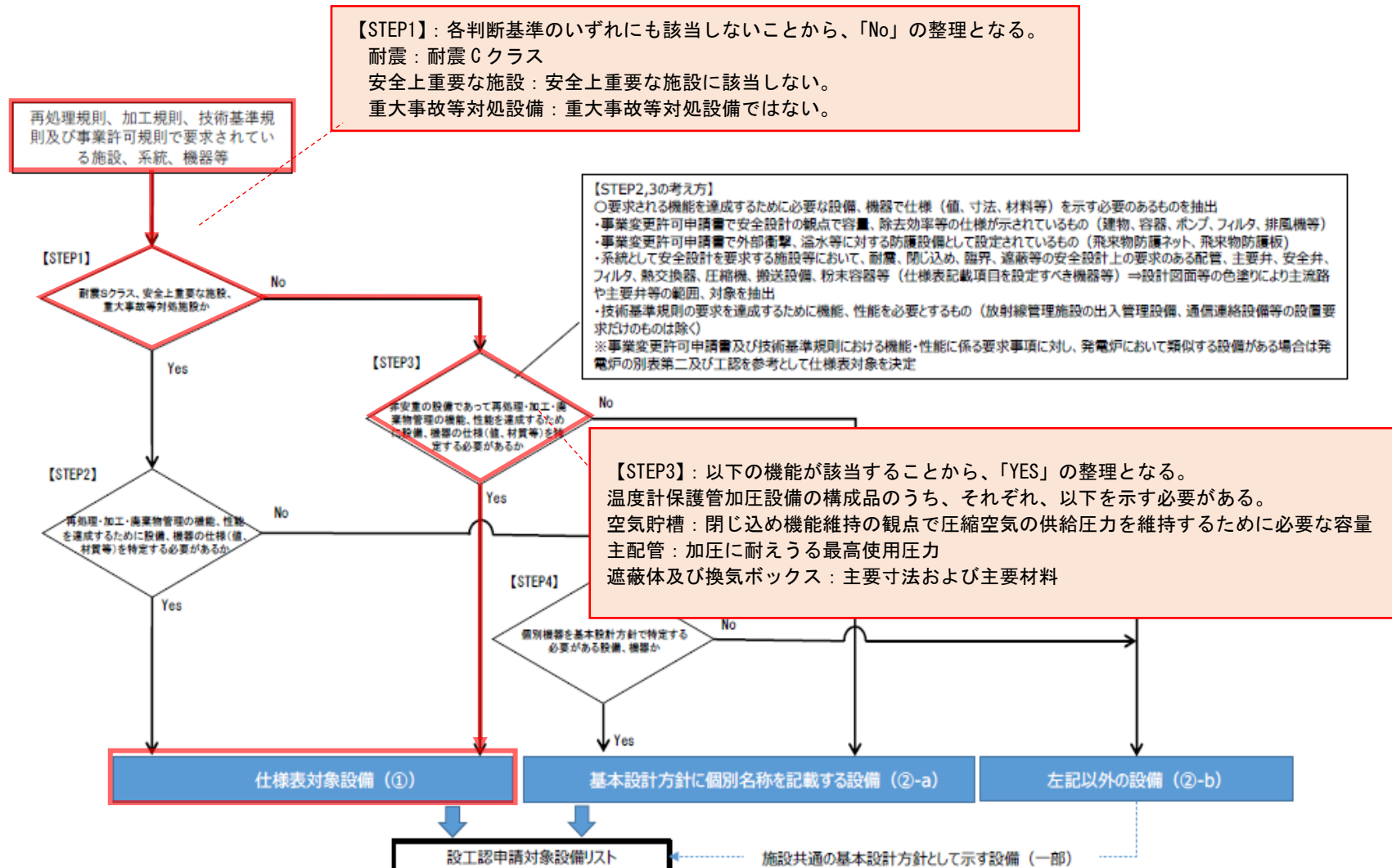
第2-2図(3) 高レベル廃液濃縮缶 温度計保護管加圧設備に対する設備選定フローでの整理
