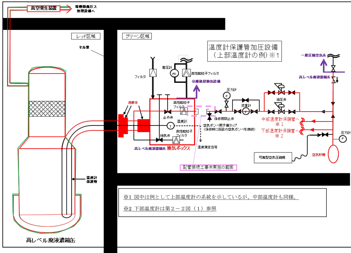
第2-2図(2) 高レベル廃液濃縮缶 温度計保護管加圧設備 (上部温度計・中部温度計) 系統概要図
