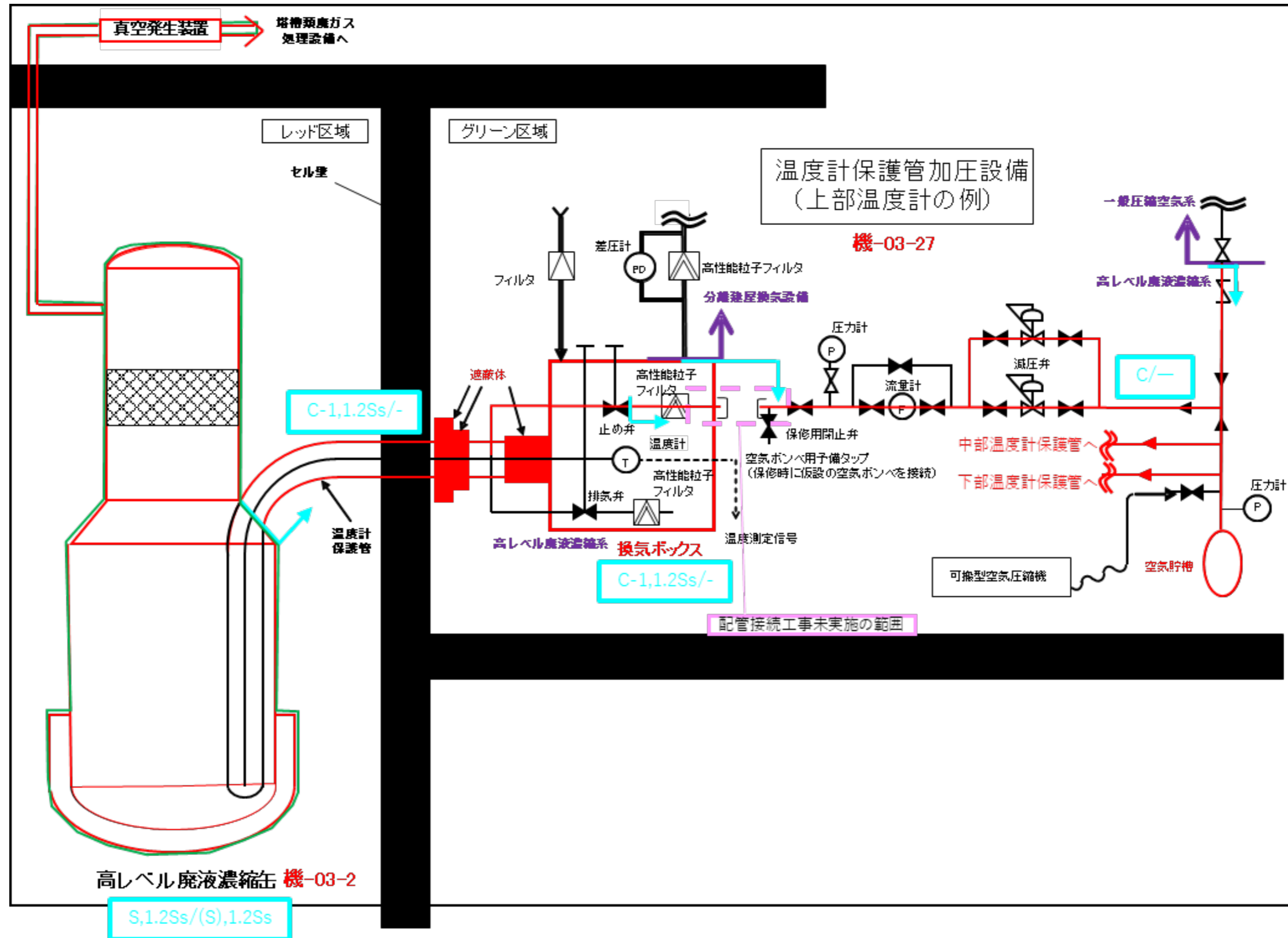
第5-1図(4) 温度計保護管加圧設備(上部温度計・中部温度計)の耐震クラス範囲の概要図
