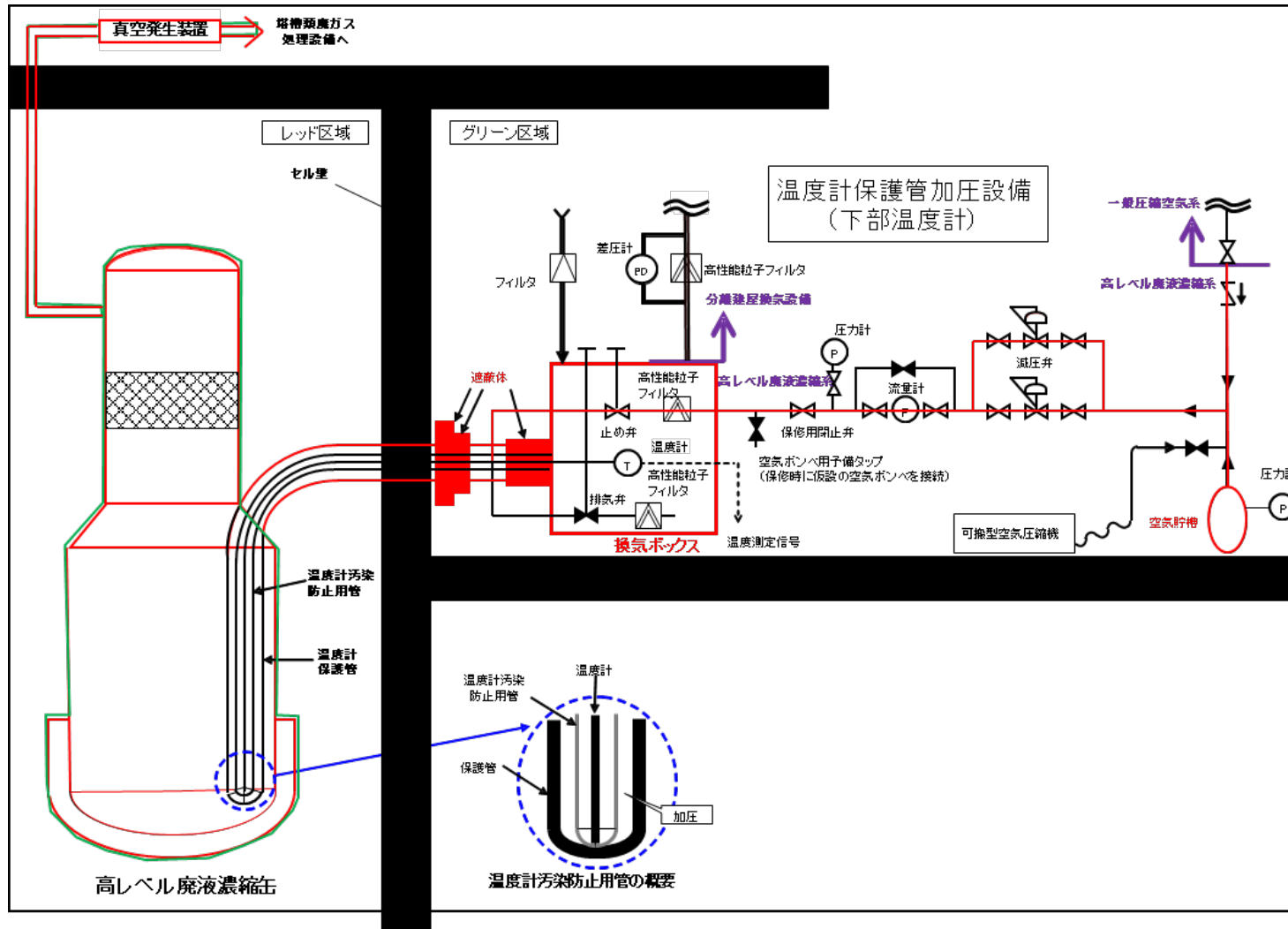
第2-2図(1) 高レベル廃液濃縮缶 温度計保護管加圧設備(下部温度計) 系統概要図
