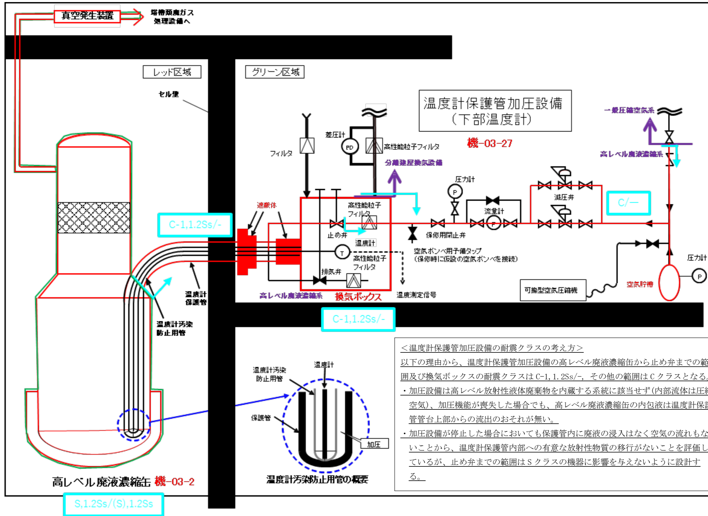
第5-1図(3) 温度計保護管加圧設備(下部温度計)の耐震クラス範囲の概要図
