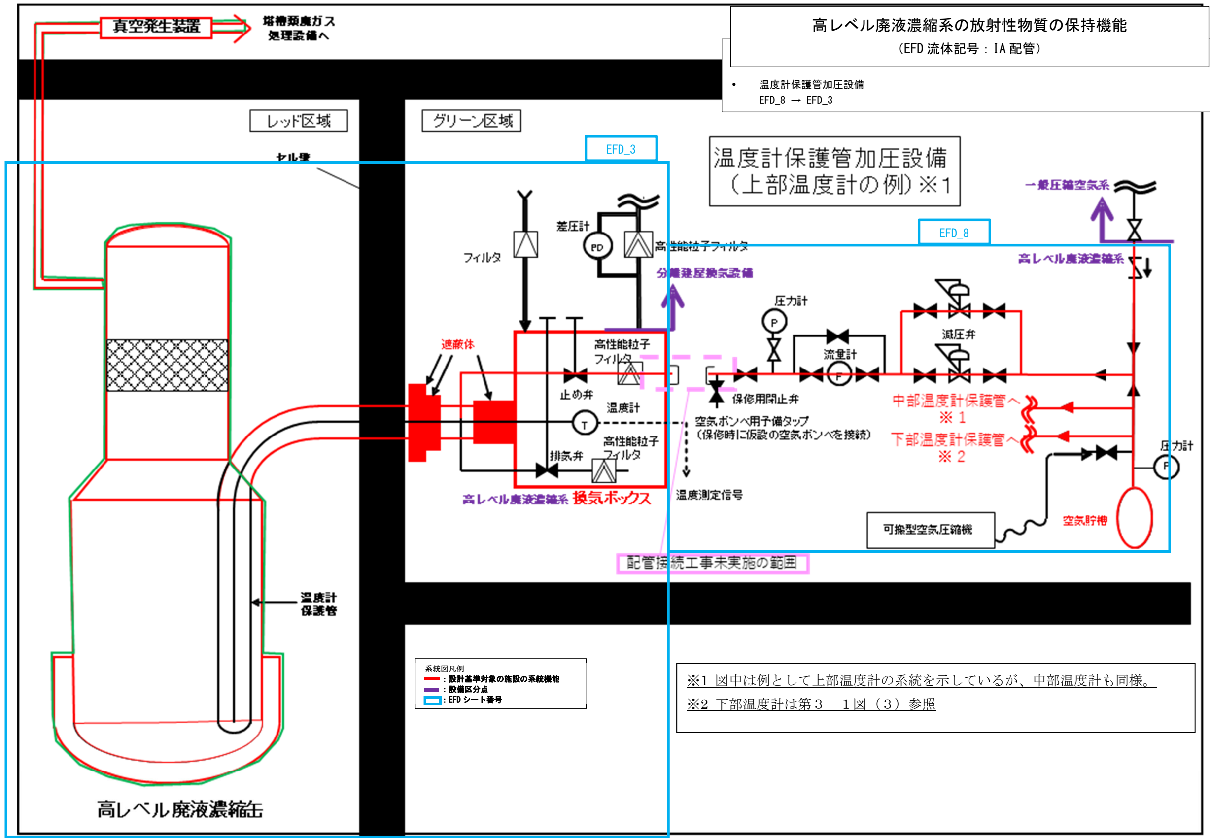
第3-1図(4) 高レベル廃液濃縮缶 温度計保護管加圧設備 (上部・中部温度計) 系統概要図 (放射性物質の保持機能)
