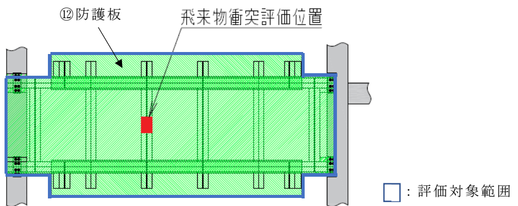
第 2 -29 図 相対する 2 辺以上で支持する防護板 設計飛来物衝突評価(鉛直)位置
