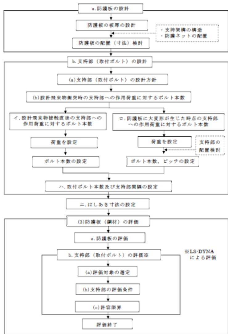
第2-19図 防護板(鋼材)の設計フロー
