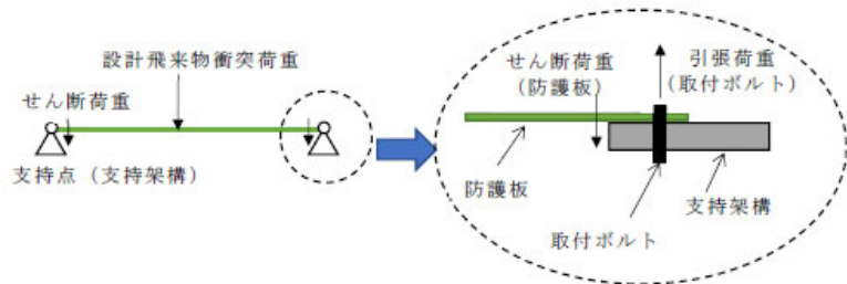
第 2-24 図 設計飛来物接触直後の荷重
