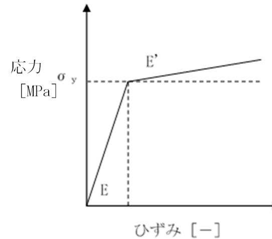
第 6.2.2-1 図 バイリニア型応力-ひずみ関係の概念図
