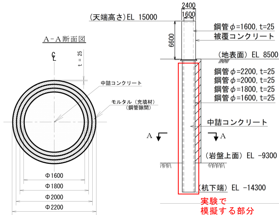
図 2-1 水平載荷実験で使用する実験体で模擬する範囲
