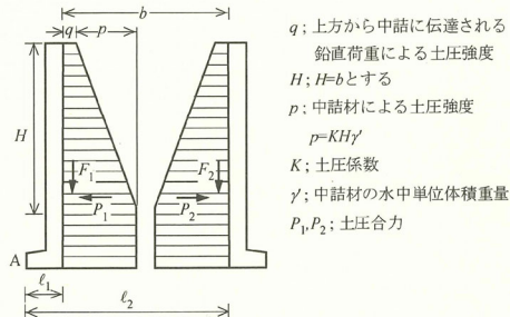
図-2.2.14 壁面摩擦抵抗の求め方
