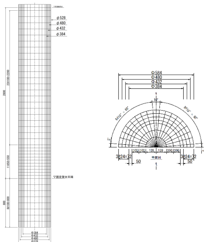
正面図（断面）
