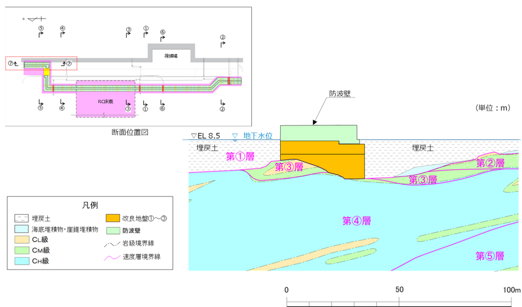
図 3.5.1-8 地質断面図（⑦-⑦断面）
