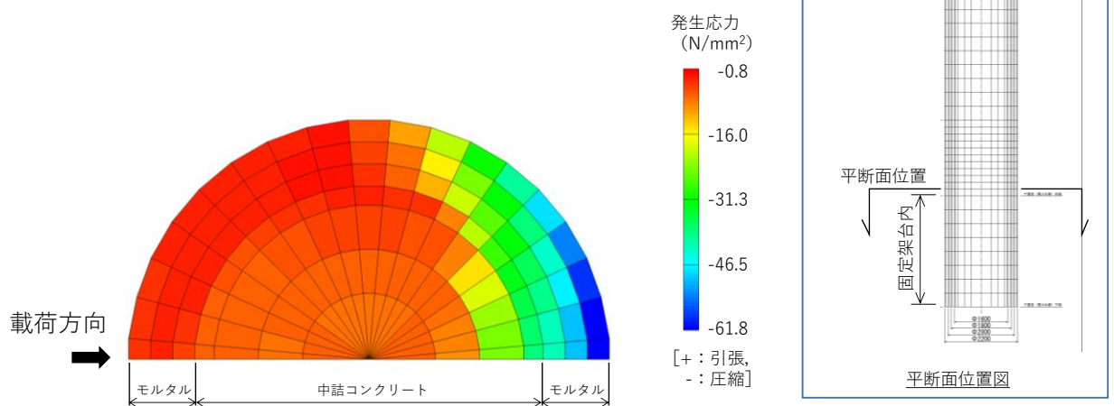
図 4-6(2) 中詰コンクリート及びモルタル（充填材）の応力図（平断面図） （実構造物スケール解析，降伏モーメント超過時，最小主応力）
