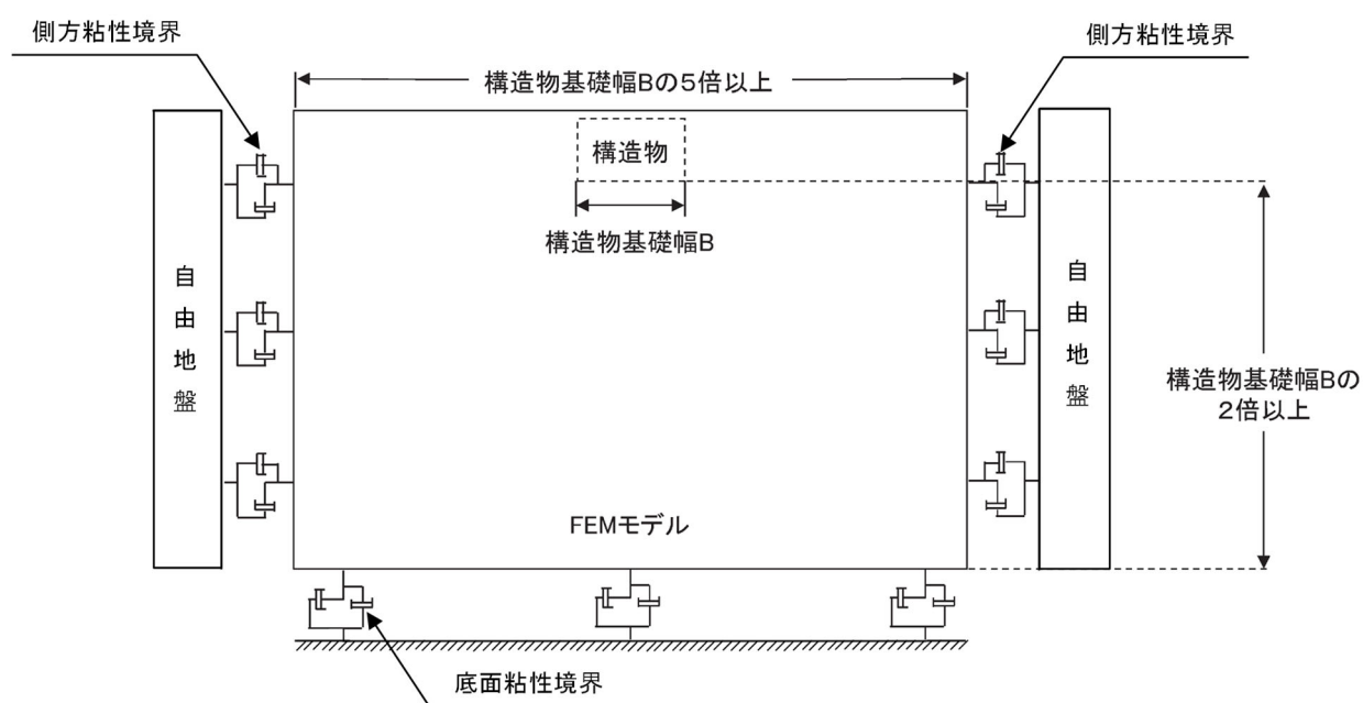
図 3.5.1-12 地震応答解析における境界条件の概念図
