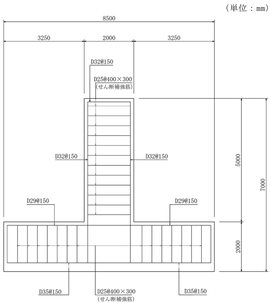
図 2.2-6 防波壁（逆 T 擁壁）の概略配筋図
