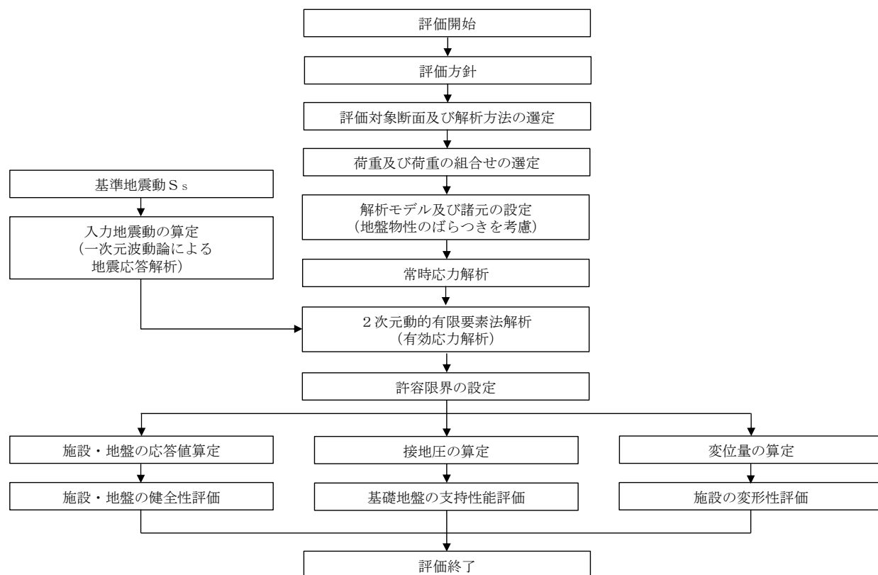
図 2.3-1 防波壁(逆 T 擁壁)の耐震評価フロー
