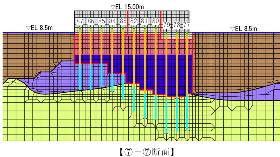
図 3.5.2-3(2) 各解析モデルにおけるグラウンドアンカ位置
