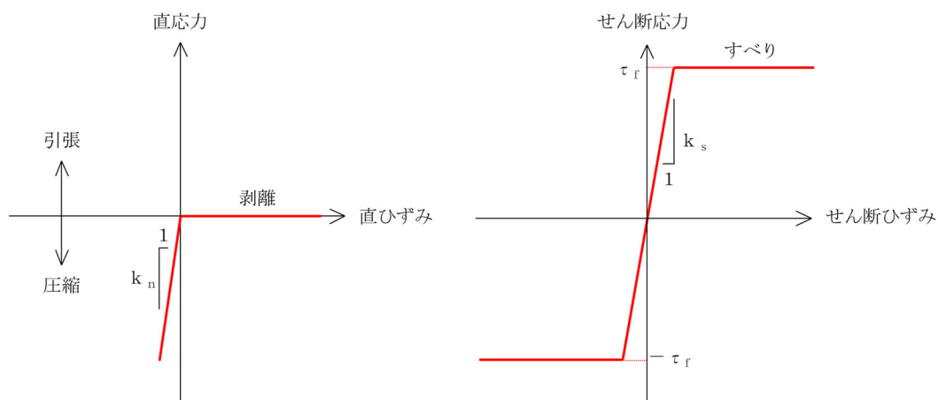
図 3.5.1-26 ジョイント要素の力学特性
