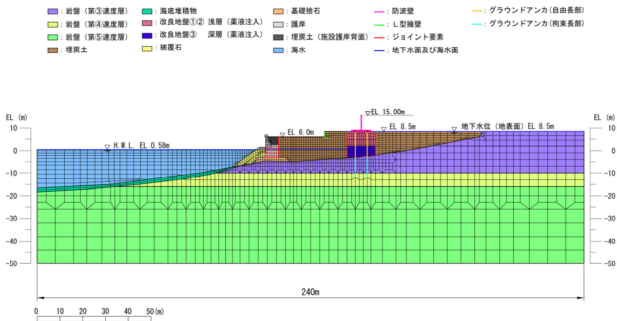
図 3.5.1-1 地震応答解析モデル（①－①断面）
