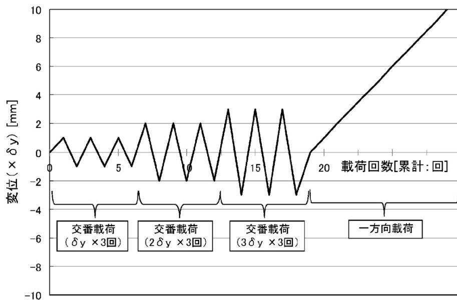
図 2-7 正負交番載荷の方法
