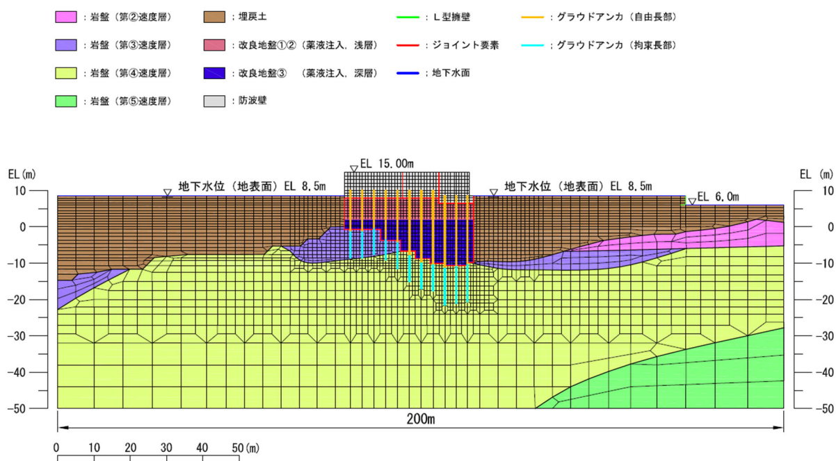
図 3.5.1-7 地震応答解析モデル（⑦-⑦断面）
