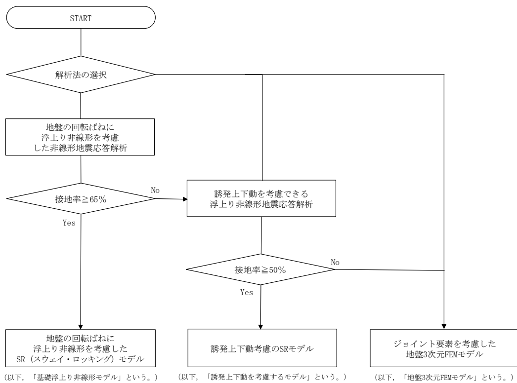
第 5. -1 図 解析モデル選定フロー
