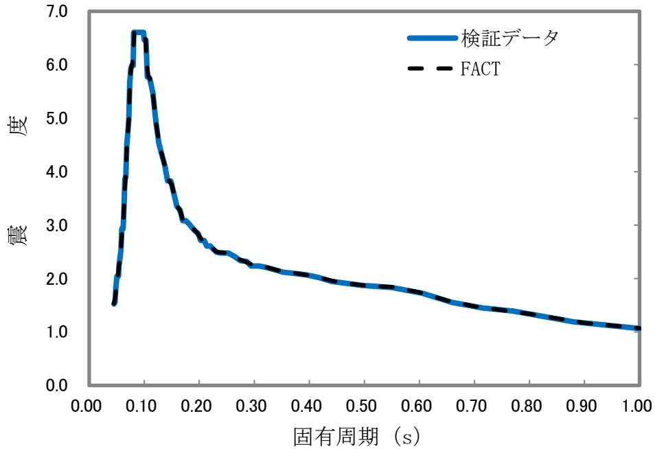
第3-3図 検証用データと本解析コードの比較結果 (EW方向床レベル55.30m 減衰1.0%)
