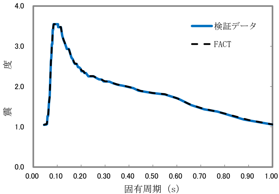
第3-4図 検証用データと本解析コードの比較結果 (NS方向床レベル47.70m 減衰1.0%)
