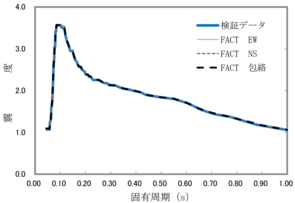
第3-6 図 検証用データと本解析コードの比較結果 (水平方向包絡 床レベル 47.70m 減衰 1.0%)
