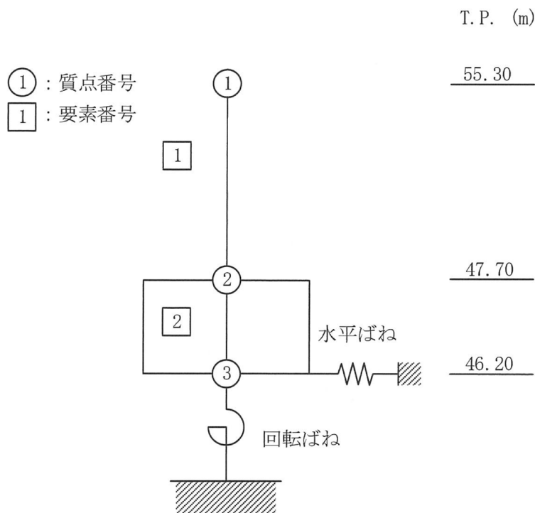
第3-2図 第1非常用ディーゼル発電設備用重油タンク室地震応答解析モデル (水平方向)
