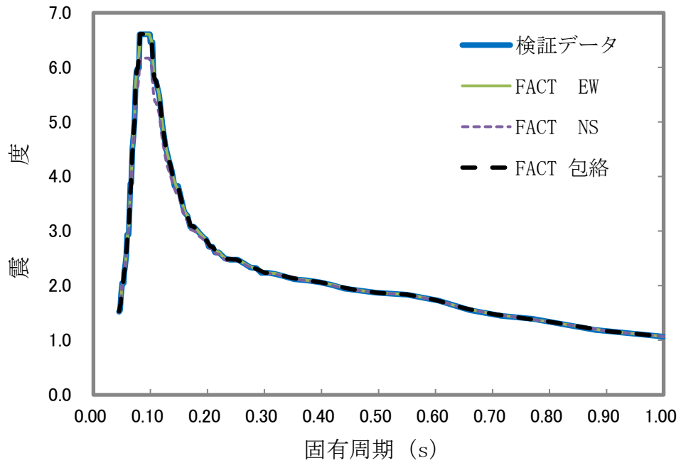
第3-5 図 検証用データと本解析コードの比較結果 (水平方向包絡 床レベル 55.30m 減衰 1.0%)
