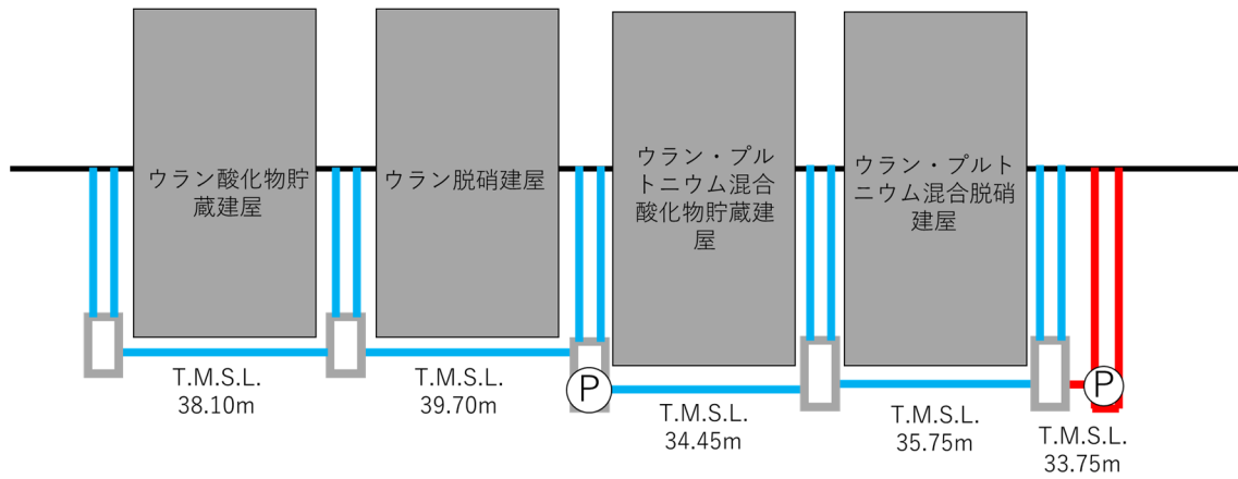
第 3.-2 図 集水エリア 4（ウラン・プルトニウム混合脱硝建屋，ウラン・プルトニウム混合酸化物貯蔵建屋，ウラン脱硝建屋，ウラン酸化物貯蔵建屋）の各建物・構築物の集水管レベル
