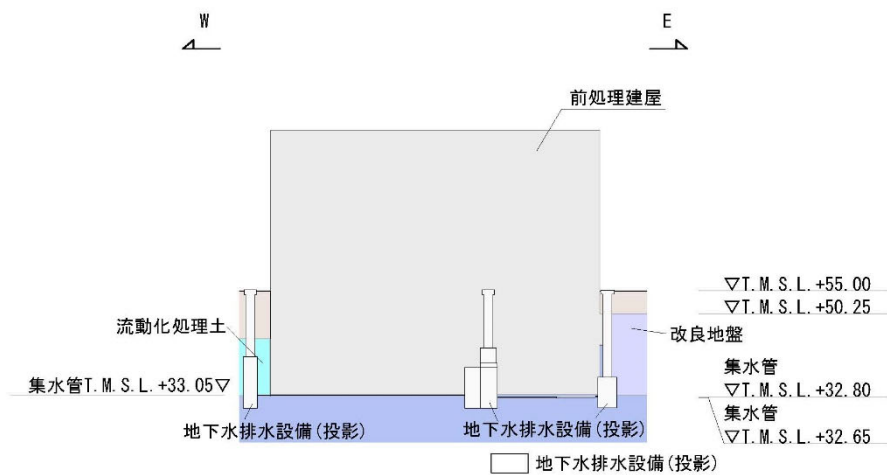
B - B 立面図
