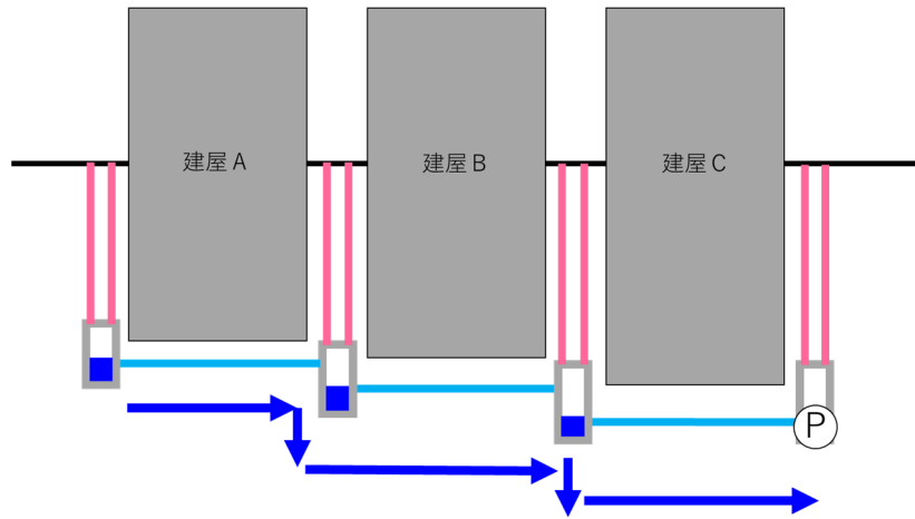
第 4.1-4 図 各集水管から耐震ポンプを設置するピットへの地下水の流れ
