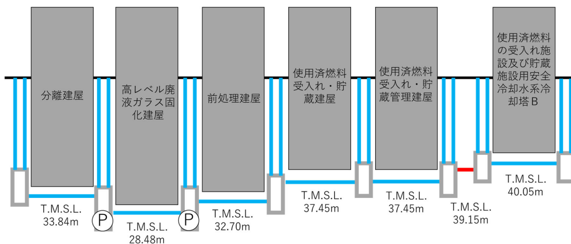
第 1.-2 図 集水エリア 1 (前処理建屋, 分離建屋, 使用済燃料受入れ・貯蔵建屋, 高レベル廃液ガラス固化建屋, 使用済燃料受入れ・貯蔵管理建屋, 使用済燃料の受入れ施設及び貯蔵施設用安全冷却水系冷却塔 B) の各建物・構築物の集水管レベル
