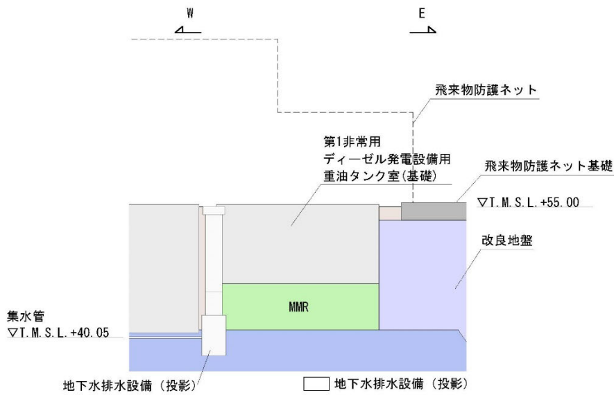
B - B 立面図
