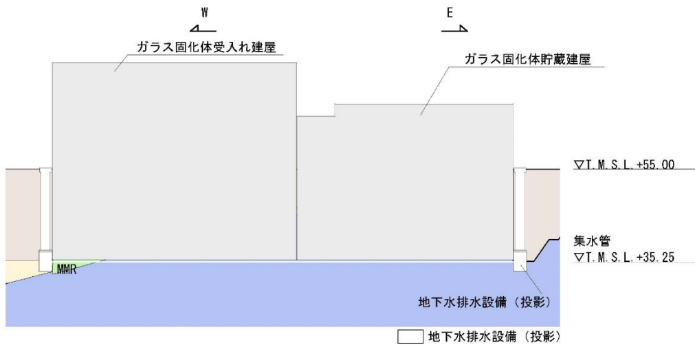
B - B 立面図
