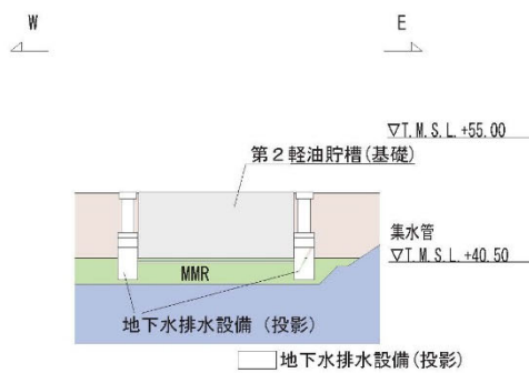
B - B 立面図
