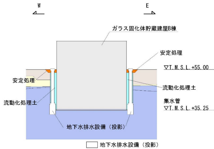
B - B 立面図
