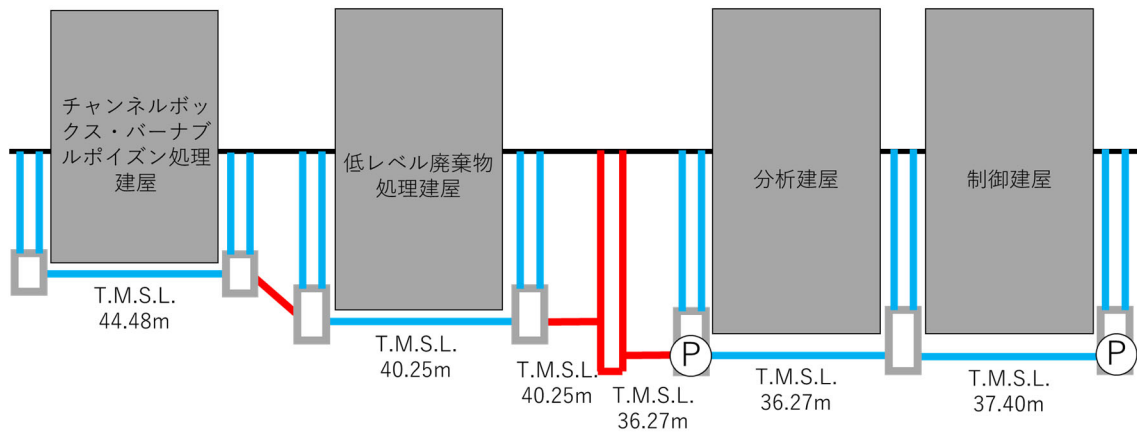
第 2.-2 図 集水エリア 3（制御建屋，チャンネルボックス・バーナブルポイズン処理建屋，分析建屋，低レベル廃棄物処理建屋）の各建物・構築物の集水管レベル
