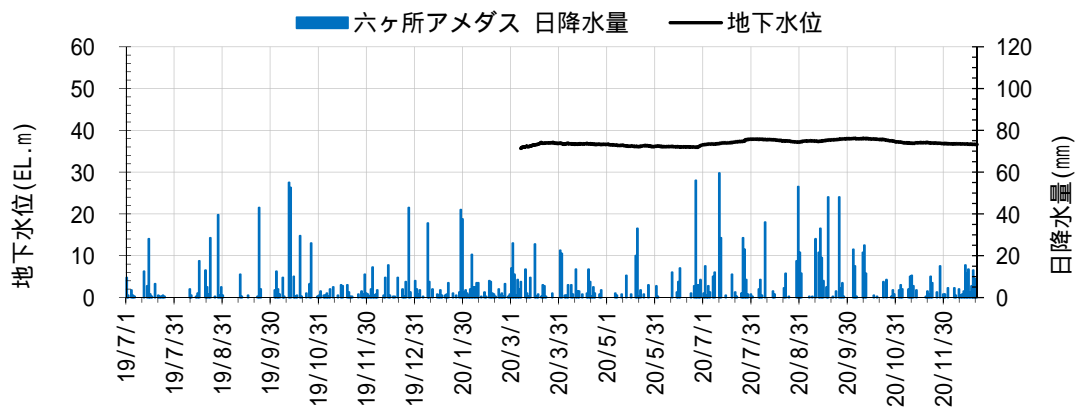
第 1.-1 図(12) EGW-1 孔における地下水水位観測記録と降水量データ
