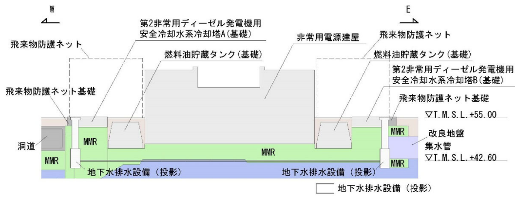
C - C 立面図
