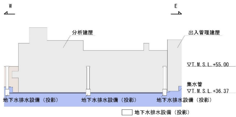
B - B 立面図
