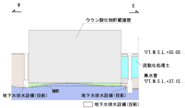
B - B 立面図
