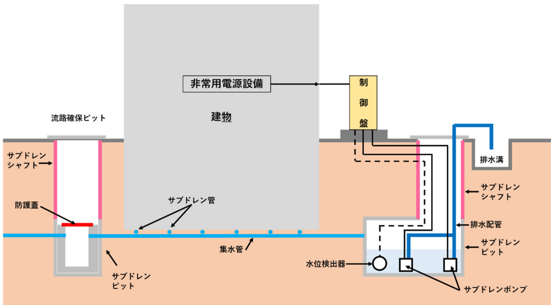
第 4.1-3 図 地下水排水設備の設備概要 (エリア 3)
