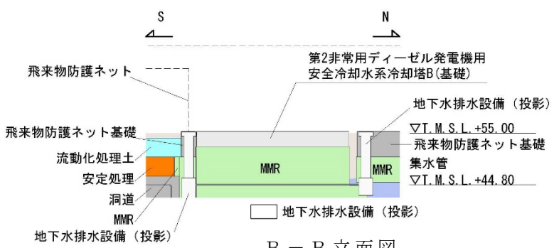
B - B 立面図
