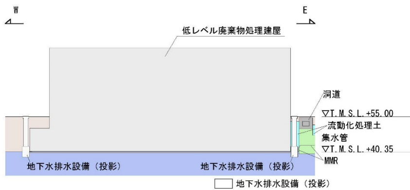
B - B 立面図
