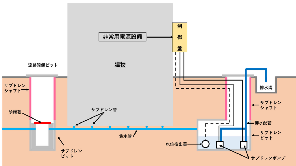
第4.1-1図 地下水排水設備の設備概要（エリア1, 2, 3, 4, 5, 6, 8, 11）
