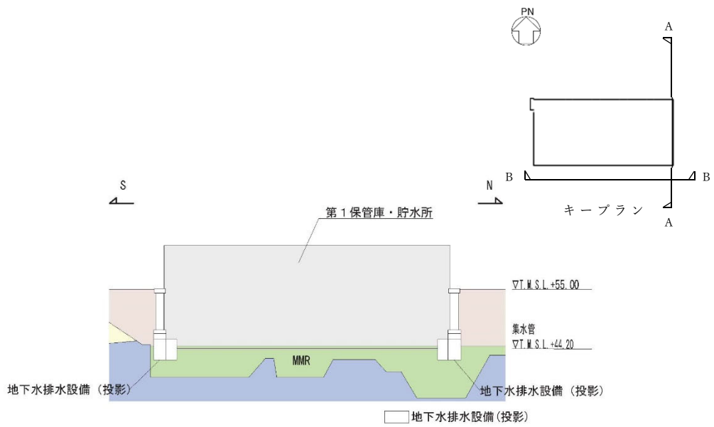
A - A 立面図
