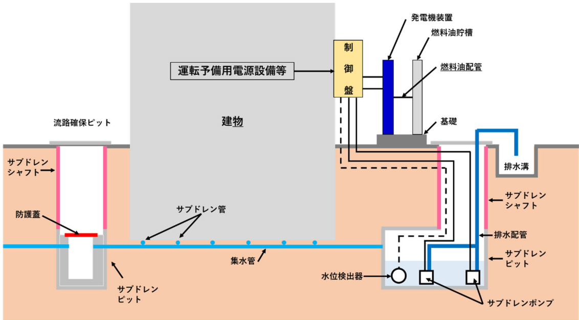
第 4.1-2 図 地下水排水設備の設備概要 (エリア 7, 9, 10)
