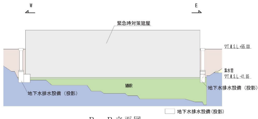
B - B 立面図
