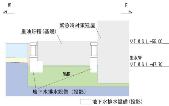
B - B 立面図
