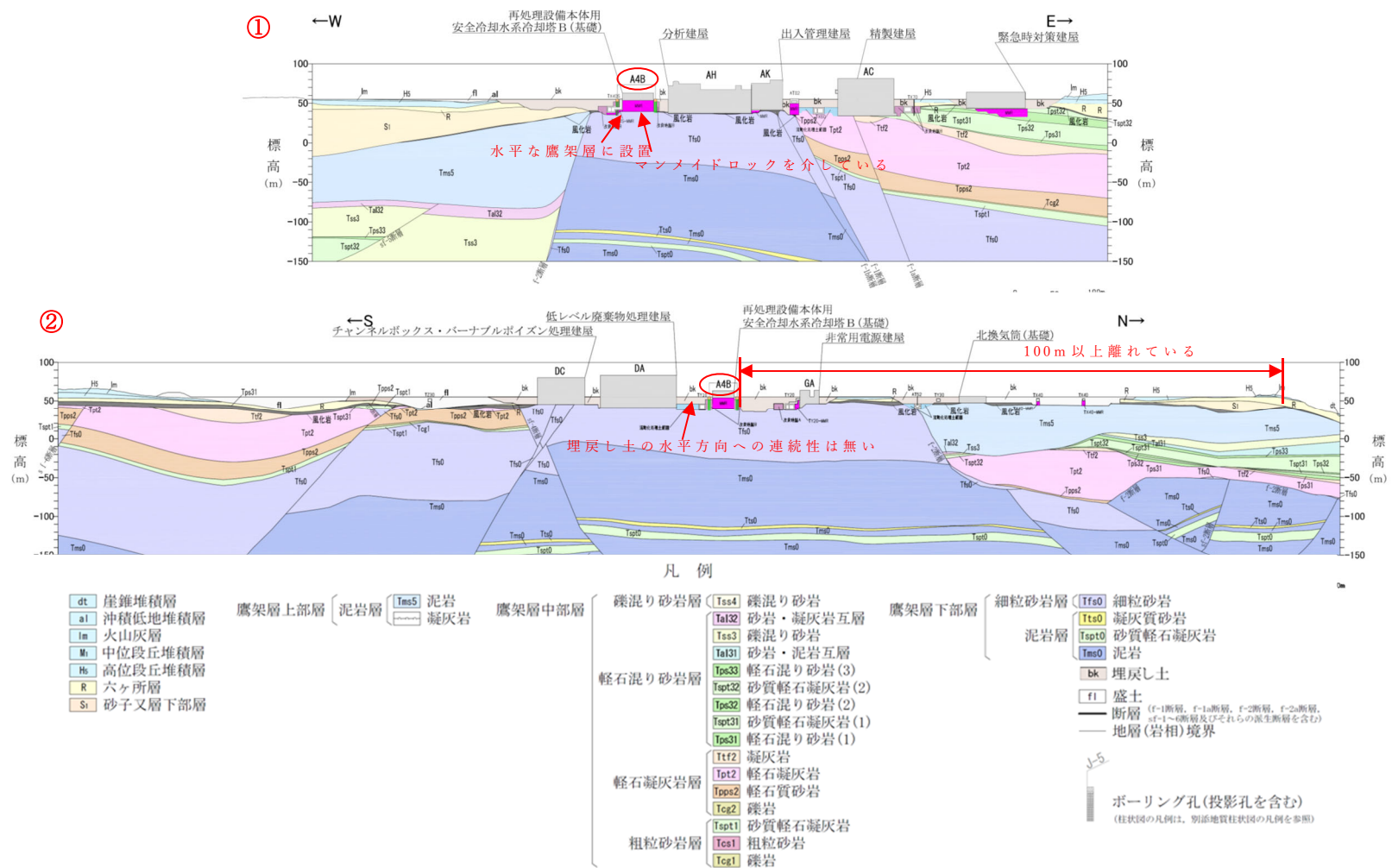
第 5.2.1-3 図 液状化影響評価対象施設の断面図
