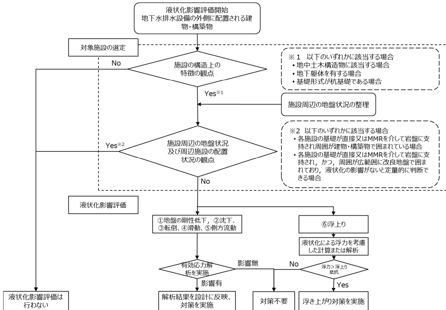
第 5.1-2 図 液状化影響評価対象施設の影響評価フロー
