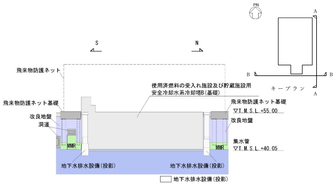
A - A 立面図
