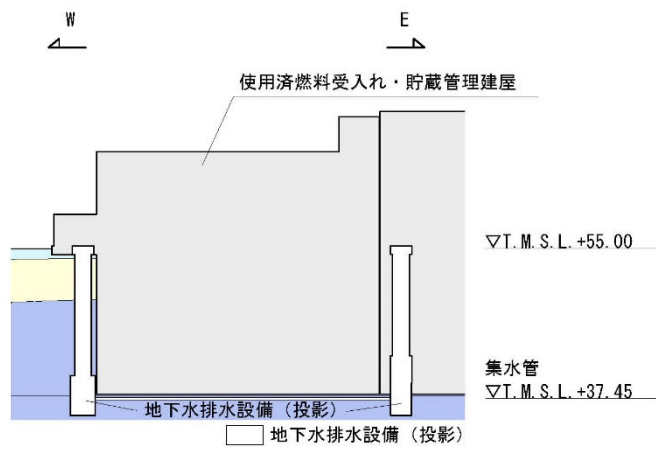
B - B 立面図
