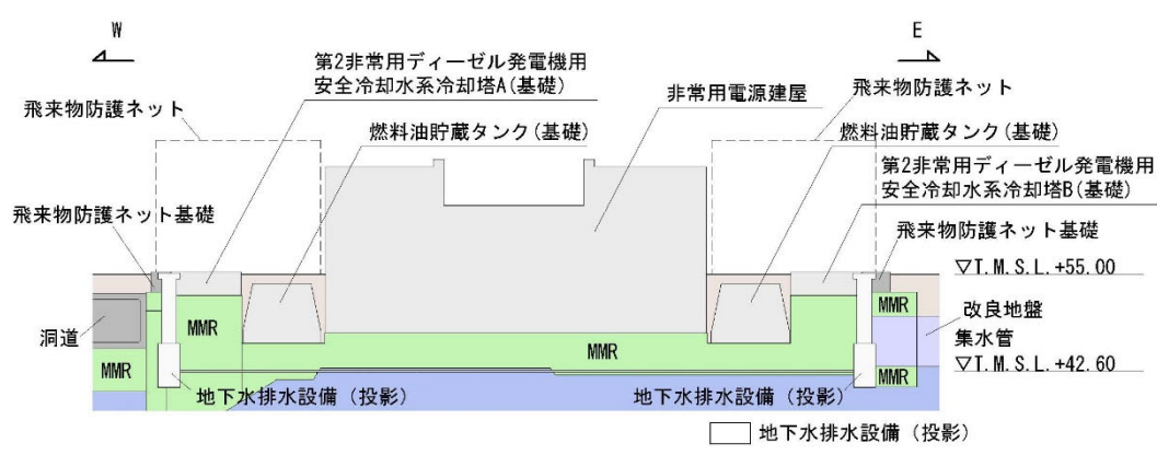
B - B 立面図
