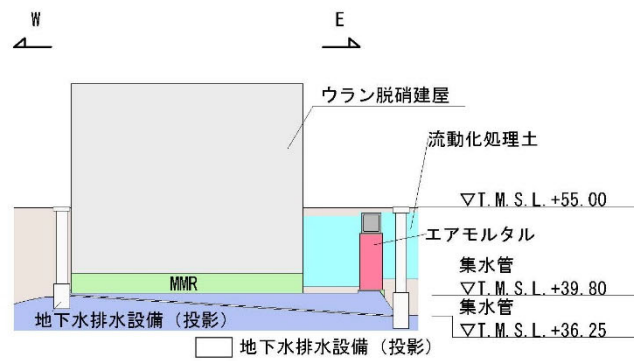
B - B 立面図
