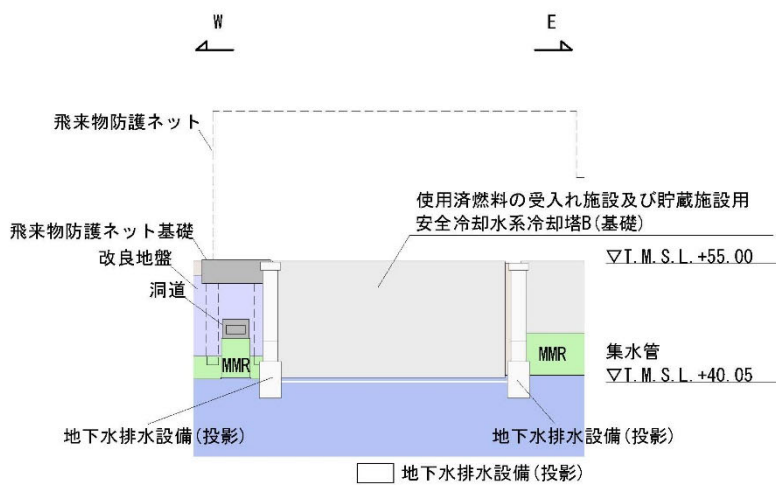
B - B 立面図
