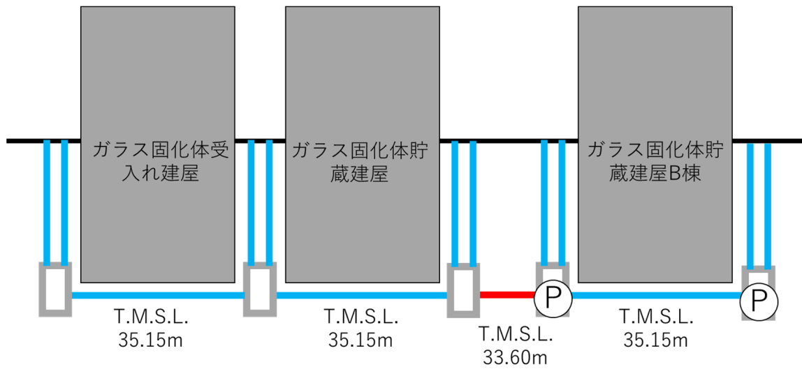
第 4.-2 図 集水エリア 10（ガラス固化体受入れ建屋，ガラス固化体貯蔵建屋，ガラス固化体貯蔵建屋 B 棟）の各建物・構築物の集水管レベル
