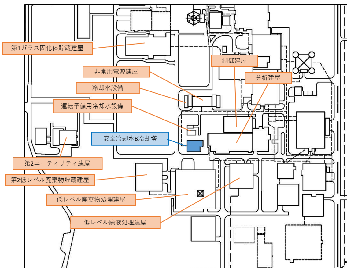
第2-6図 安全冷却水B冷却塔周辺の建屋配置状況
