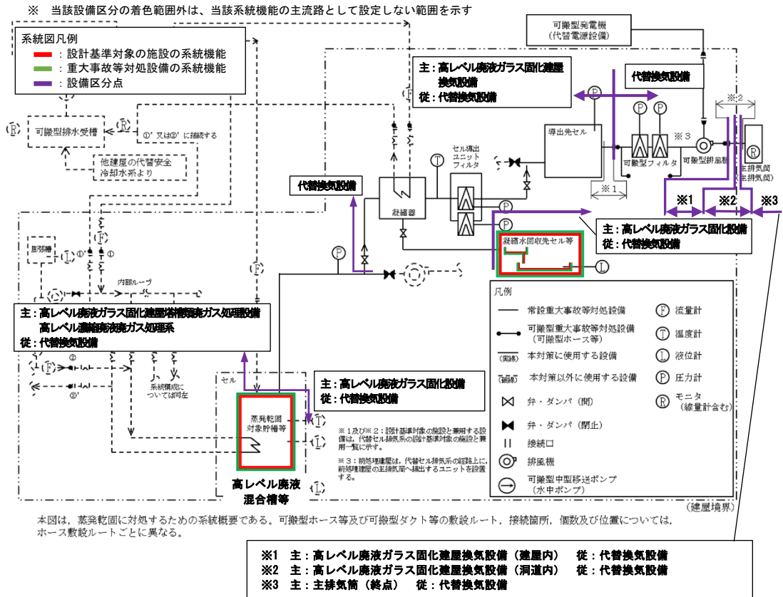
第2-14図 代替換気設備の系統概要図 (事業変更許可申請書 添付書類六 第7.2-38図(1)抜粋)
