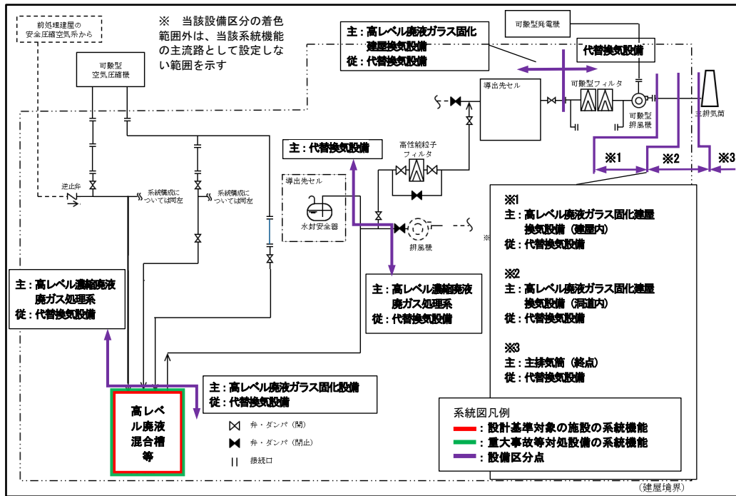
第 2 - 18 図 代替換気設備 系統概要図
