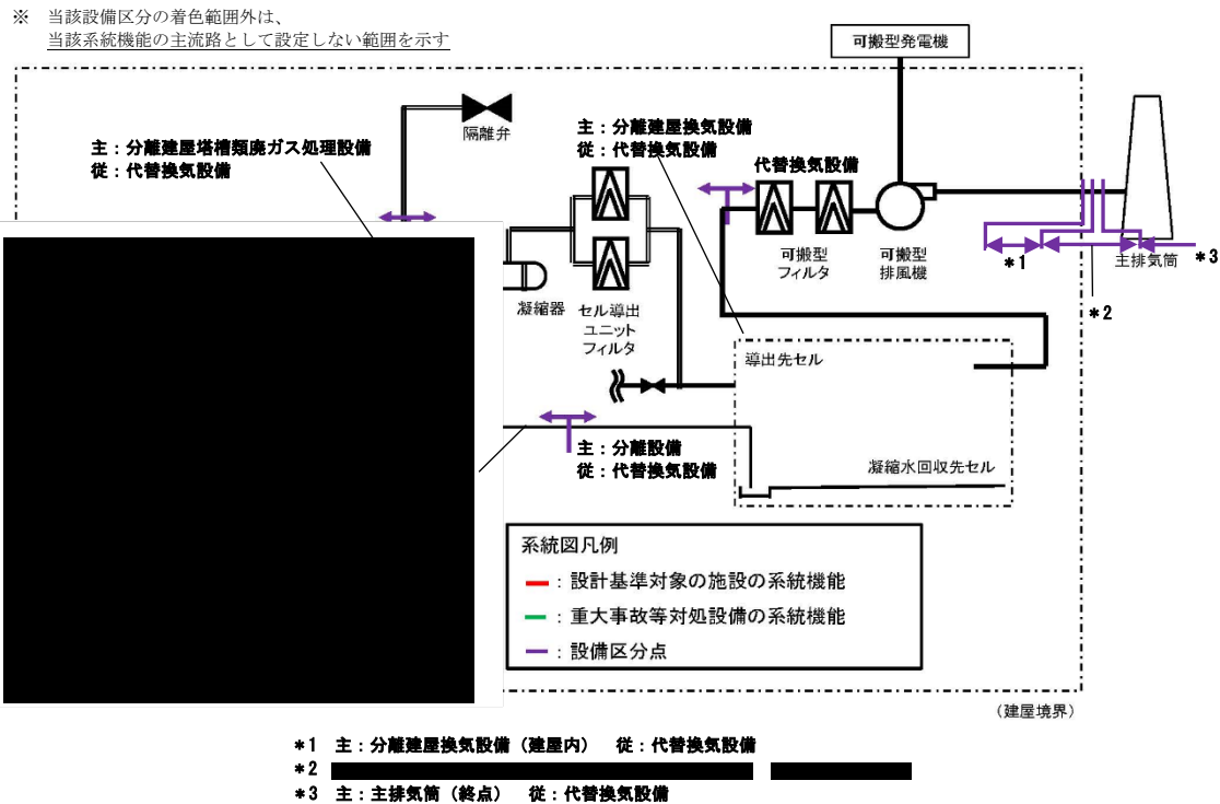
第2-15図 代替換気設備（セル導出設備） 系統概要図
