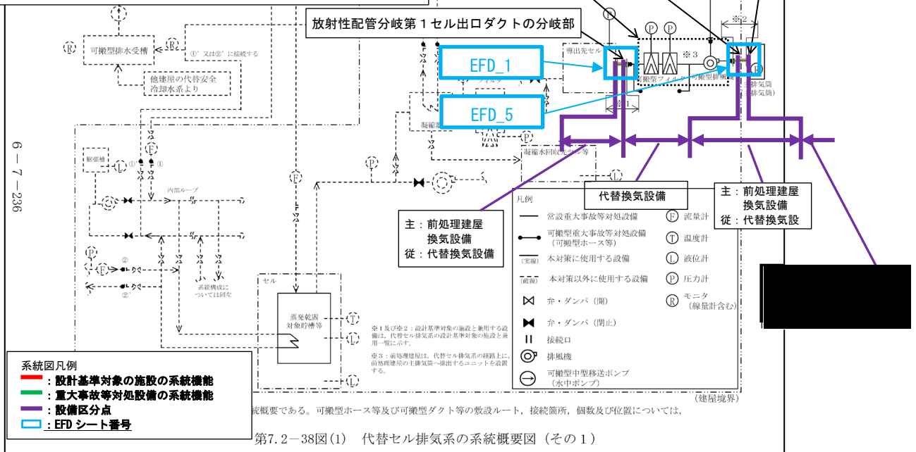
第3-2図 代替換気設備の系統概要図
