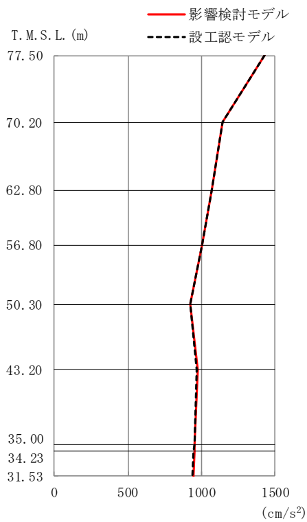
第 3.2-1 図 最大応答加速度 (NS 方向)
