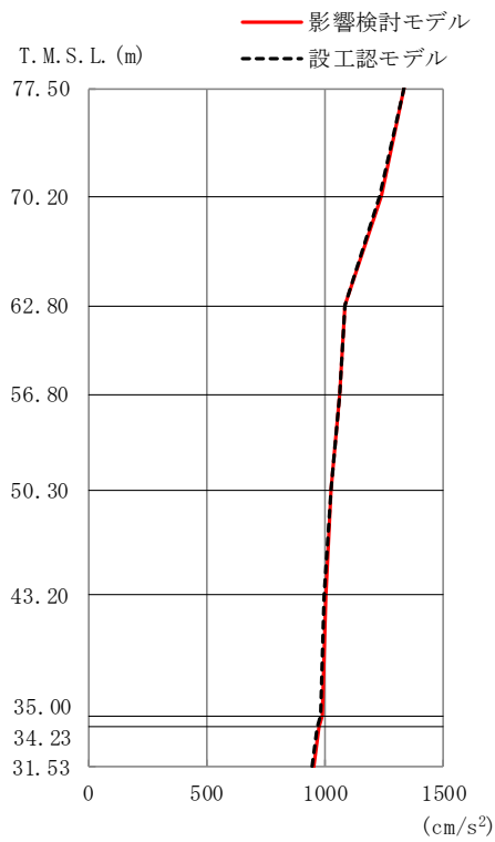
第 3.2-4 図 最大応答加速度 (EW 方向)
