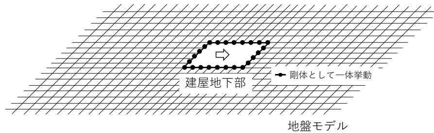
第 4.1-1 図 有限要素法の概念図
