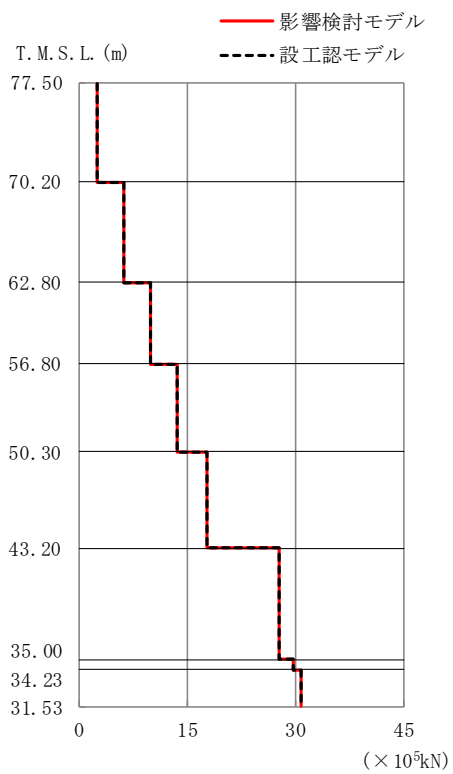
第 3.2-2 図 最大応答せん断力 (NS 方向)
