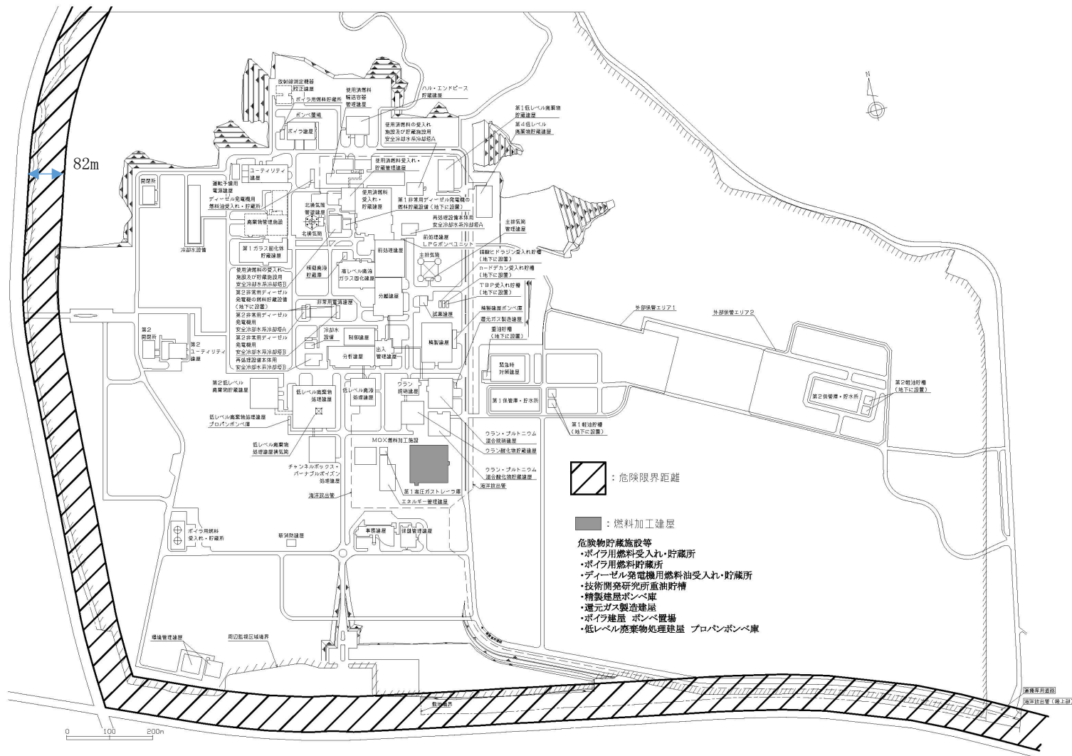
第 3-2 図 公道と燃料加工建屋の位置関係
